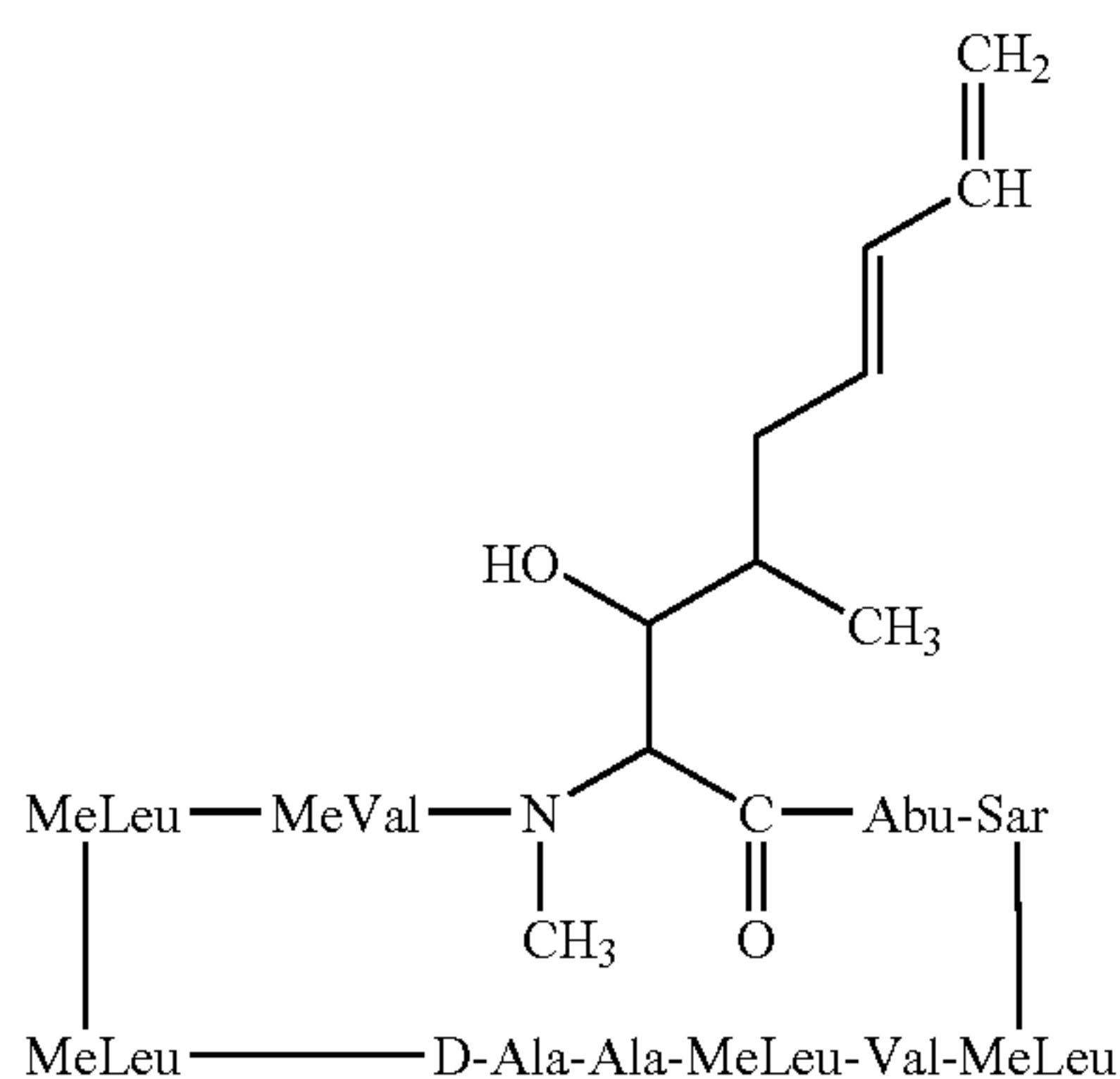
E-isomer
