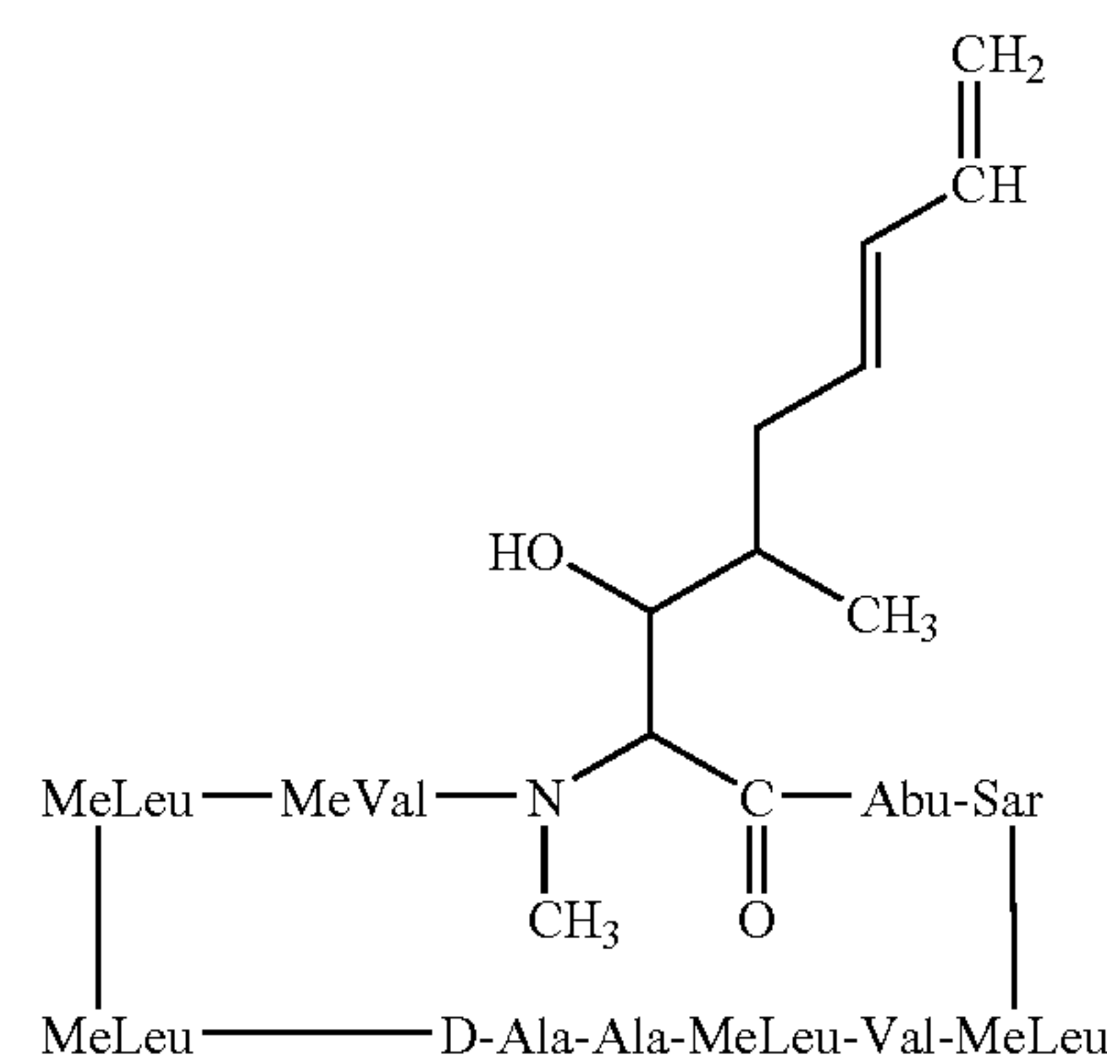
E-isomer
