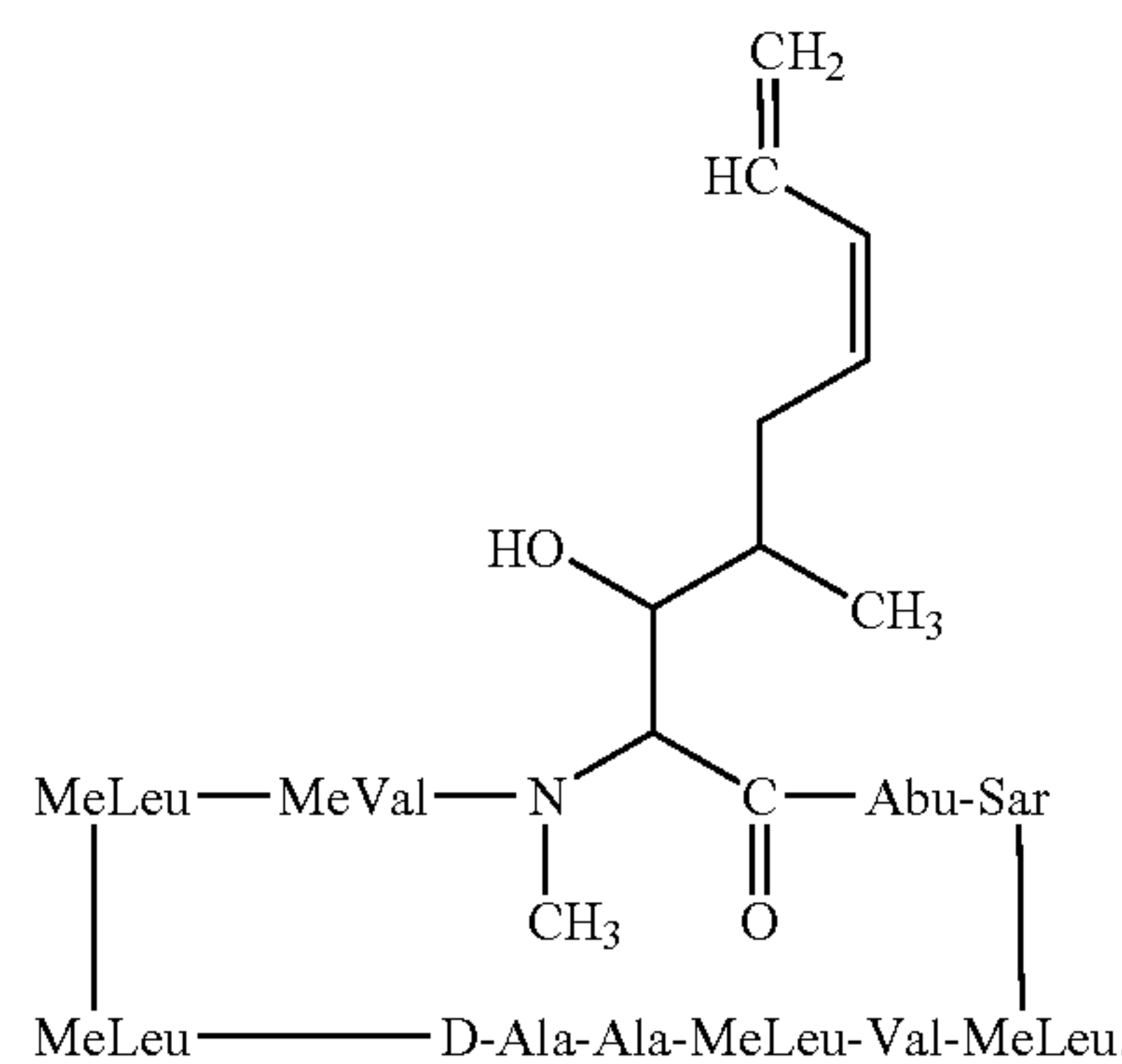
E-isomer
