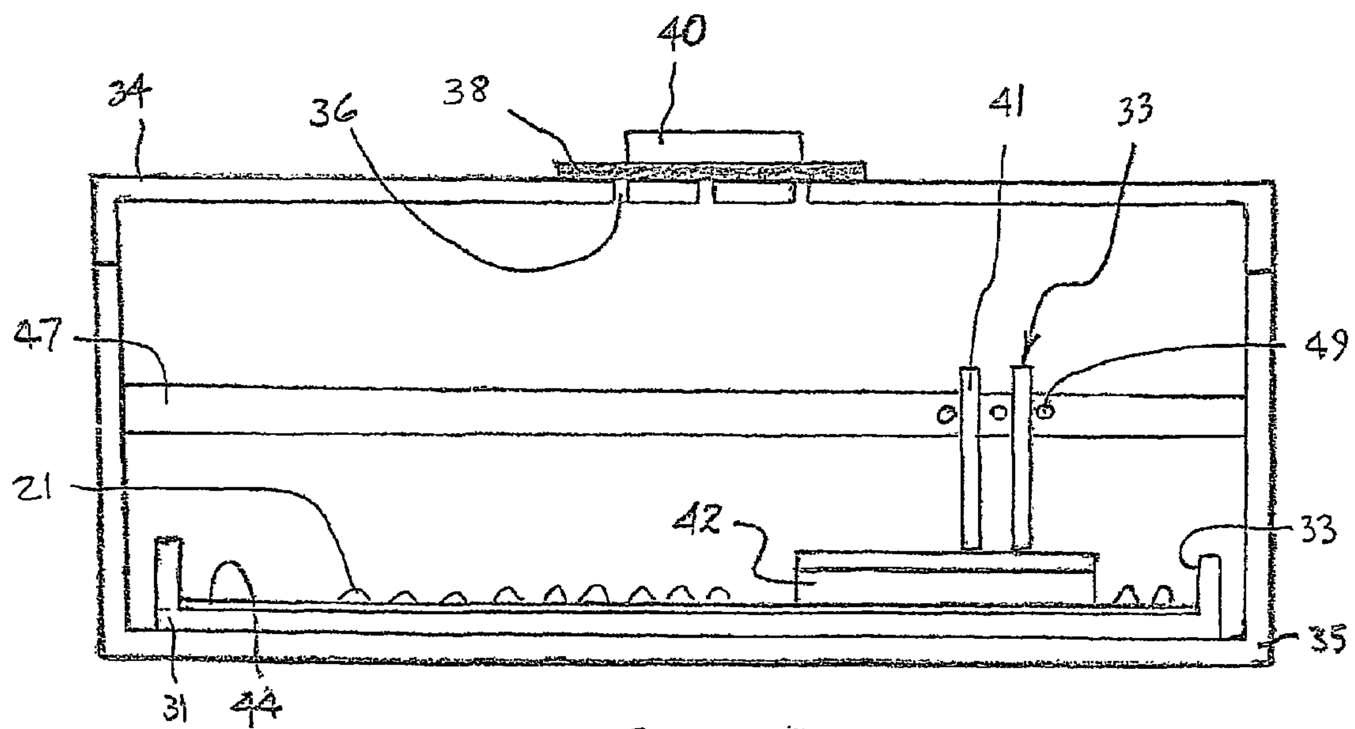
FIG. 2B
