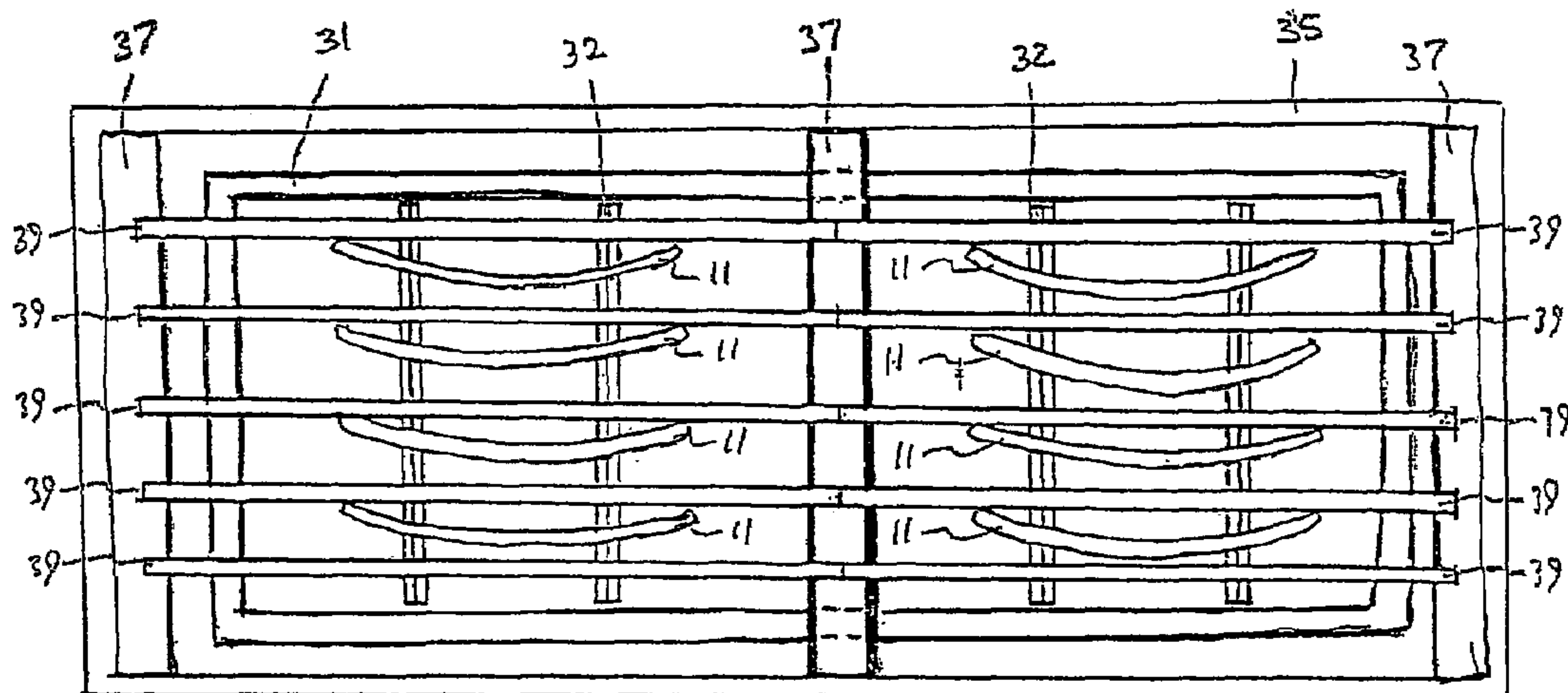
FIG. 4A
