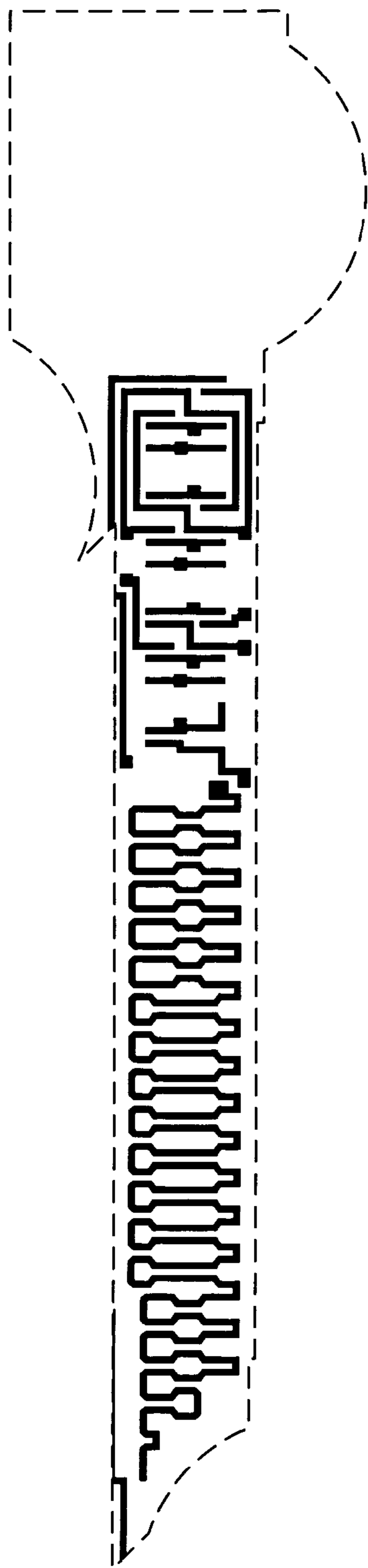
Poly mask
