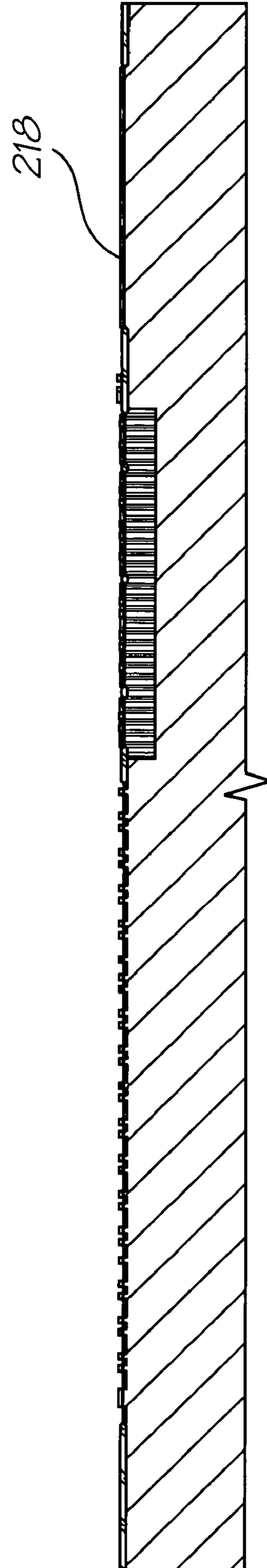
p+ implant
