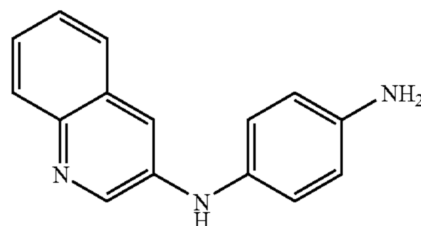
N-Quinol-3-yl)-benzene-1,4-diamine
