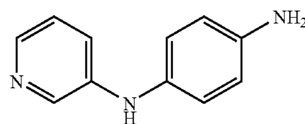
N-Pyrid-3-yl)-benzene-1,4-diamine
