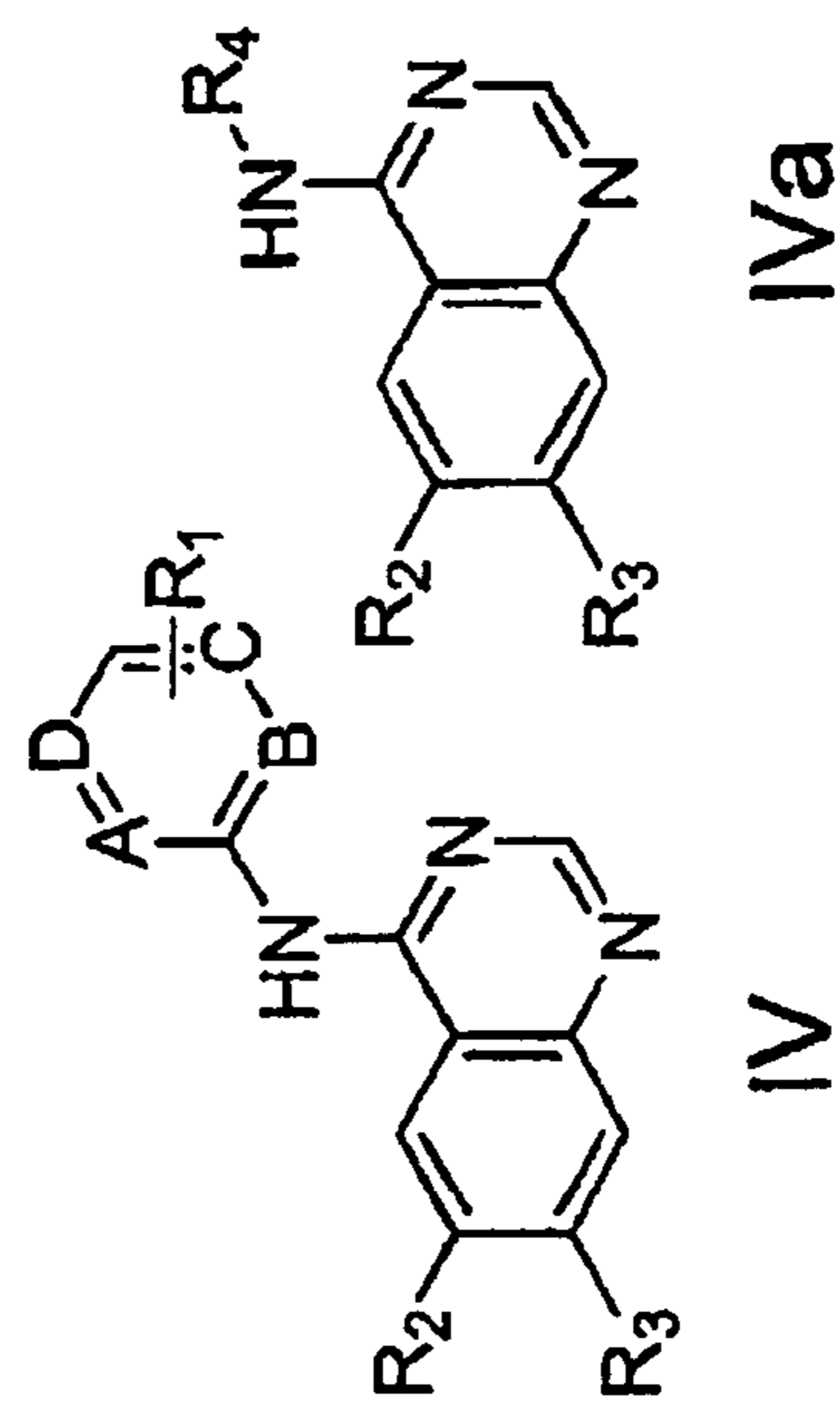
Quinazolines
