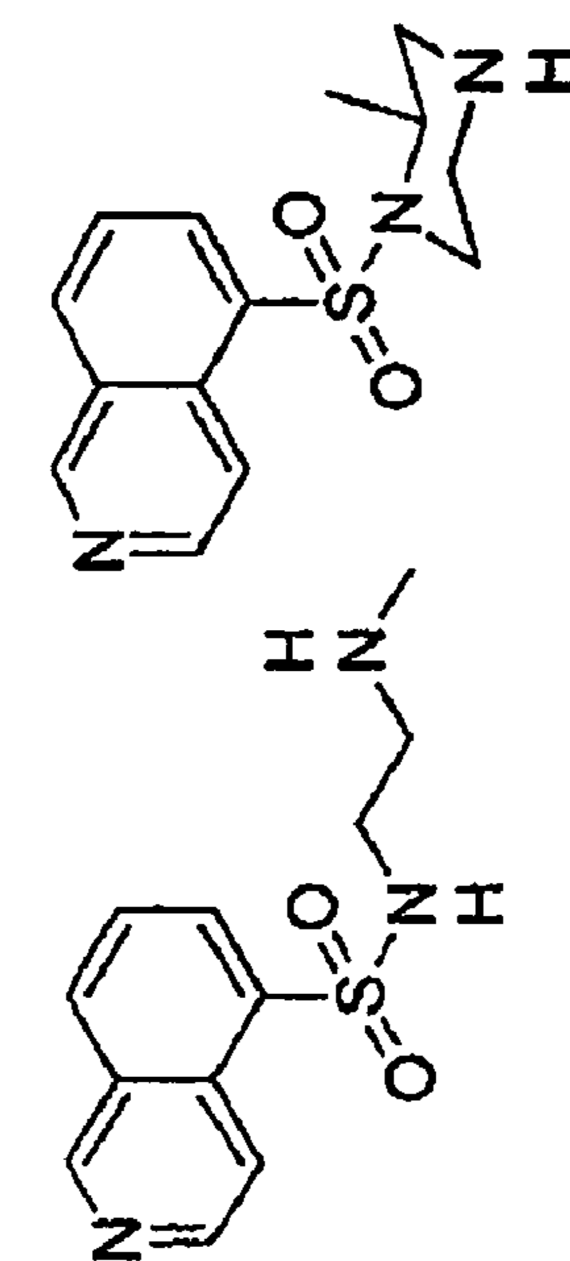
H-8
