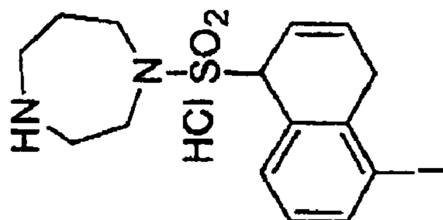
ML-7
