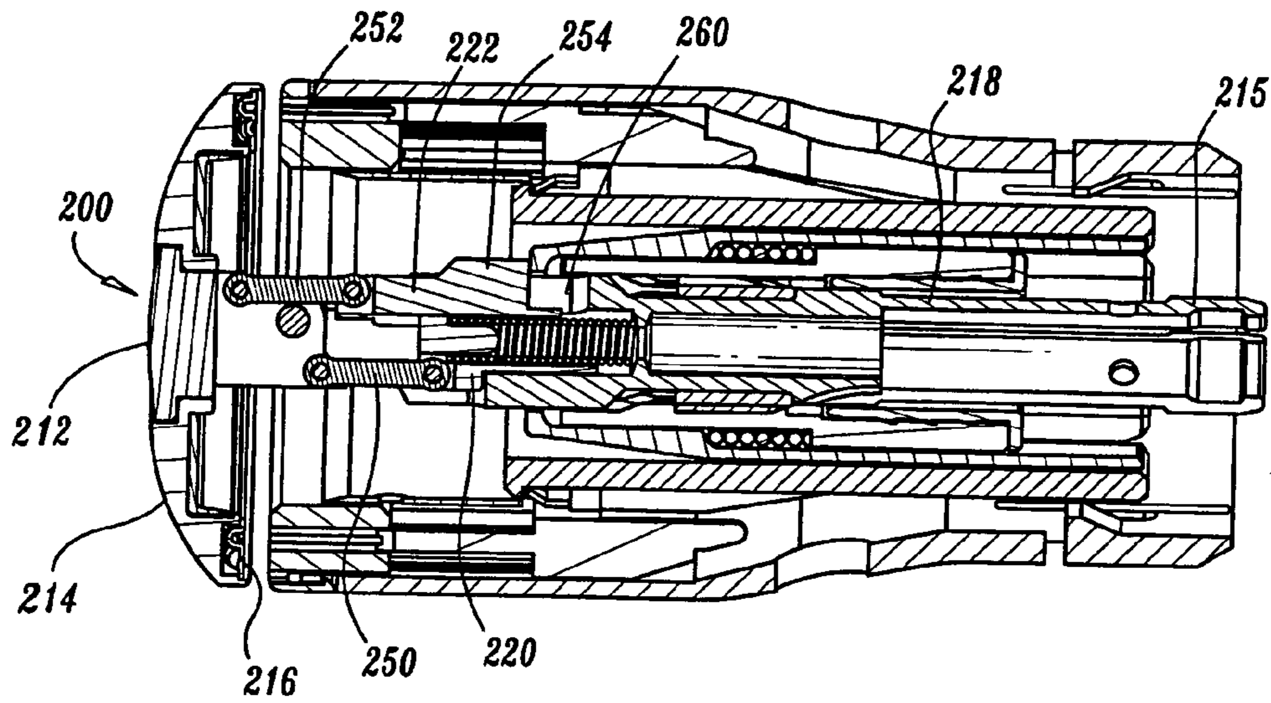
FIG. 12
