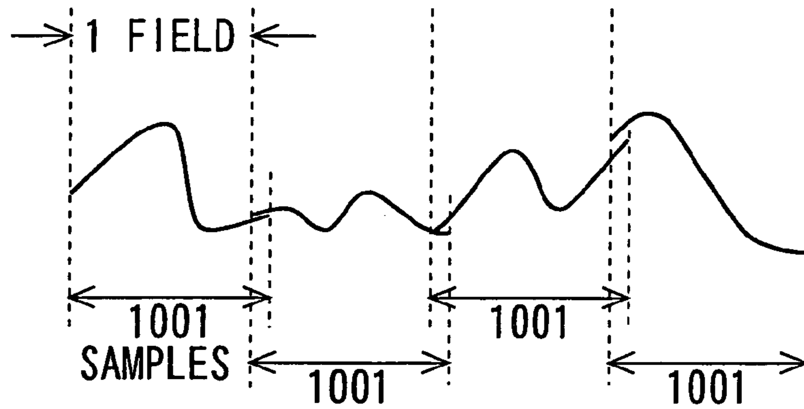
FIG. 2B (25Hz)
