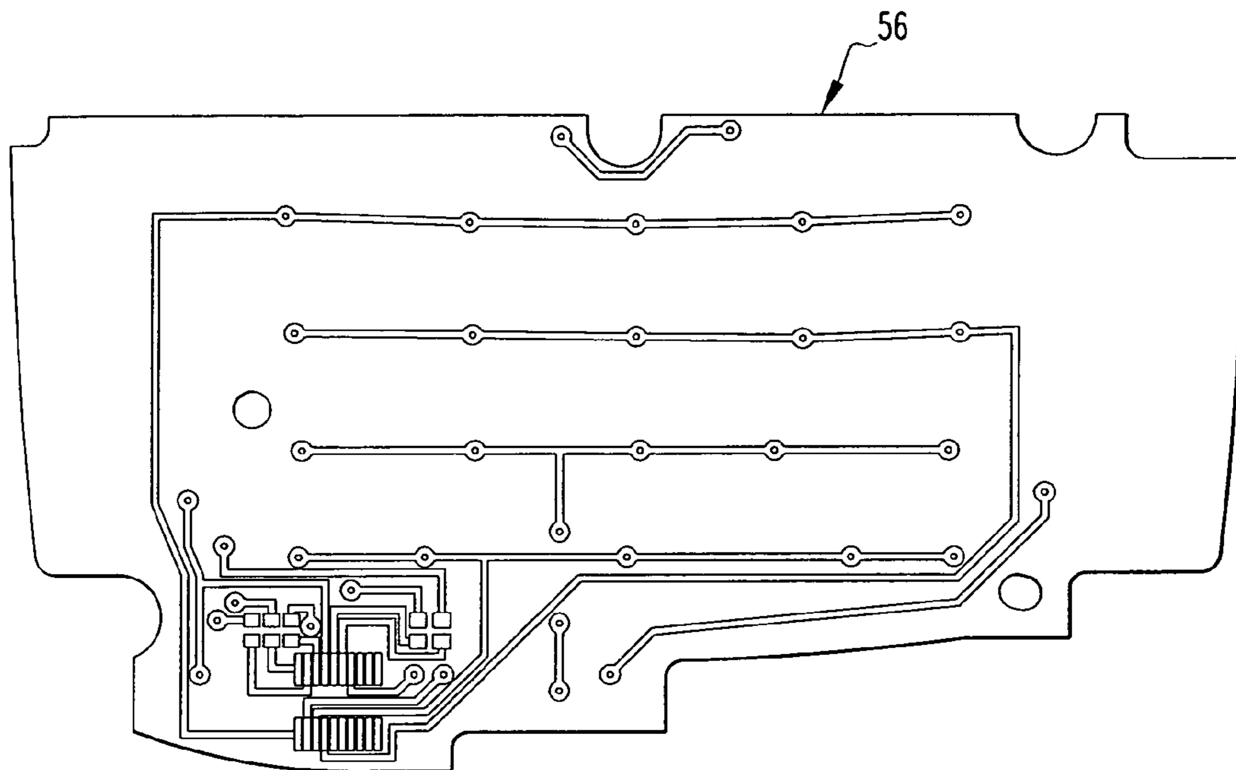
FIG. 7A
