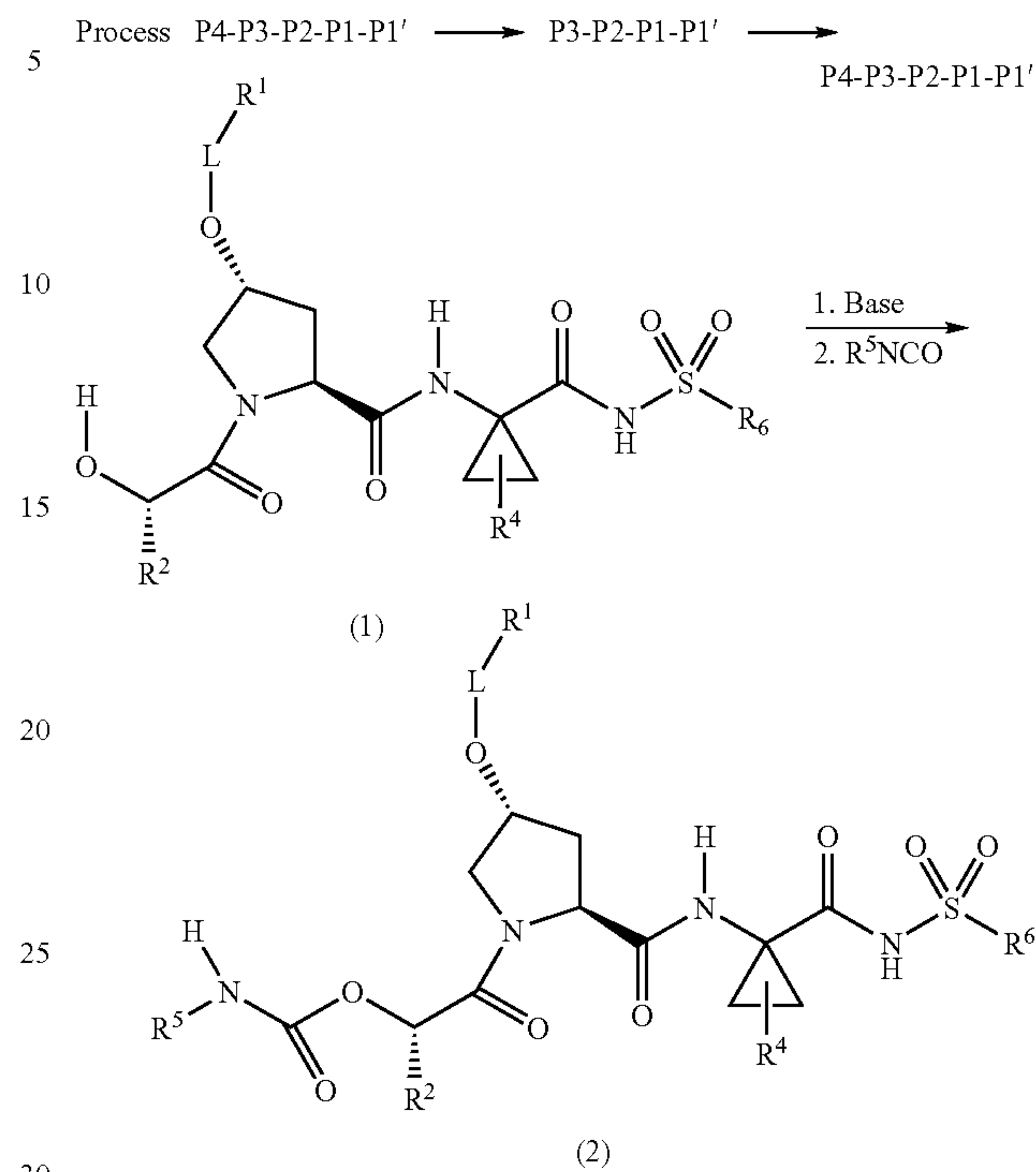
Scheme VI
