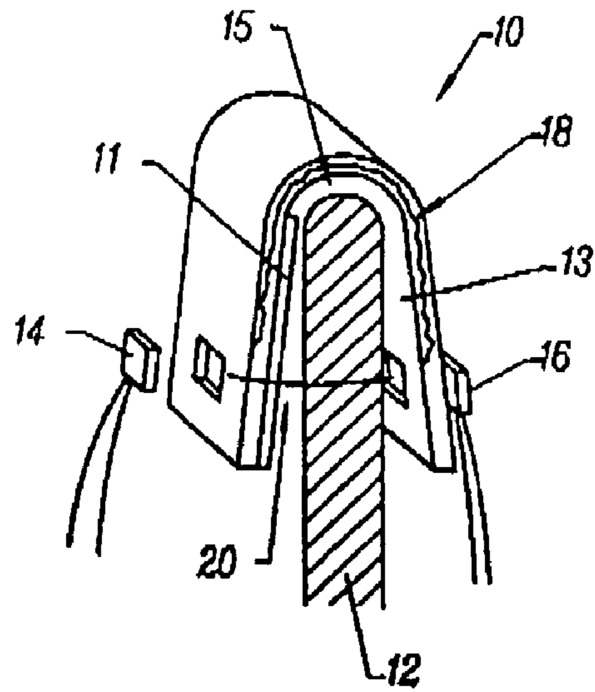
FIG. 1 PRIORART
