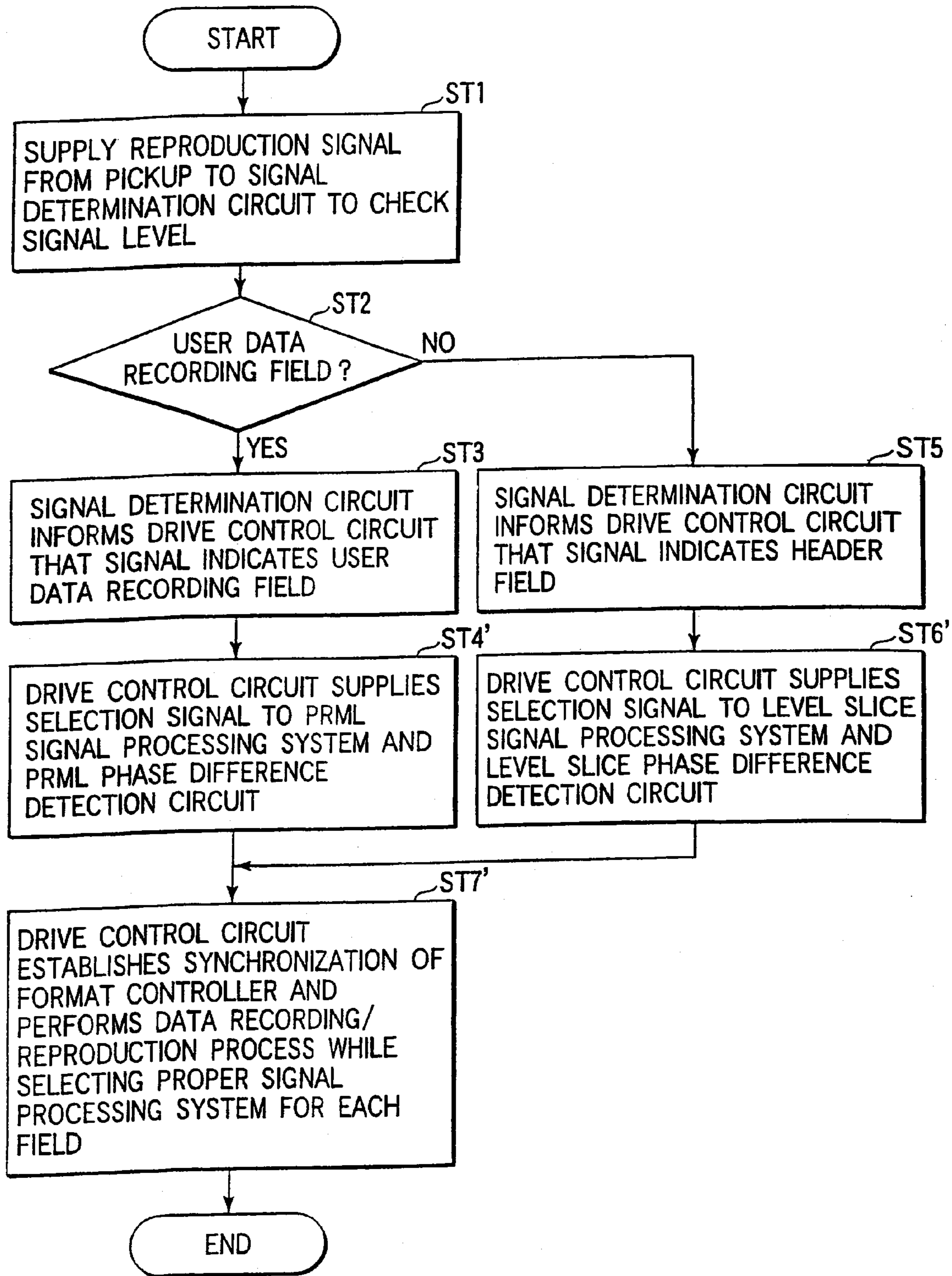
FIG. 28
