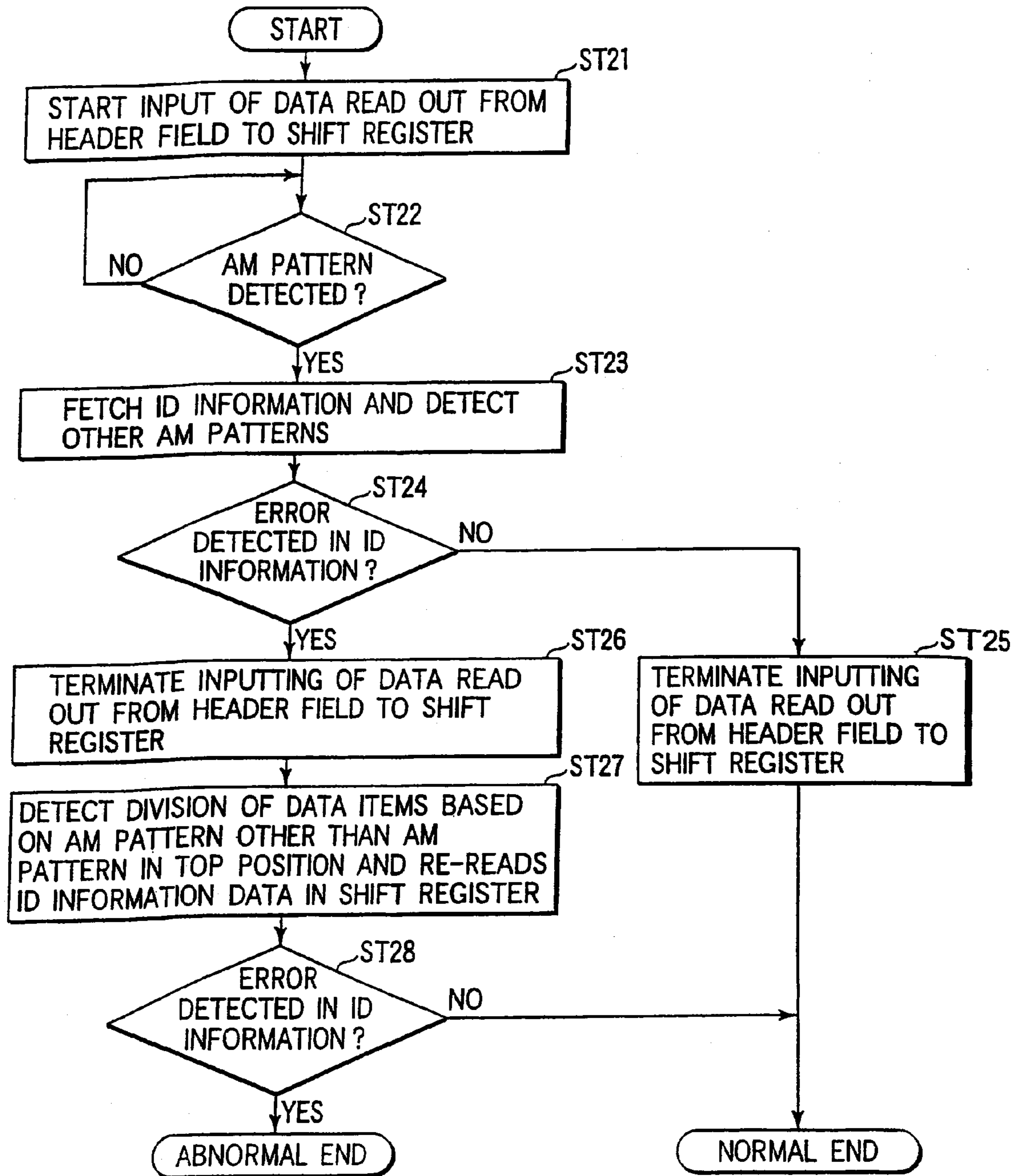
FIG. 32
