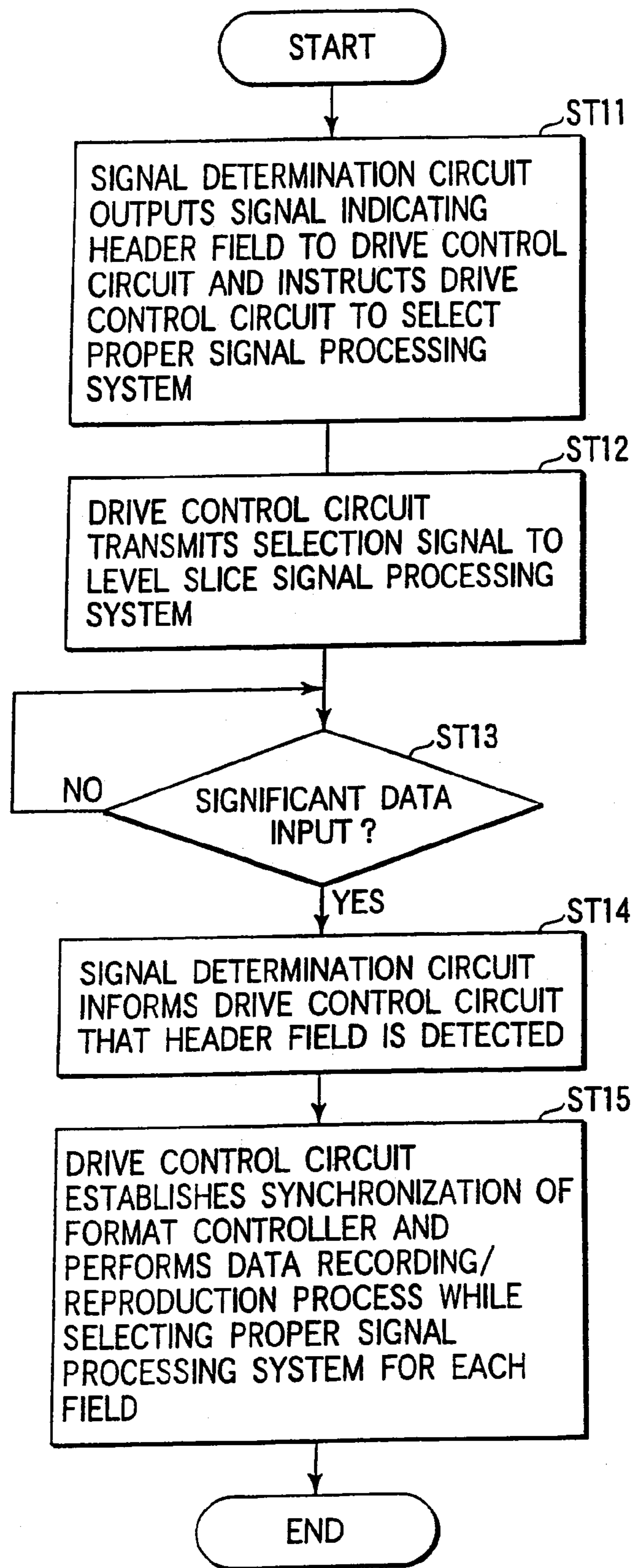
FIG. 25
