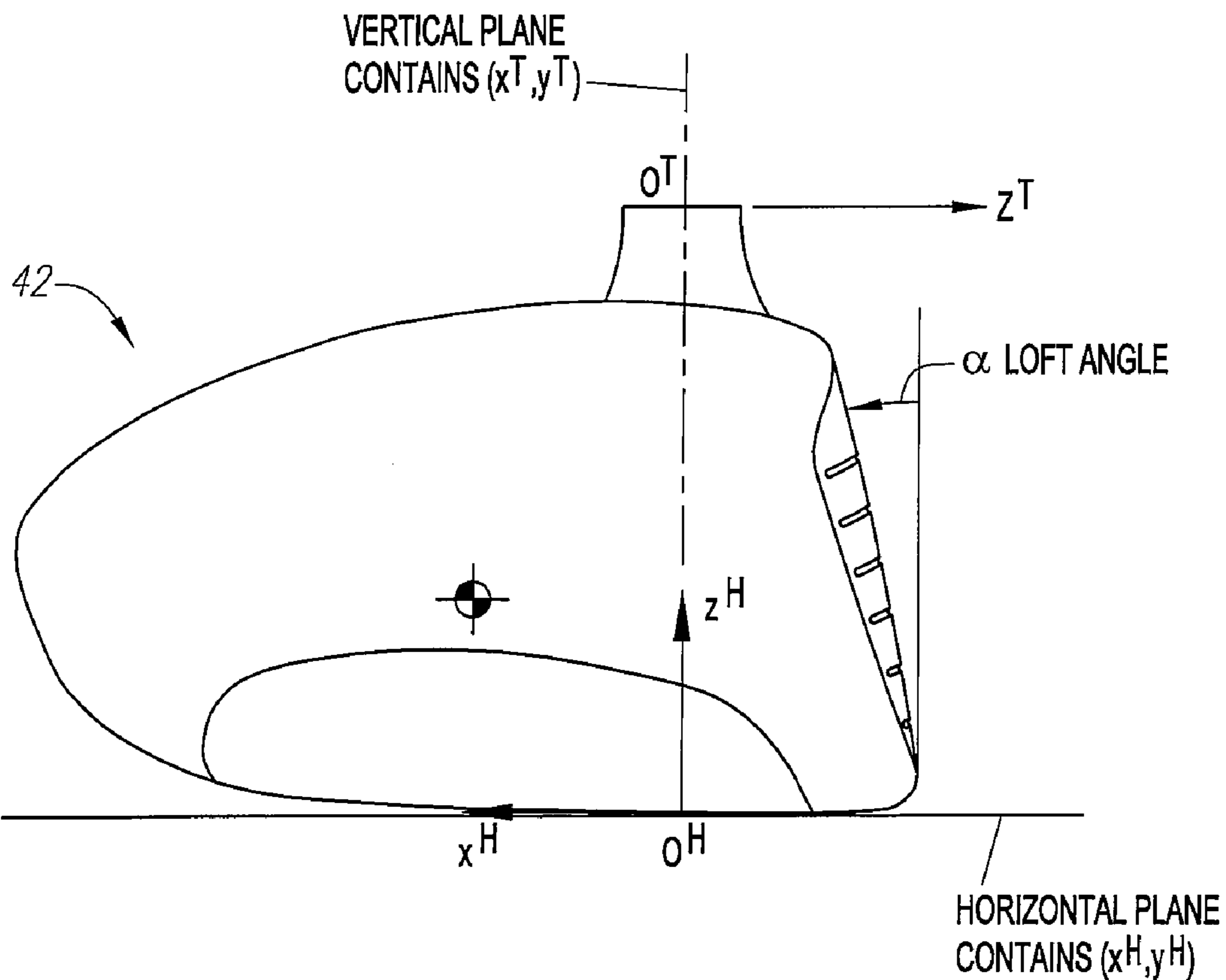
FIG. 11A
