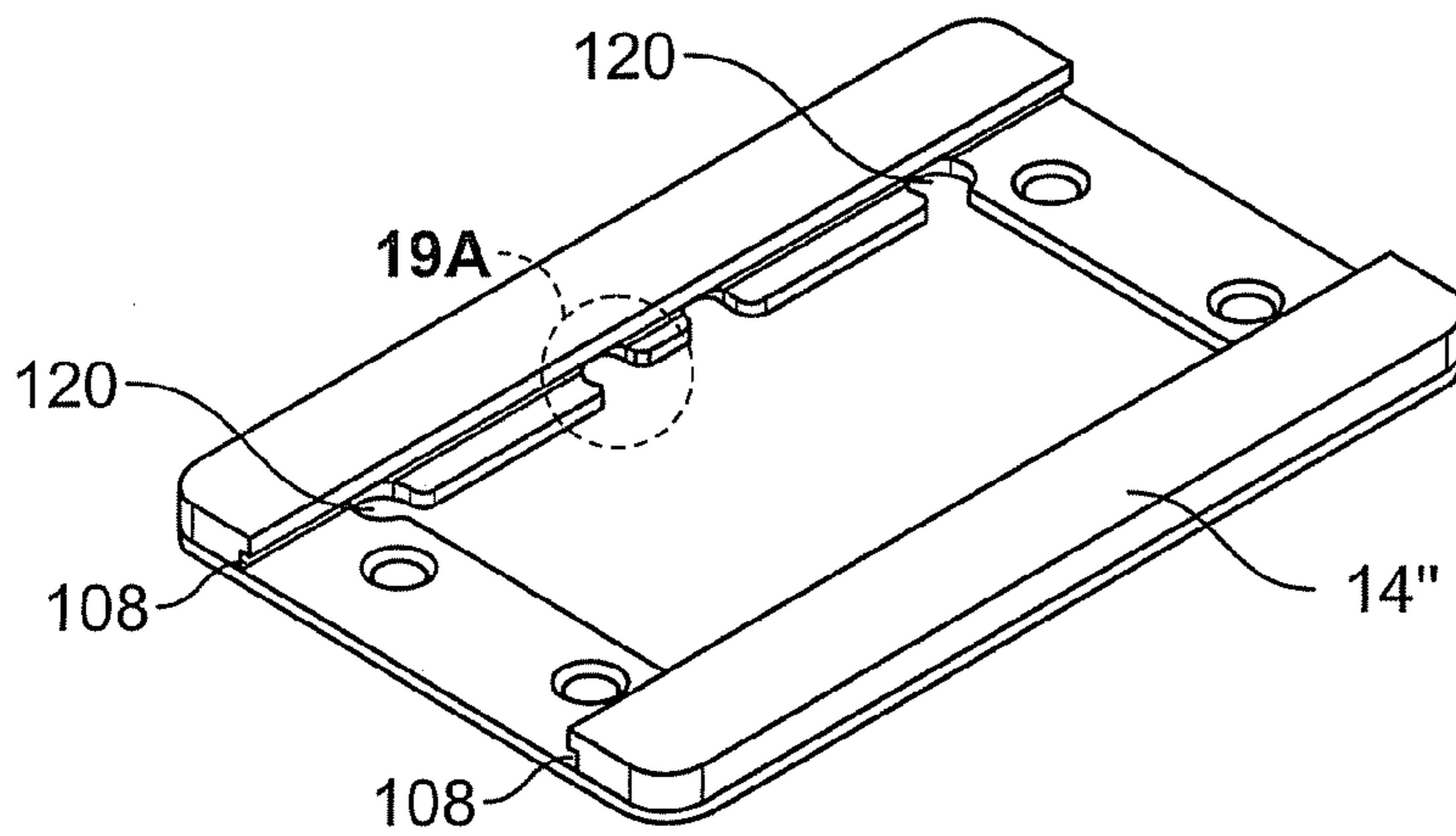
FIG. 19
