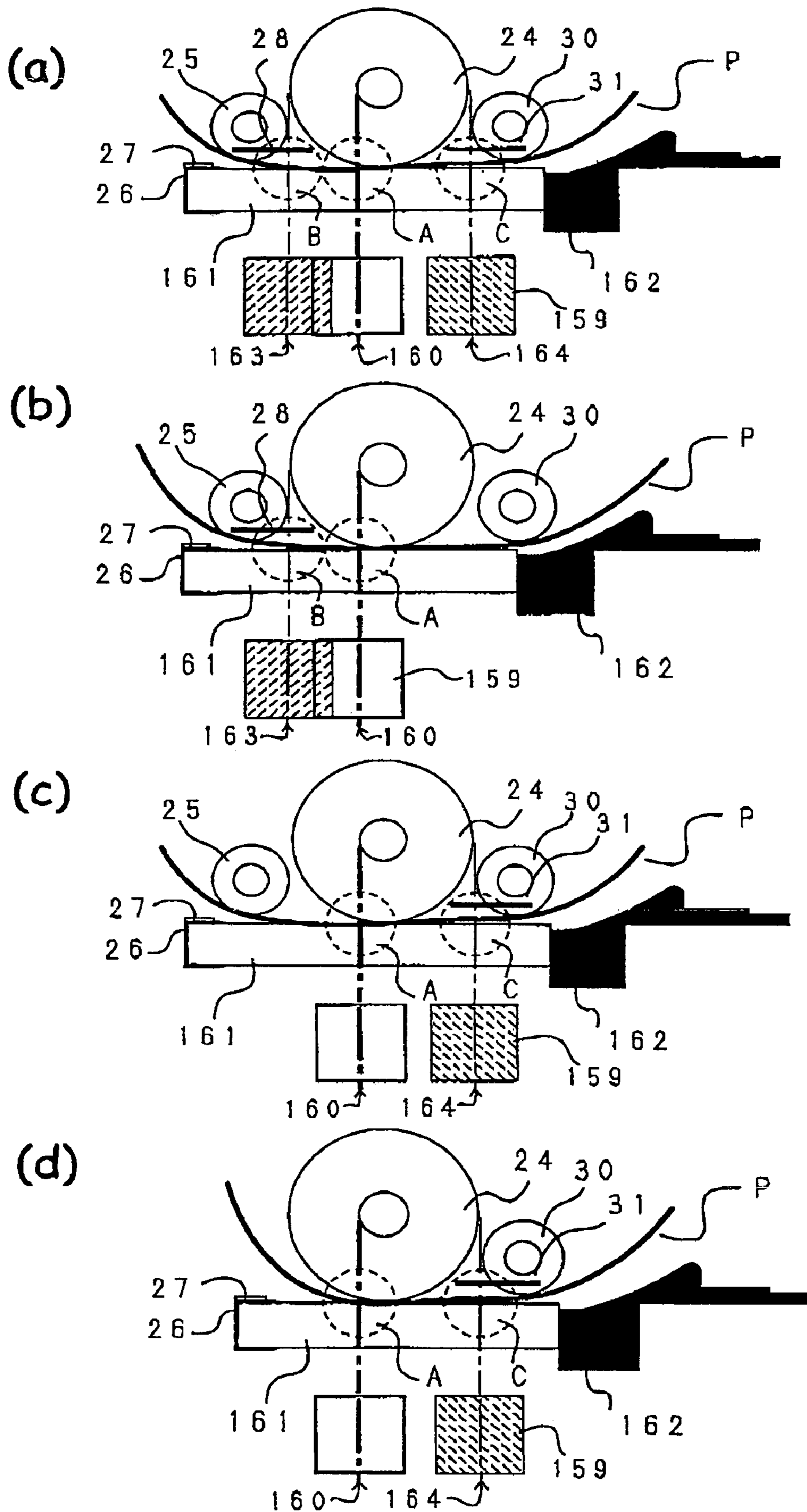
FIG. 9
