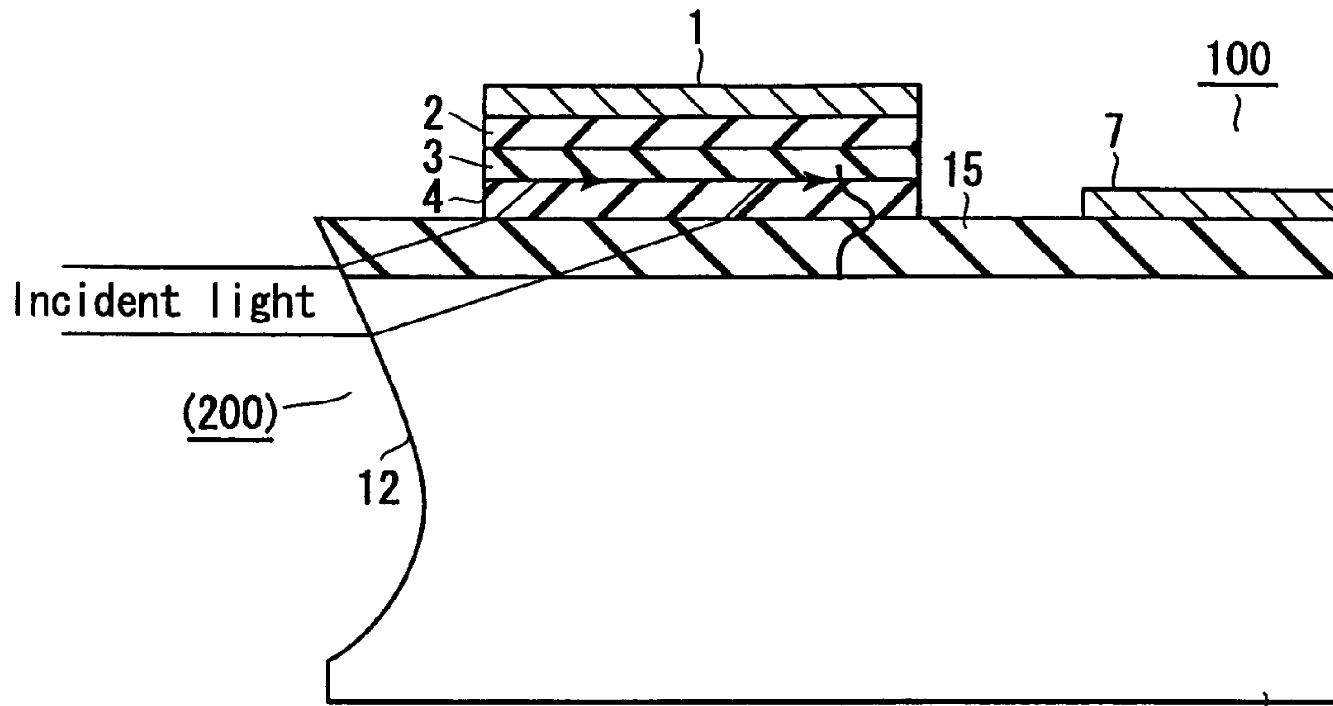
FIG. 32
