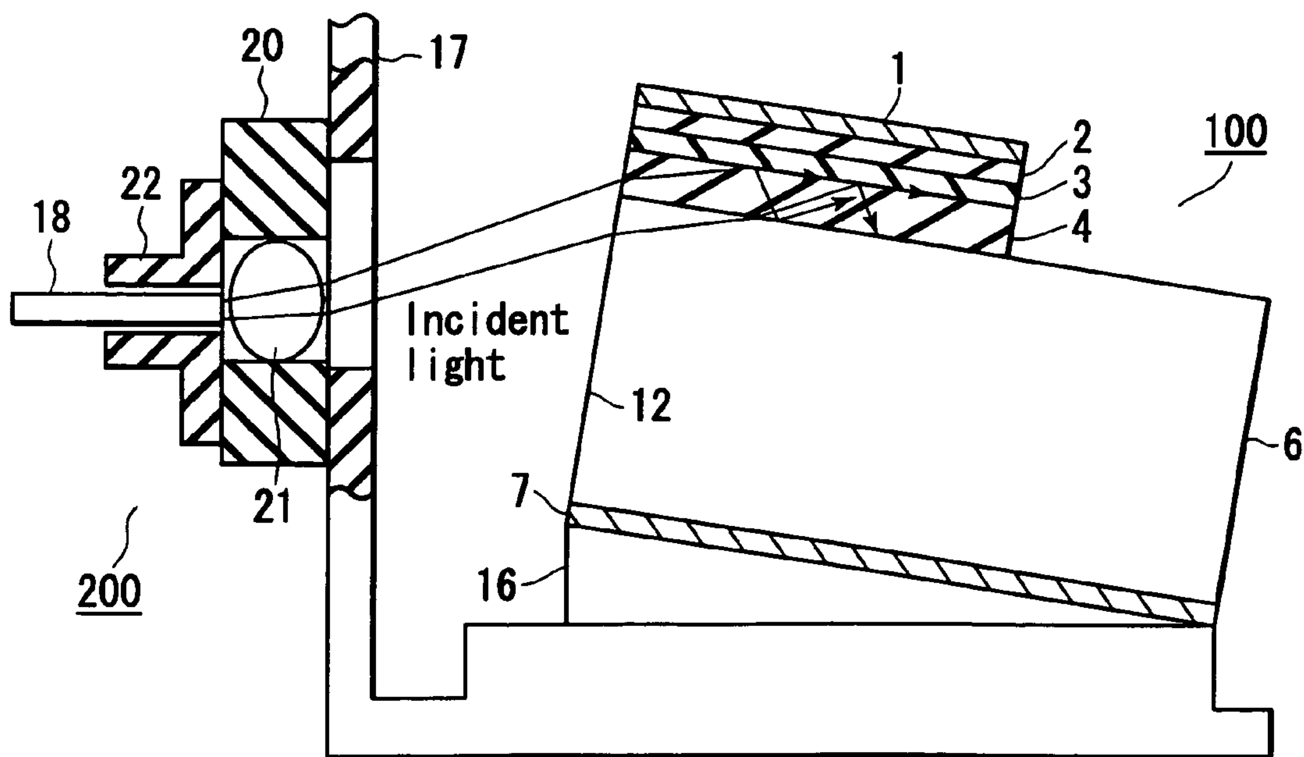
FIG. 11
