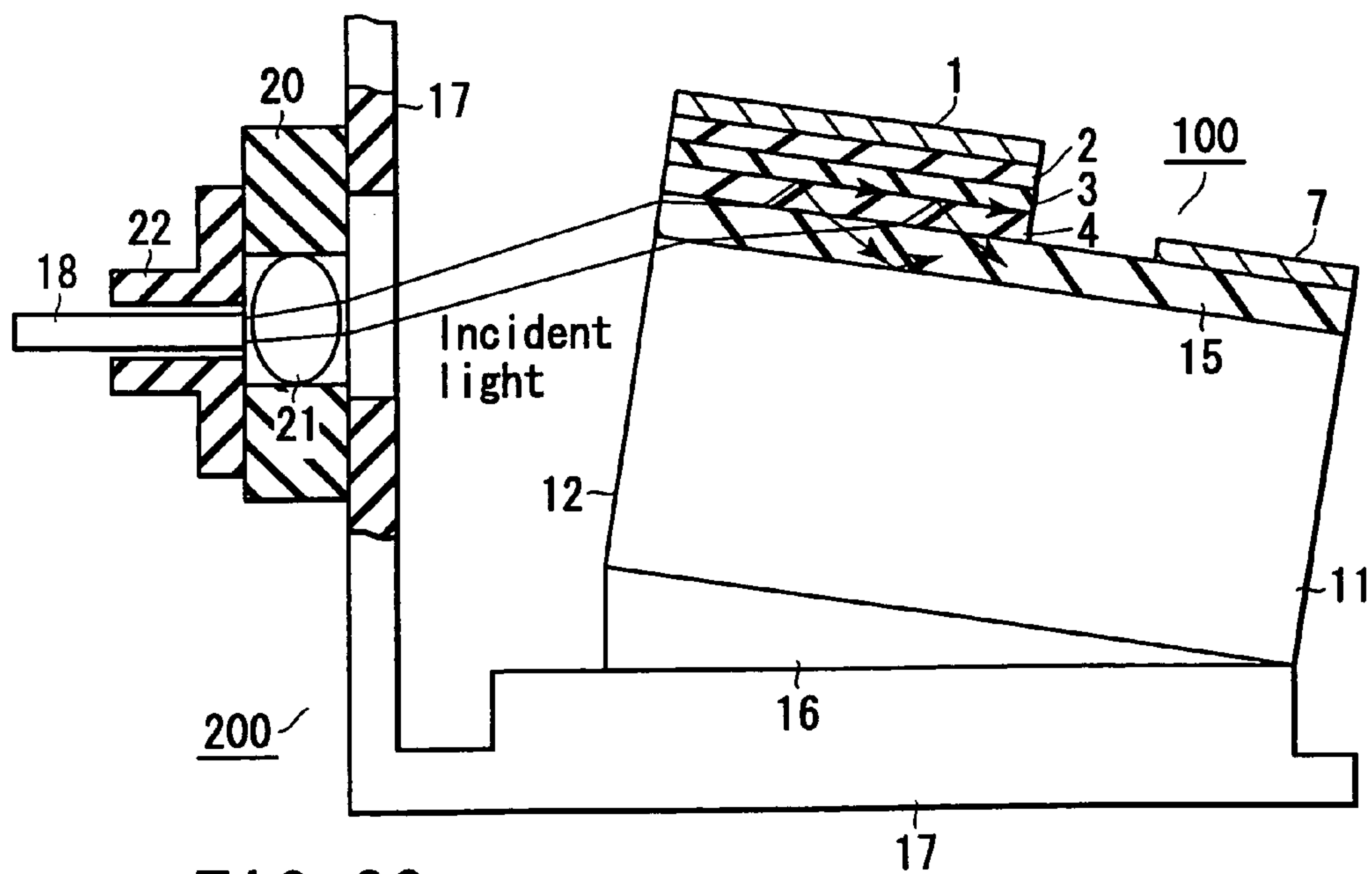
FIG. 22
