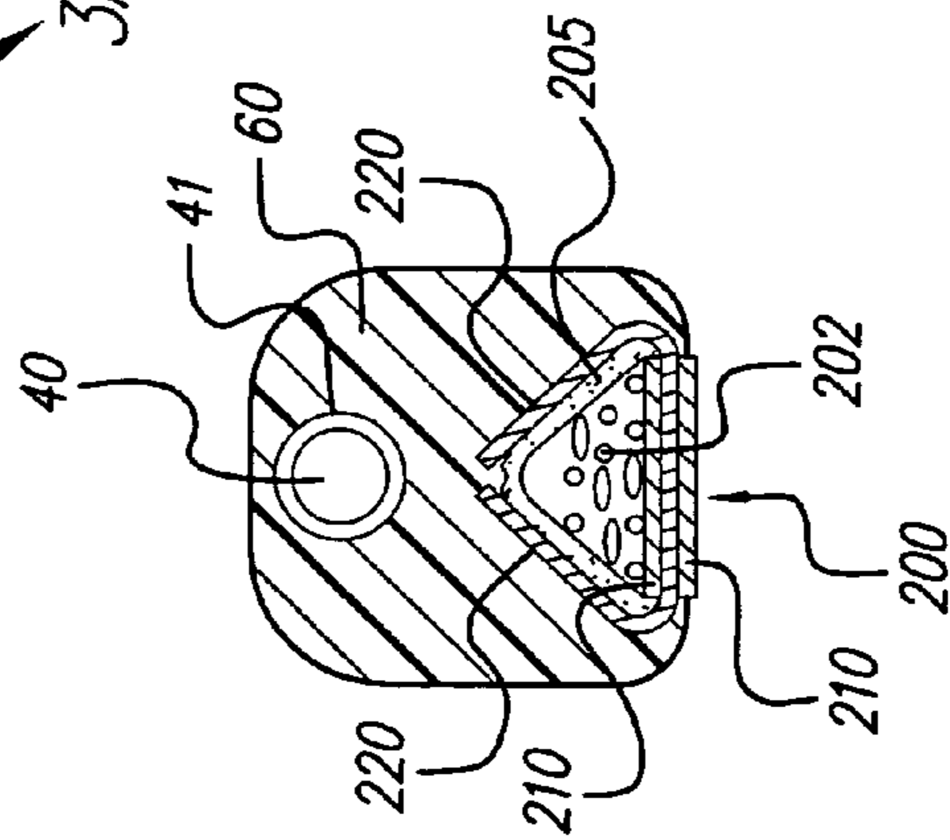
FIG. 3B
