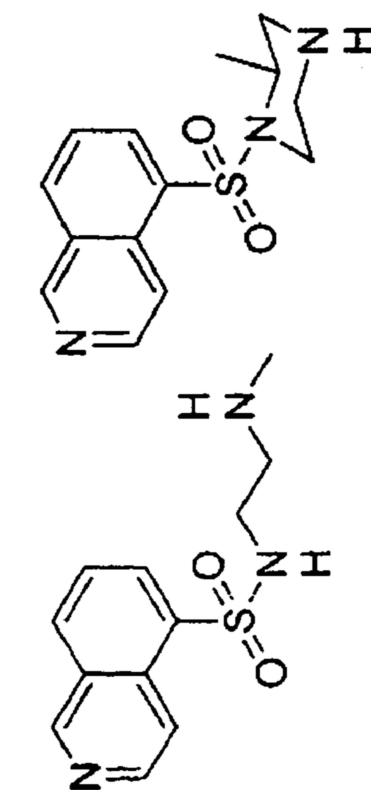
H-8
