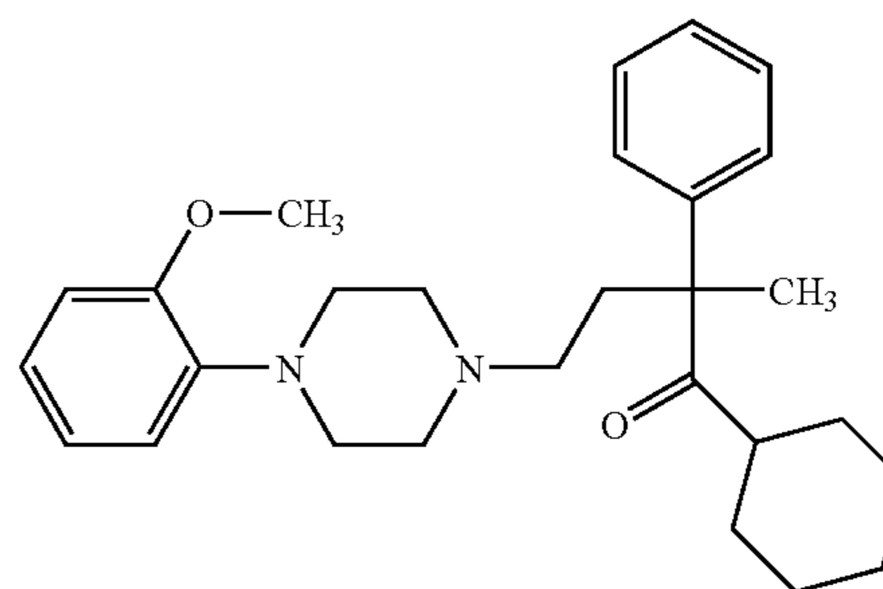
1-(2-methoxyphenyl)-4-[3-(cyclohexanecarbonyl)-3-(phenyl)butyl]piperazine
