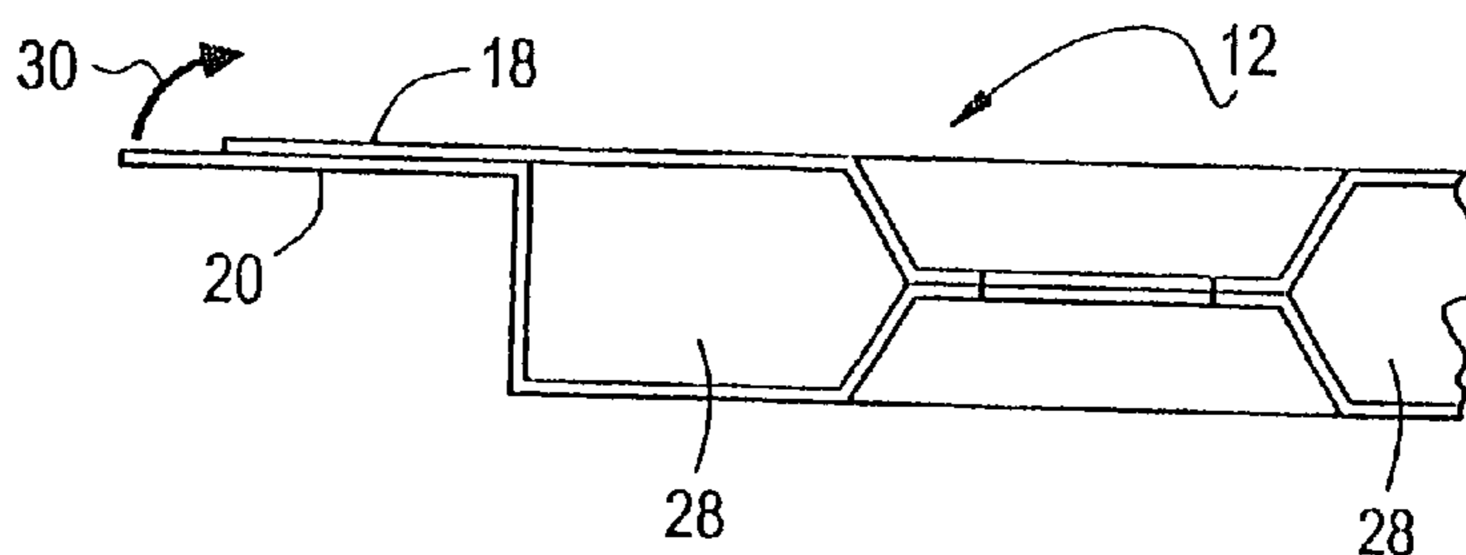
FIG. 4A
