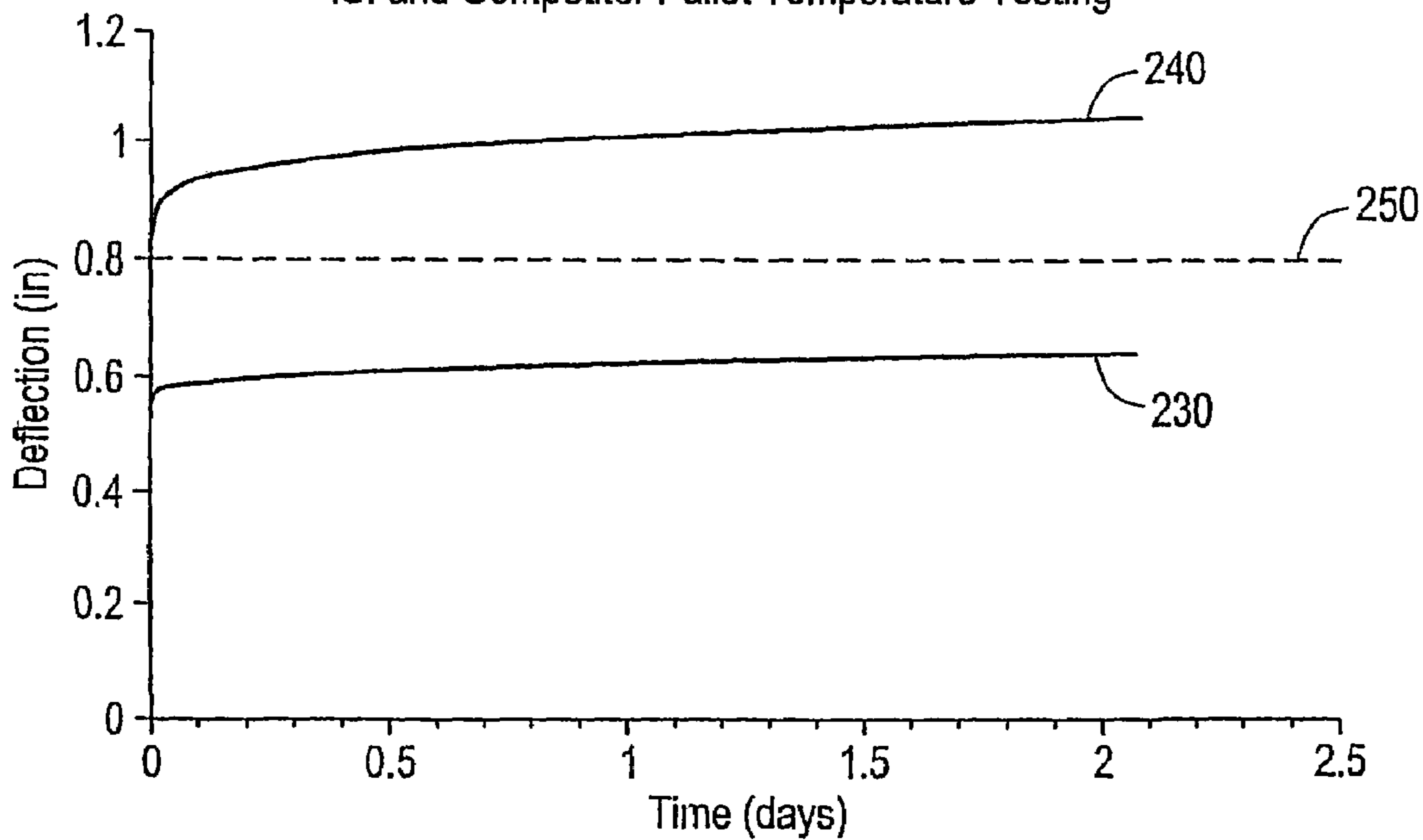
FIG. 29
