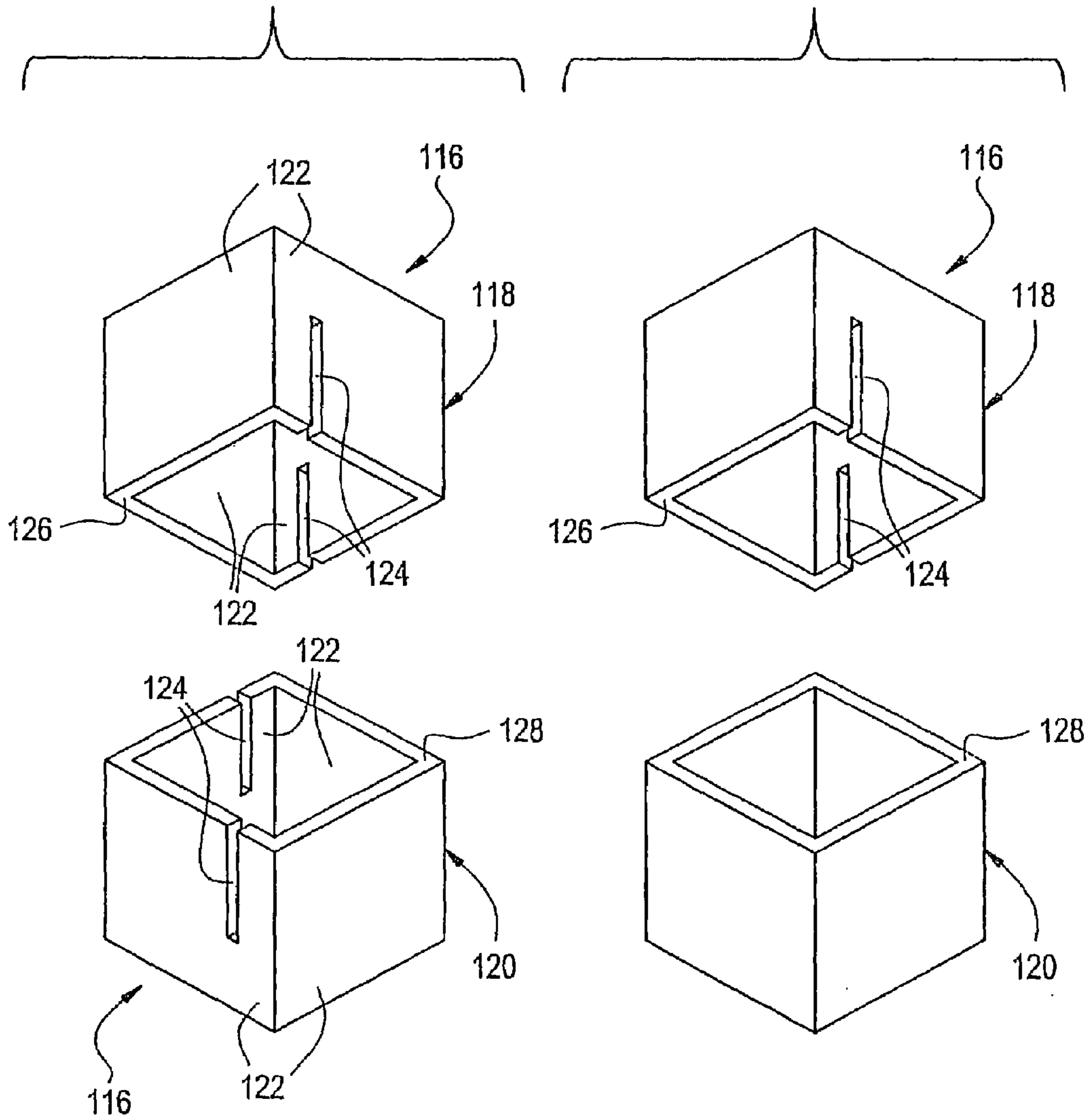
FIG. 12B
