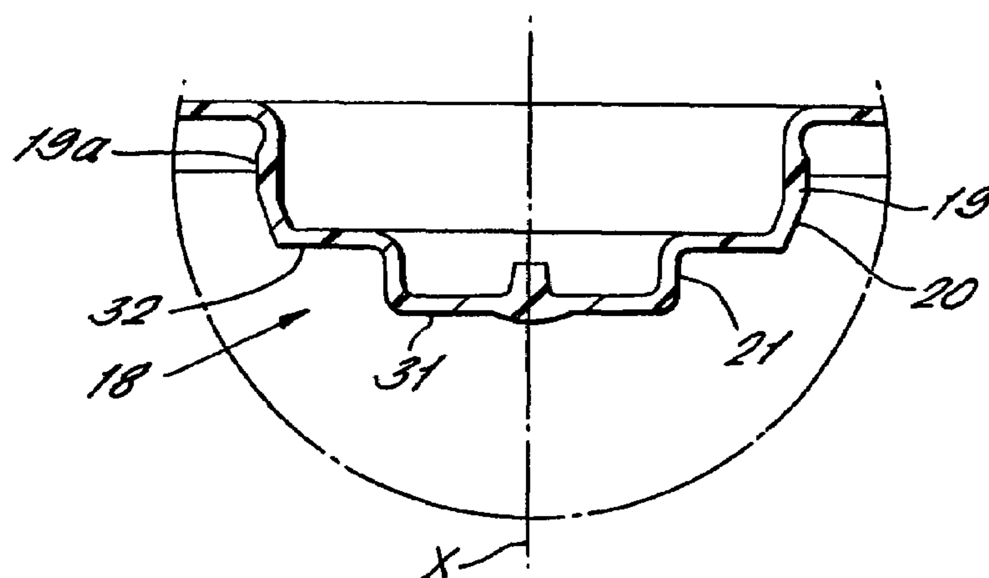
FIG. 20.
