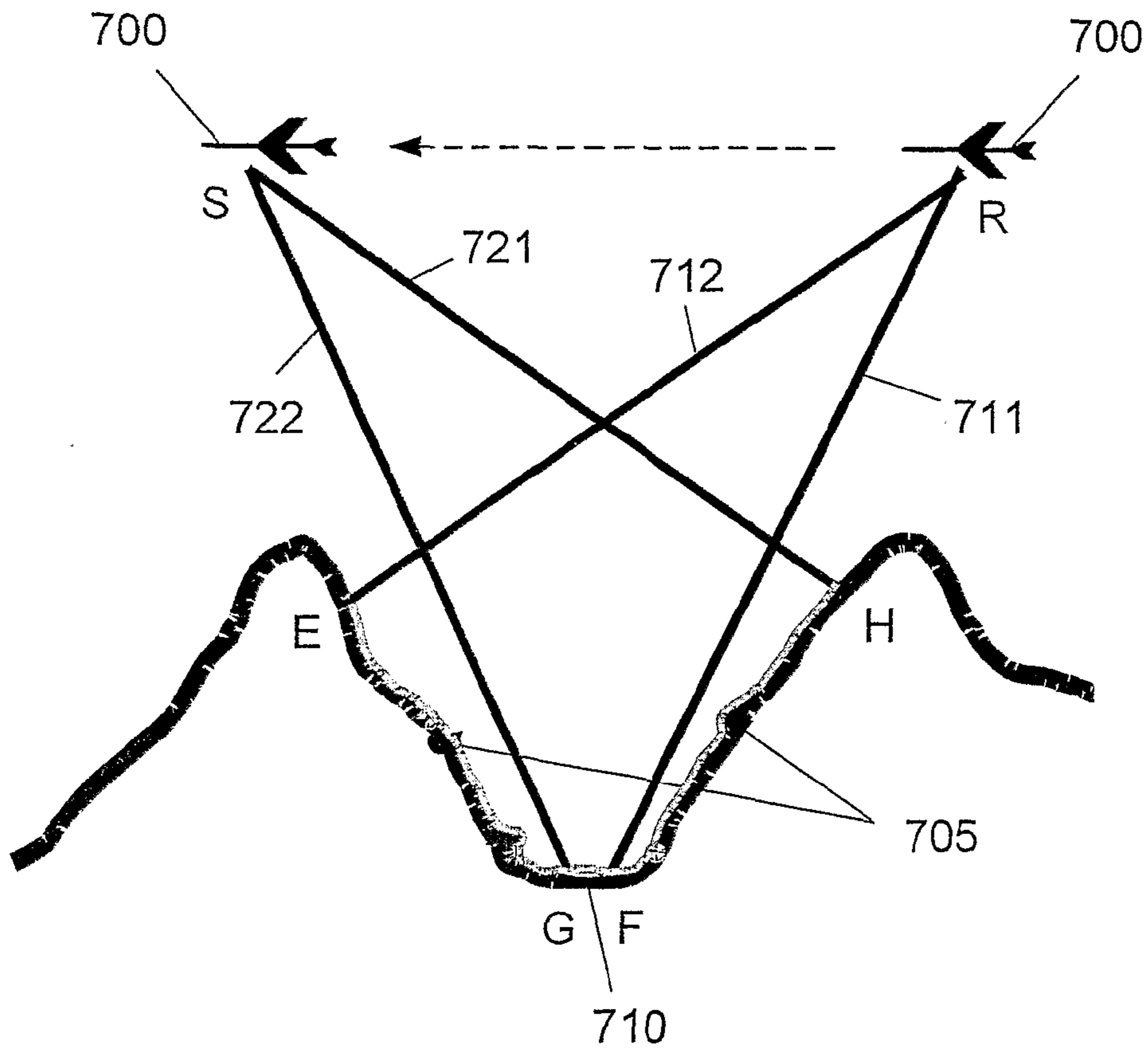
Fig. 8A
