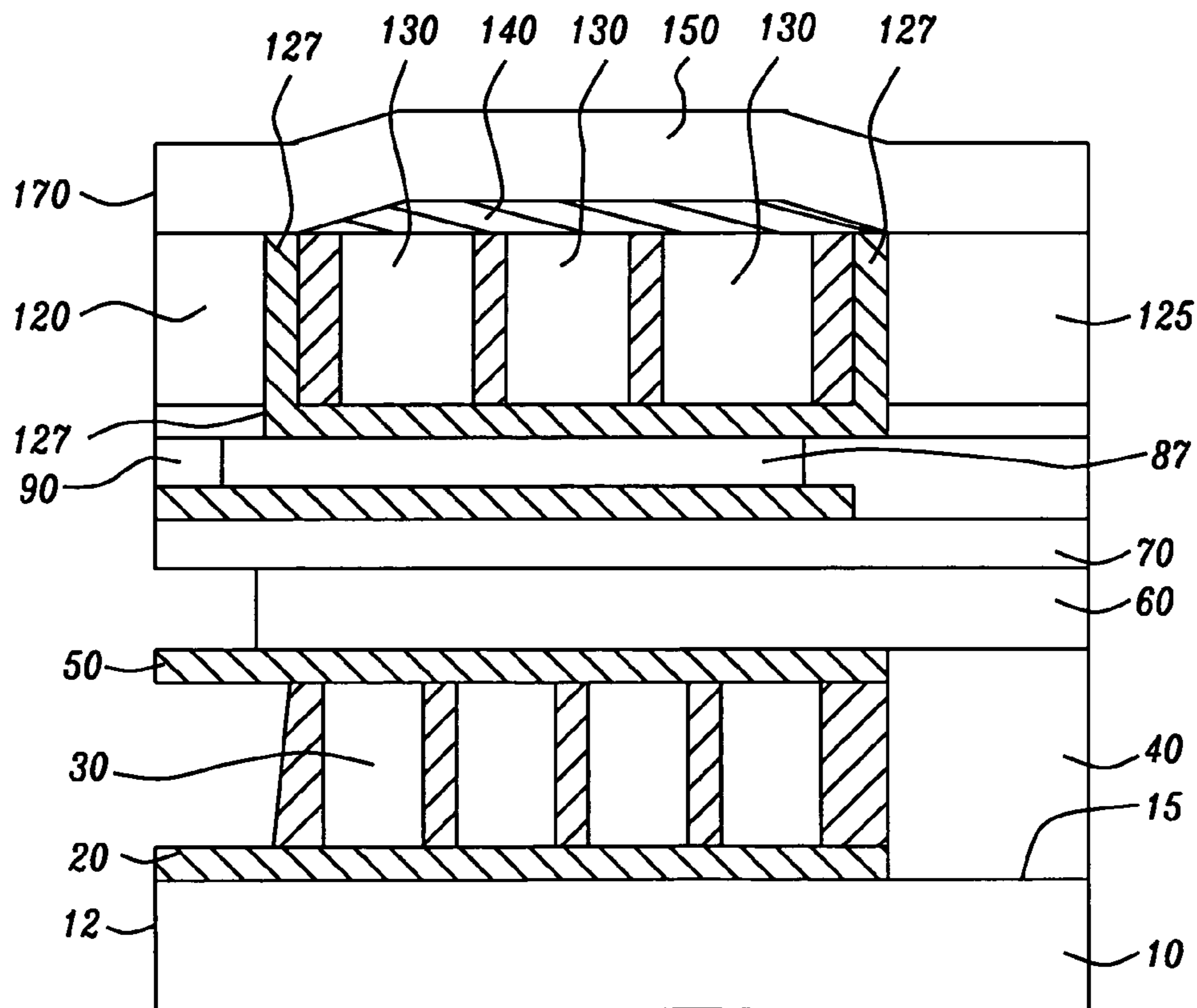
FIG. 4g
