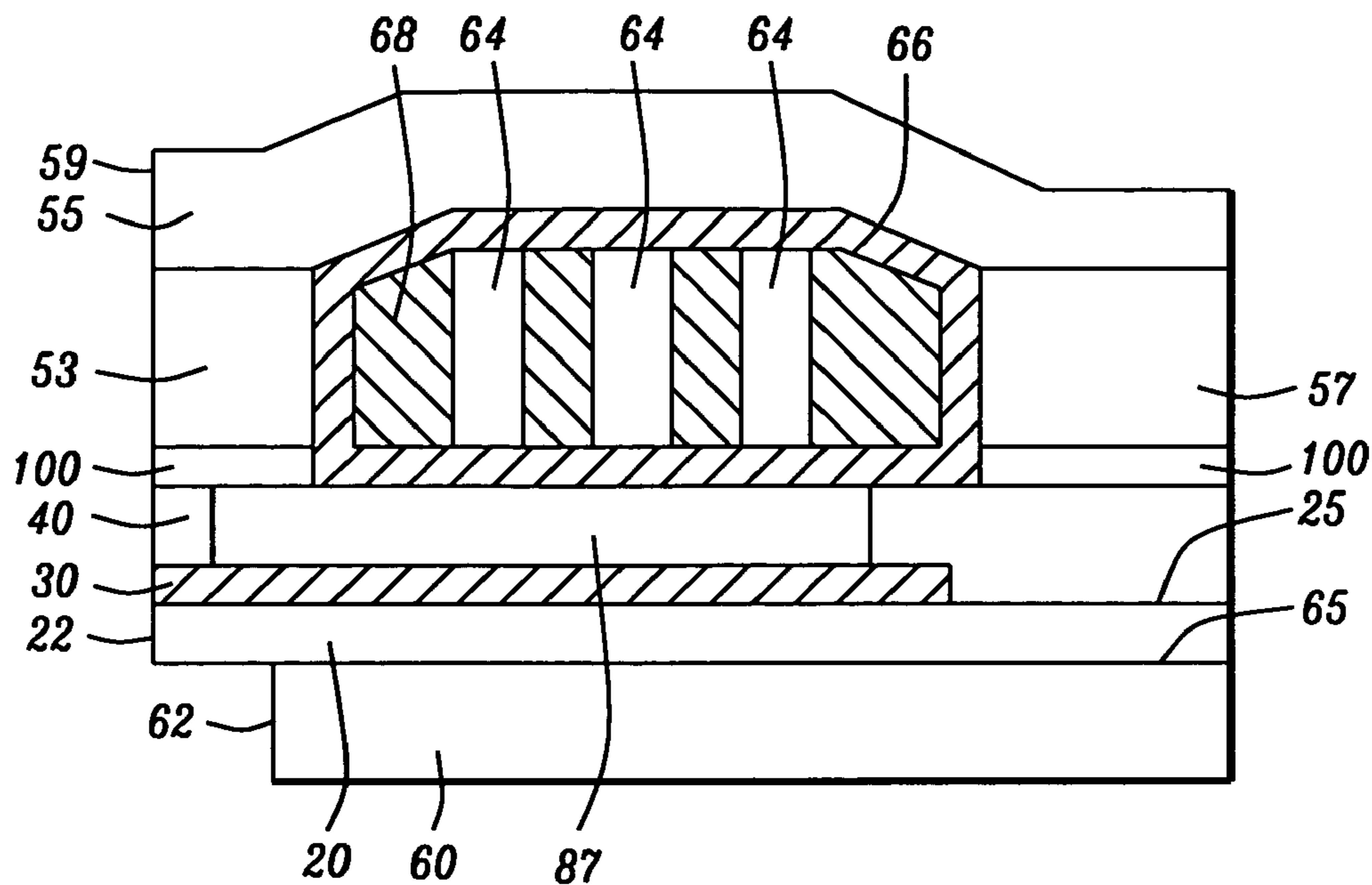
FIG. 2b
