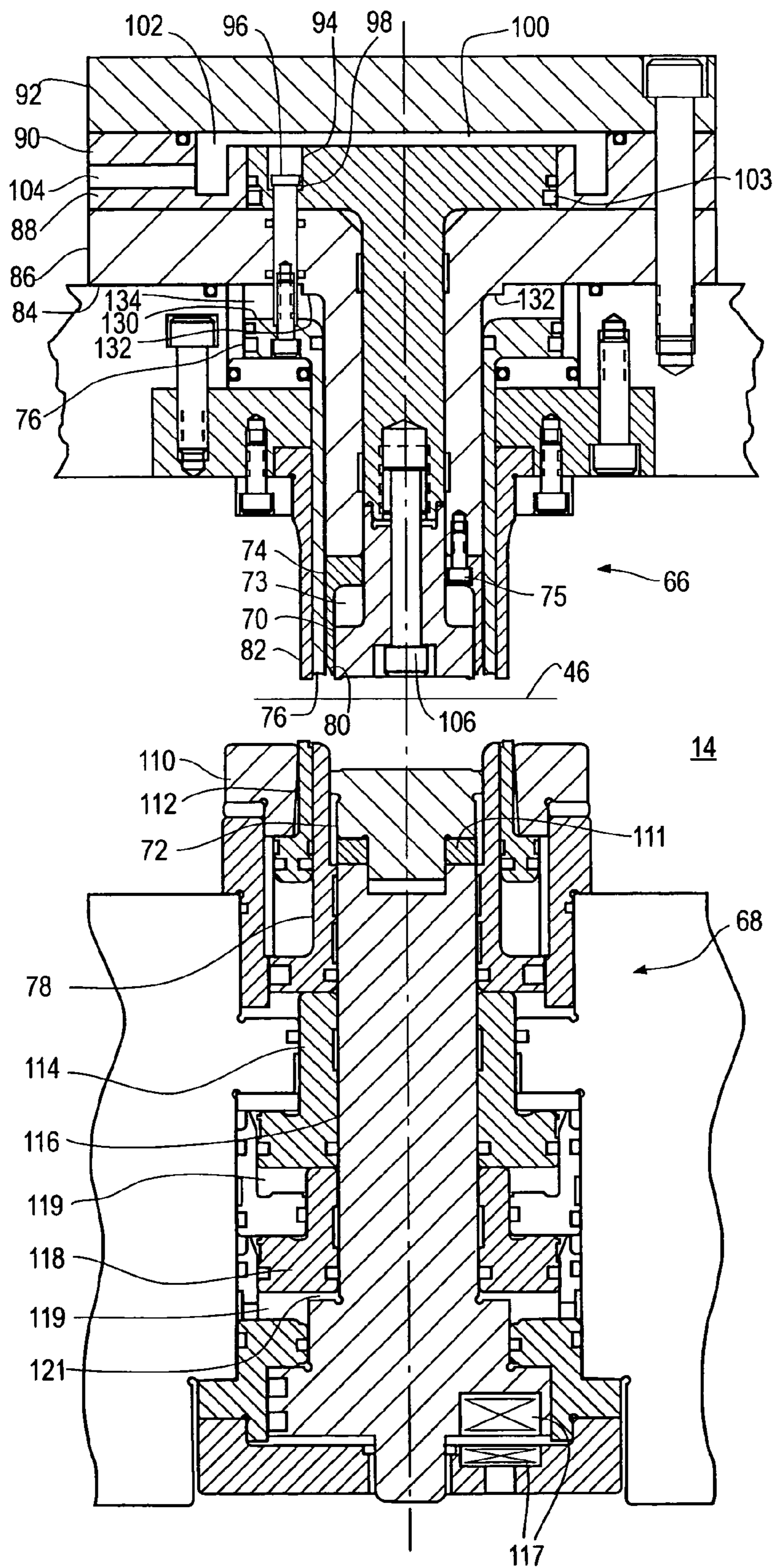
FIG. 3
