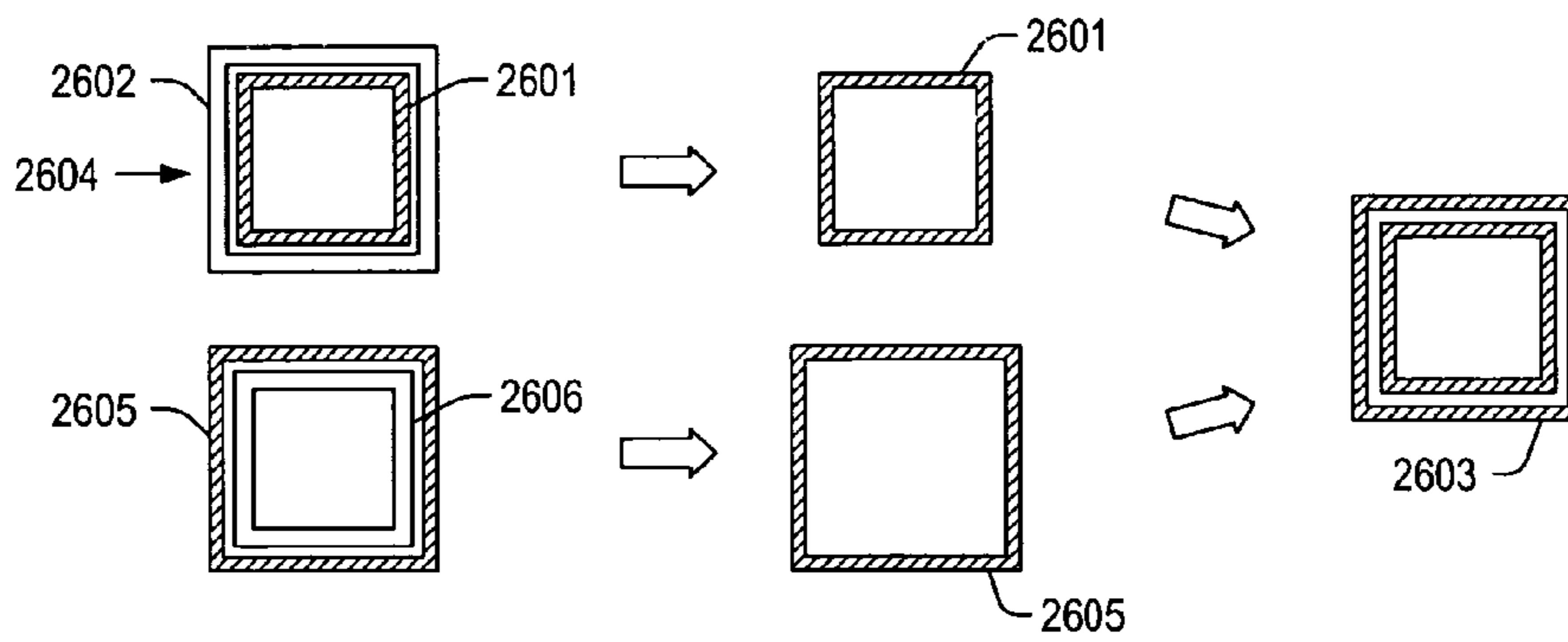
FIG. 26
