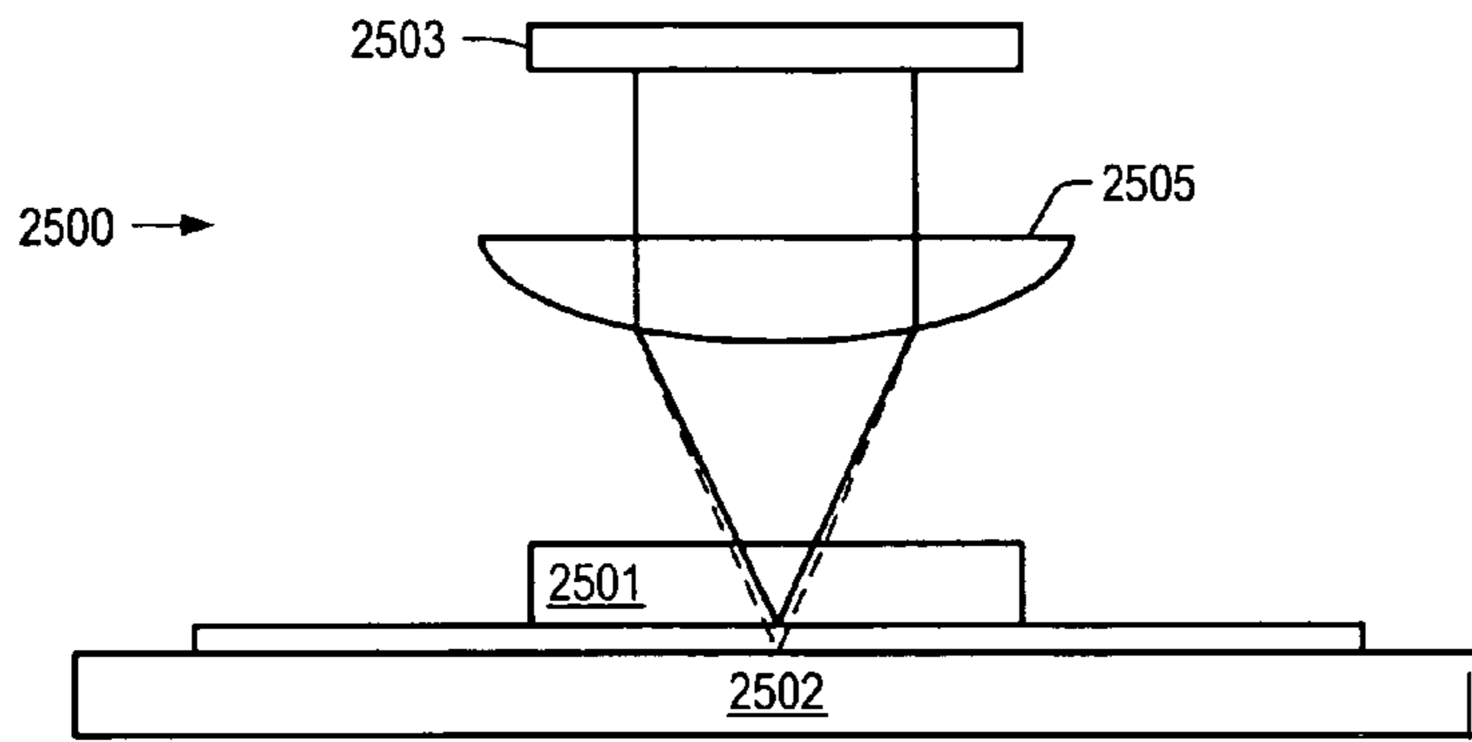
FIG. 25
