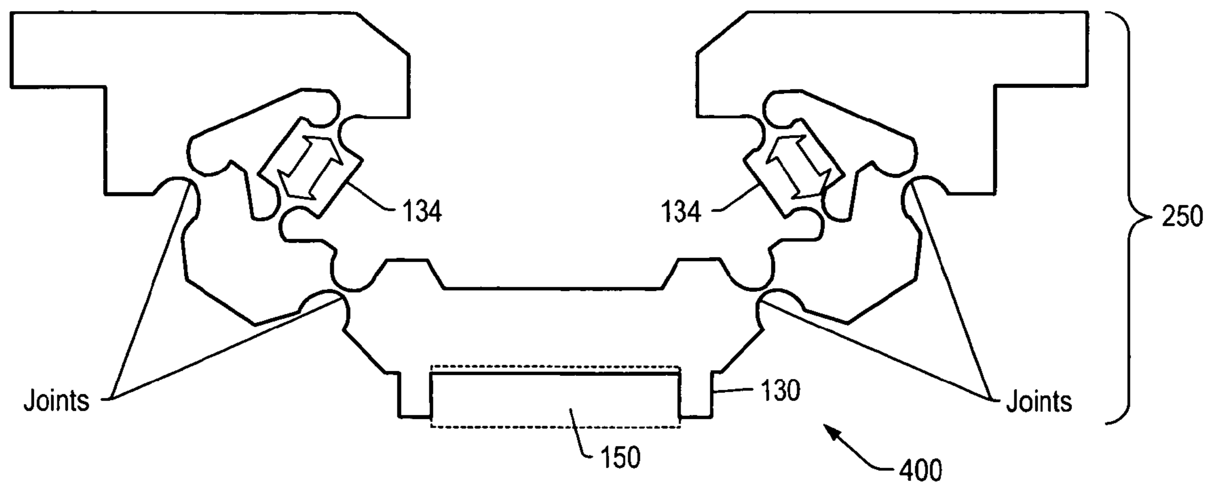
FIG. 46
