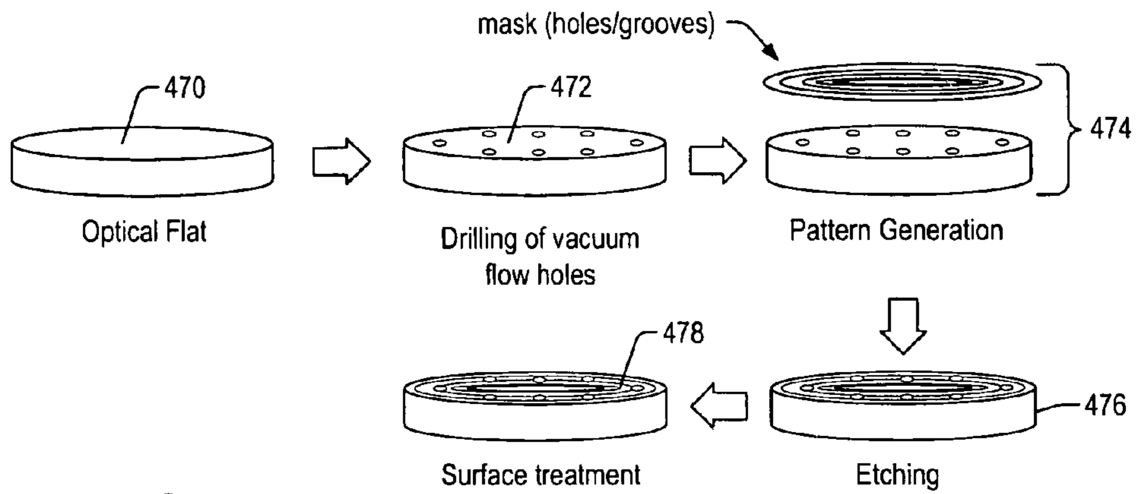
FIG. 47
