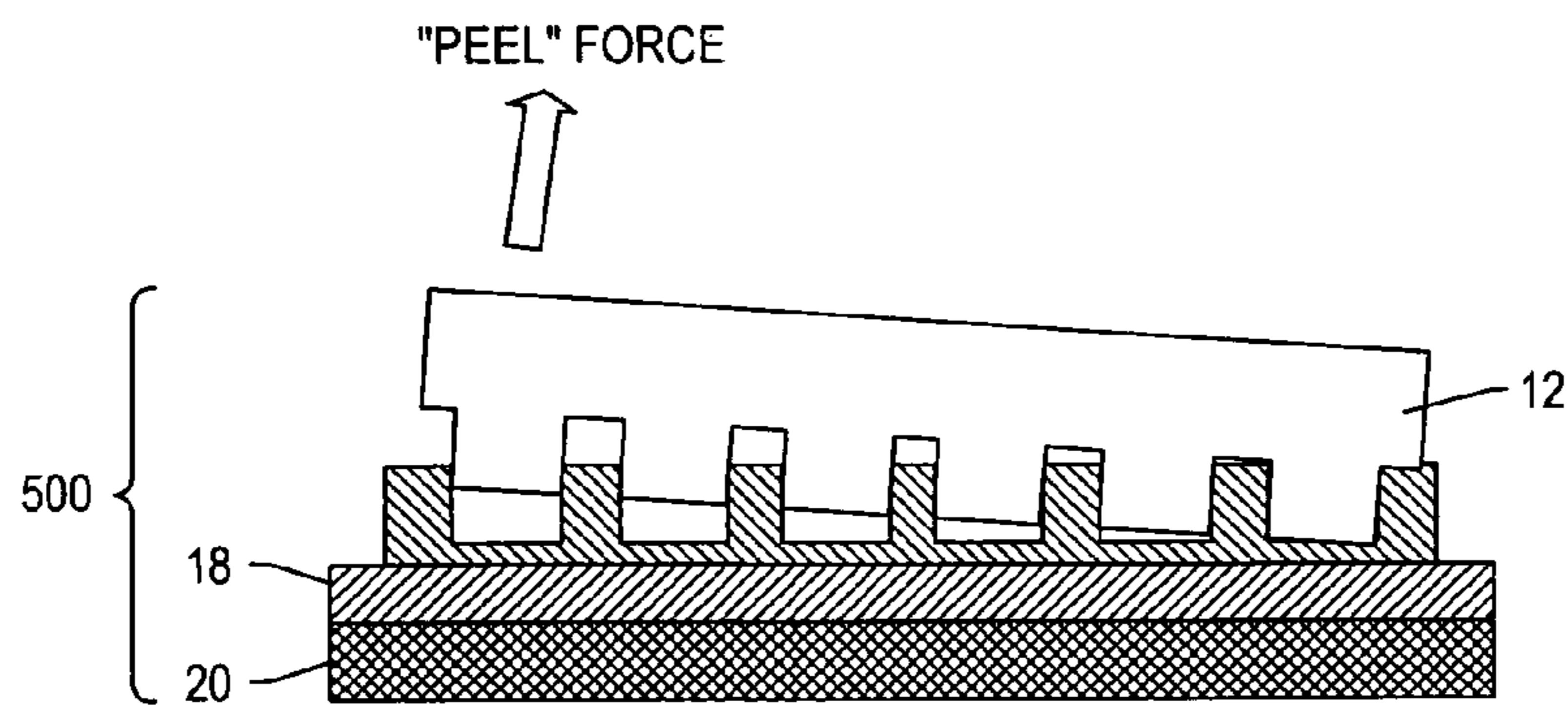
FIG. 49B
