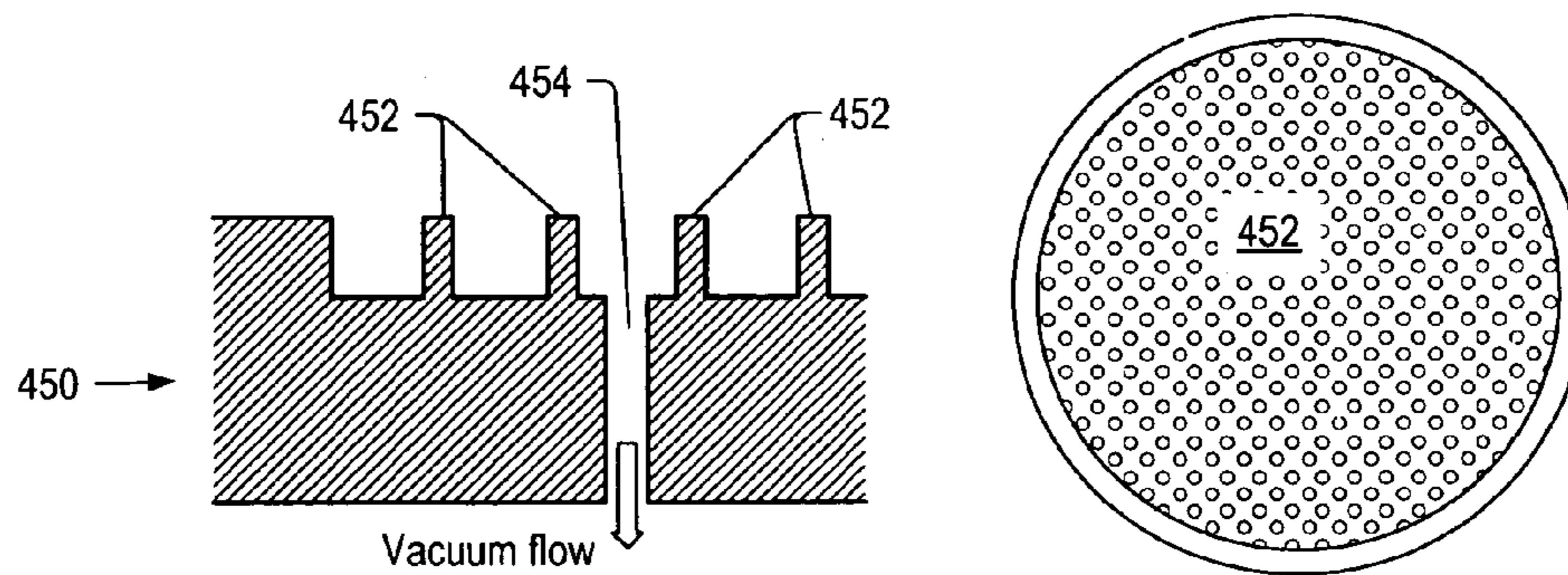
FIG. 48A
