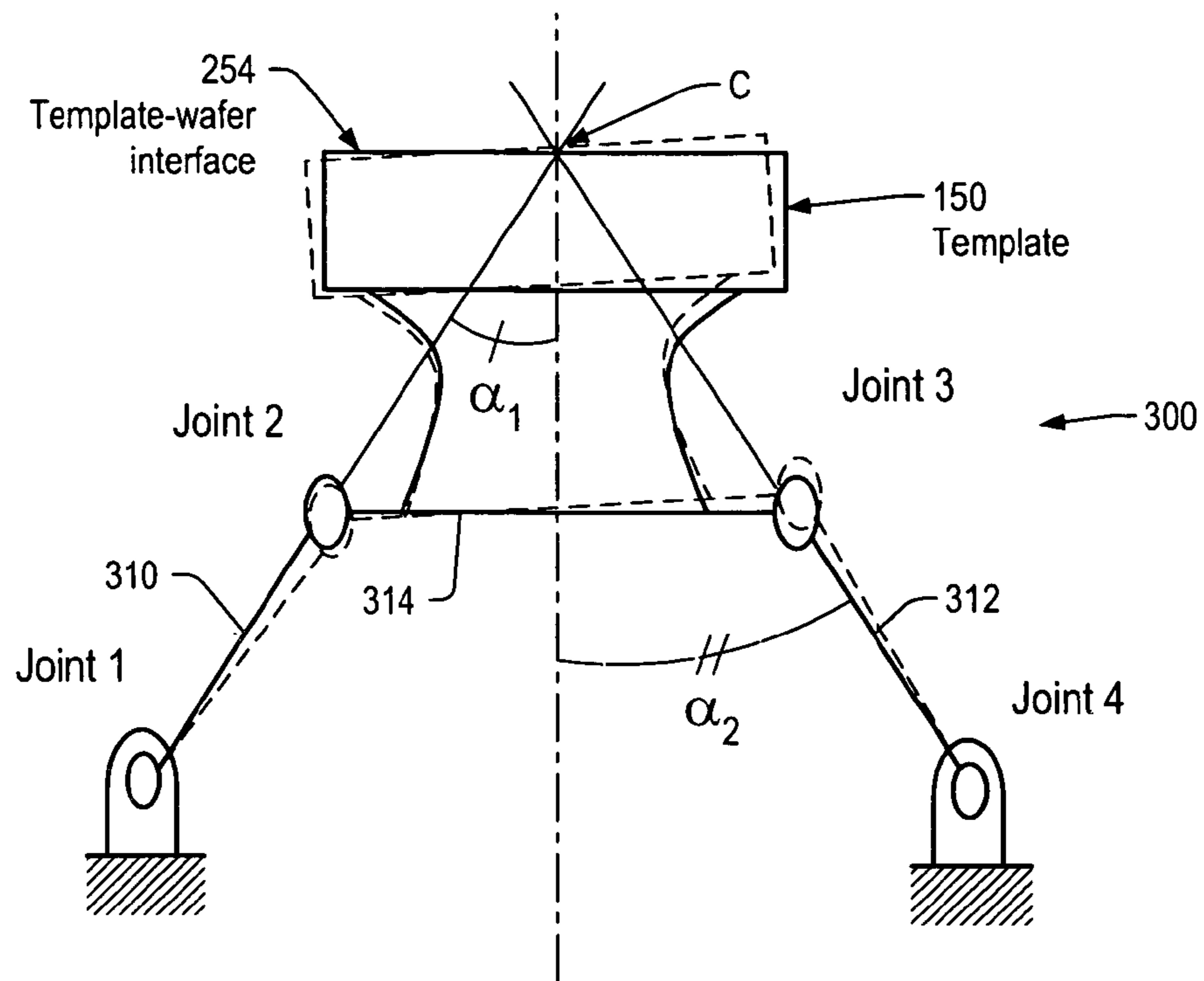
FIG. 45
