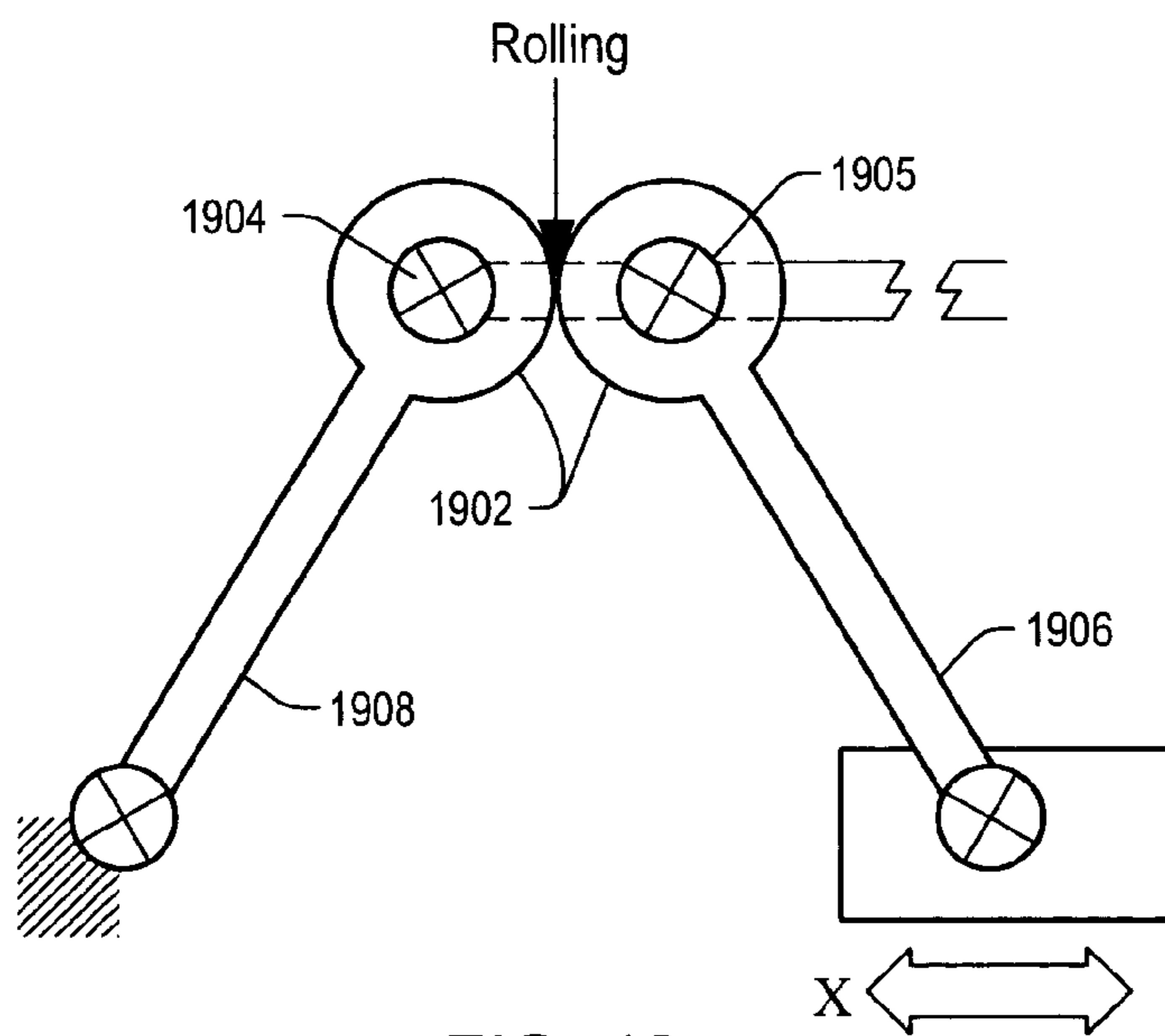
FIG. 19
