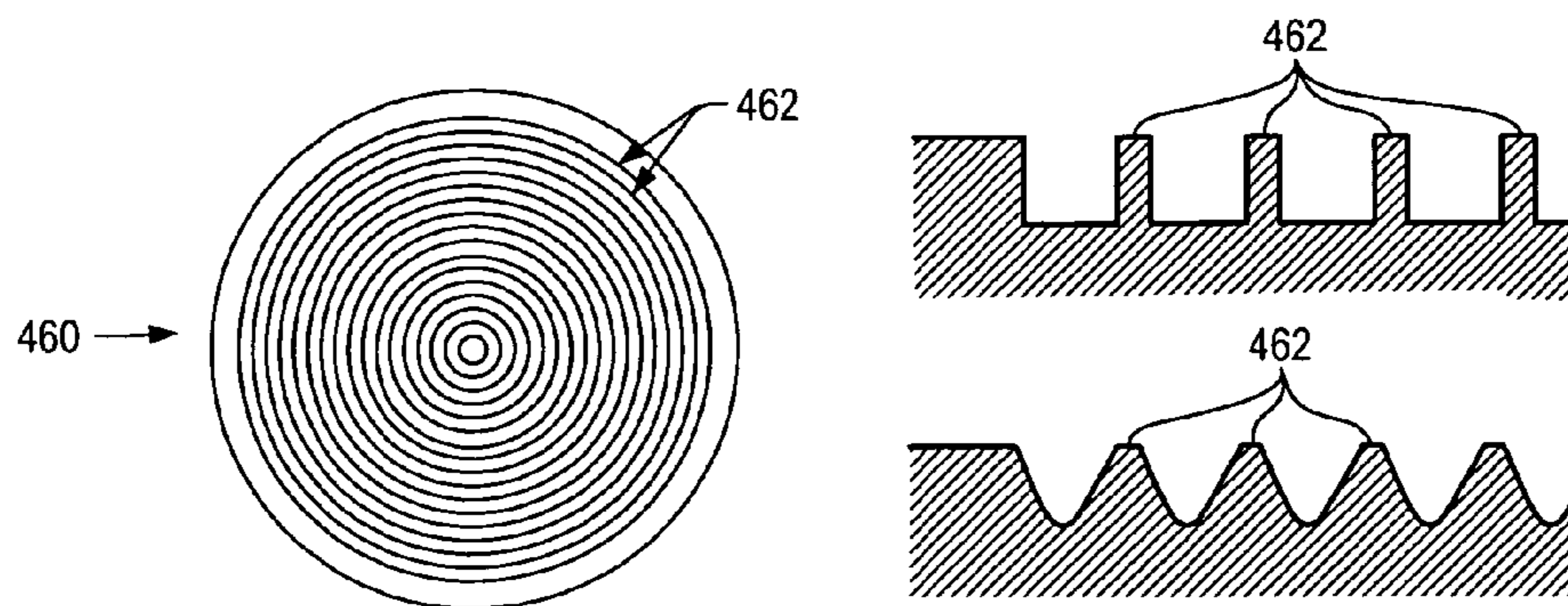
FIG. 48B
