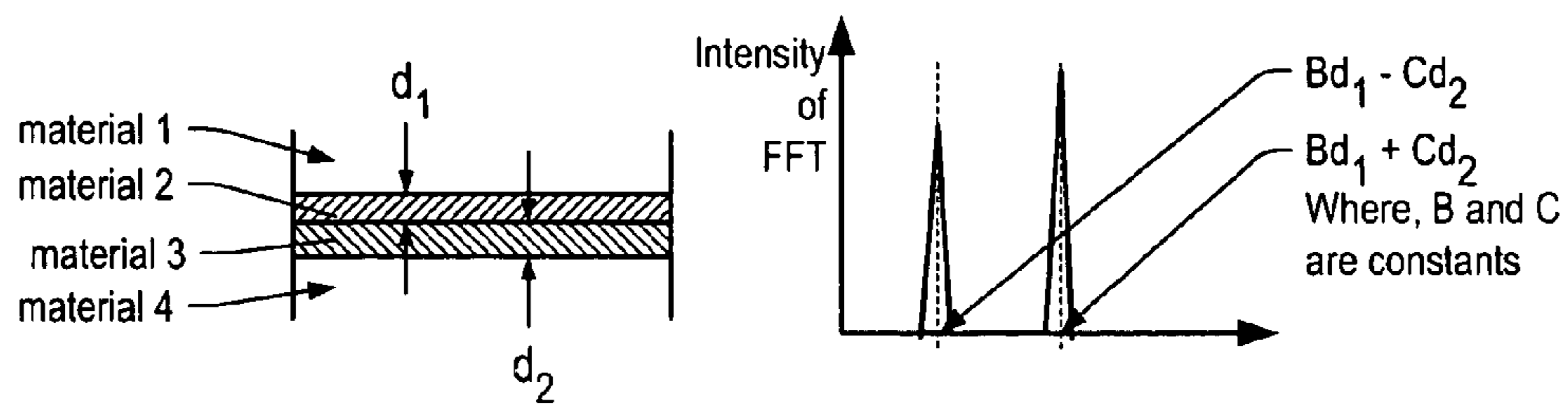
FIG. 35
