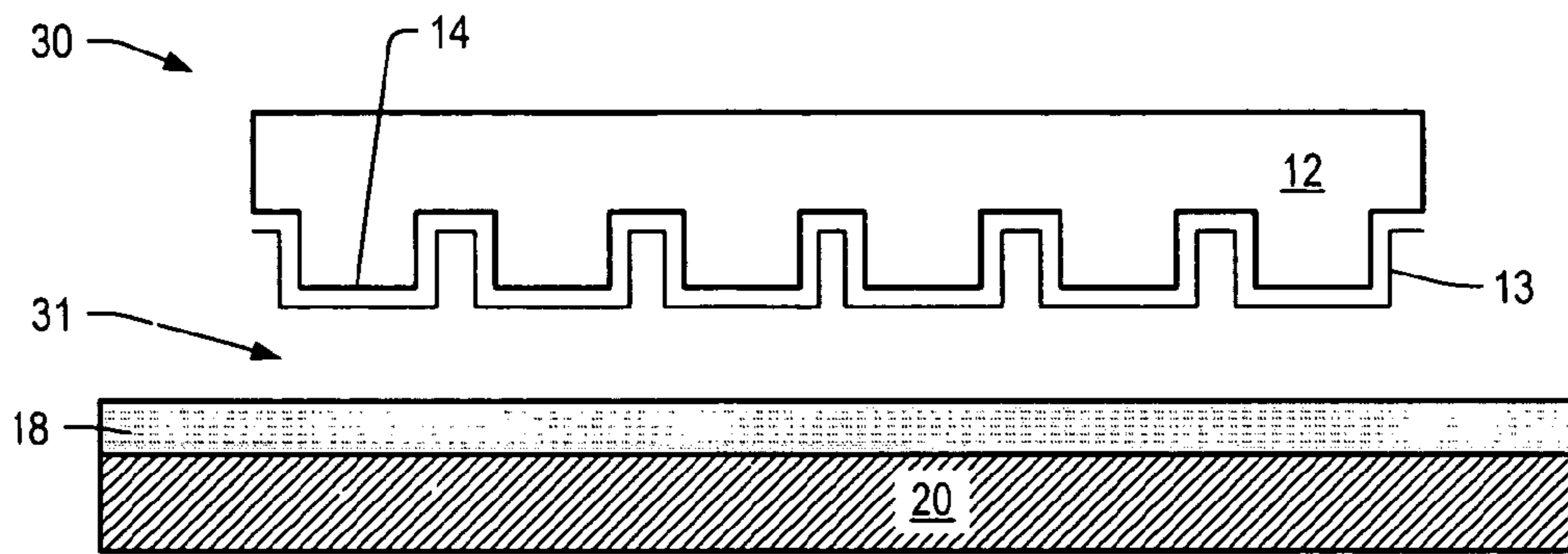
FIG. 2A
