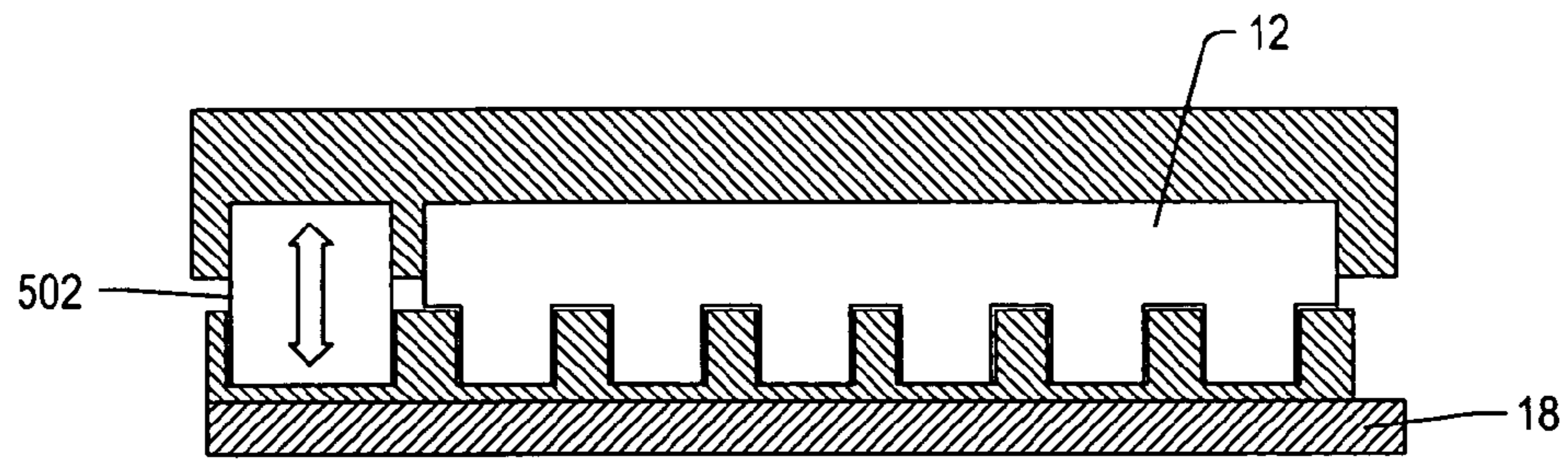
FIG. 50A
