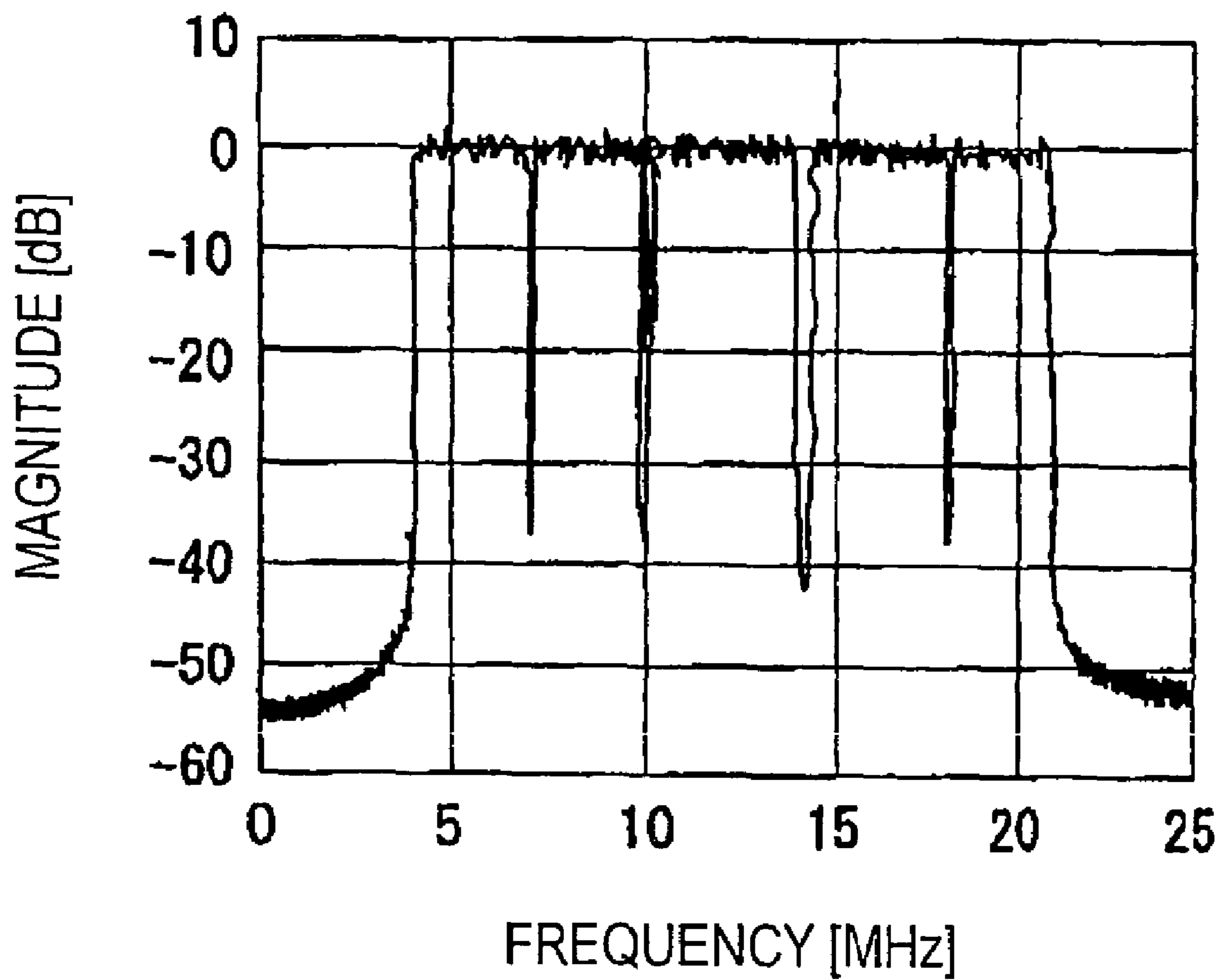
WOFDM SPECTRUM
