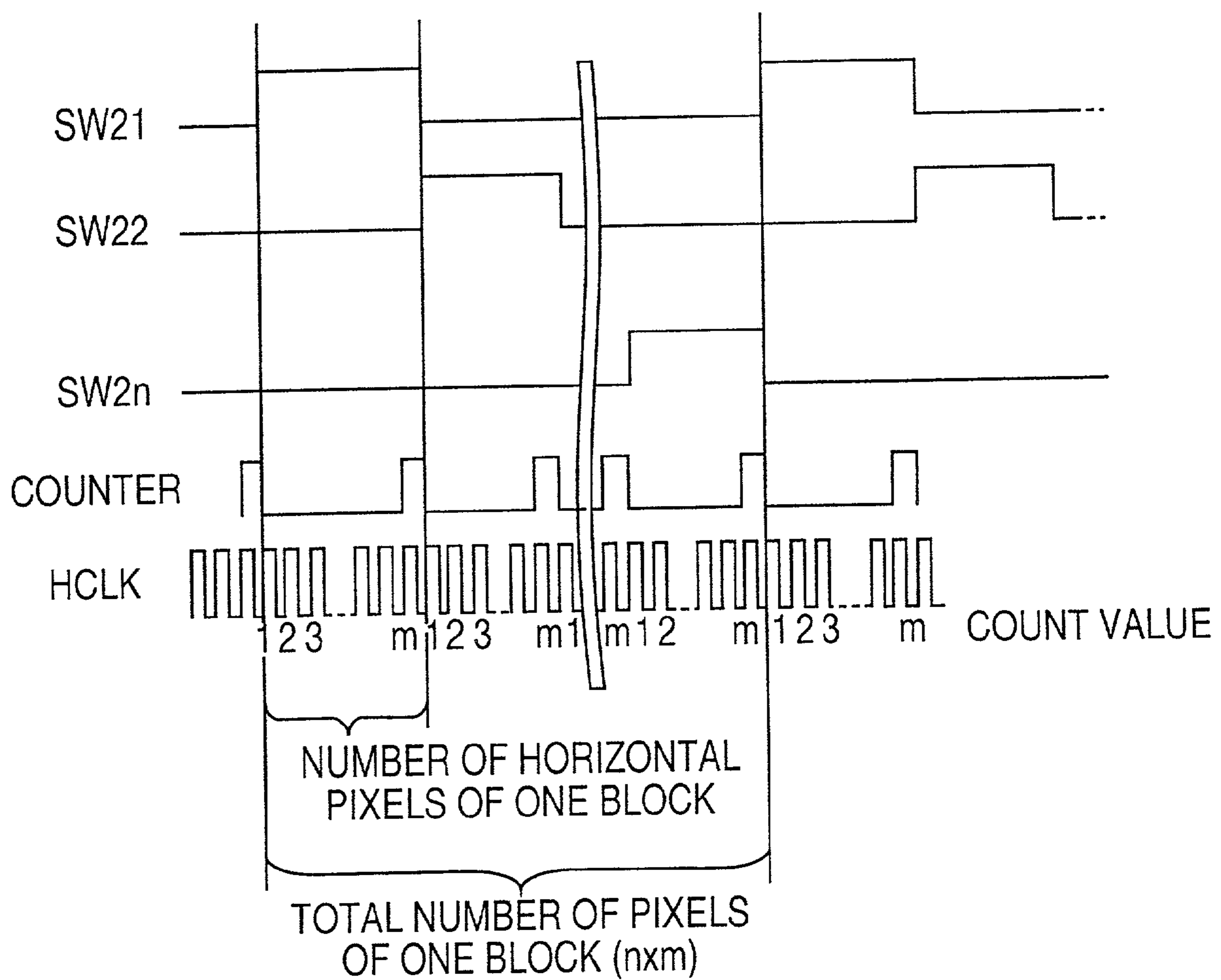
FIG. 12
