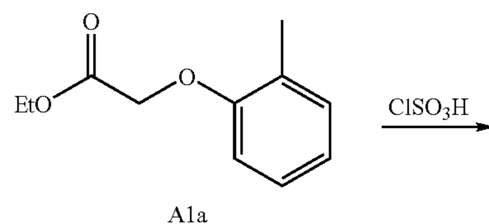
Scheme A1
