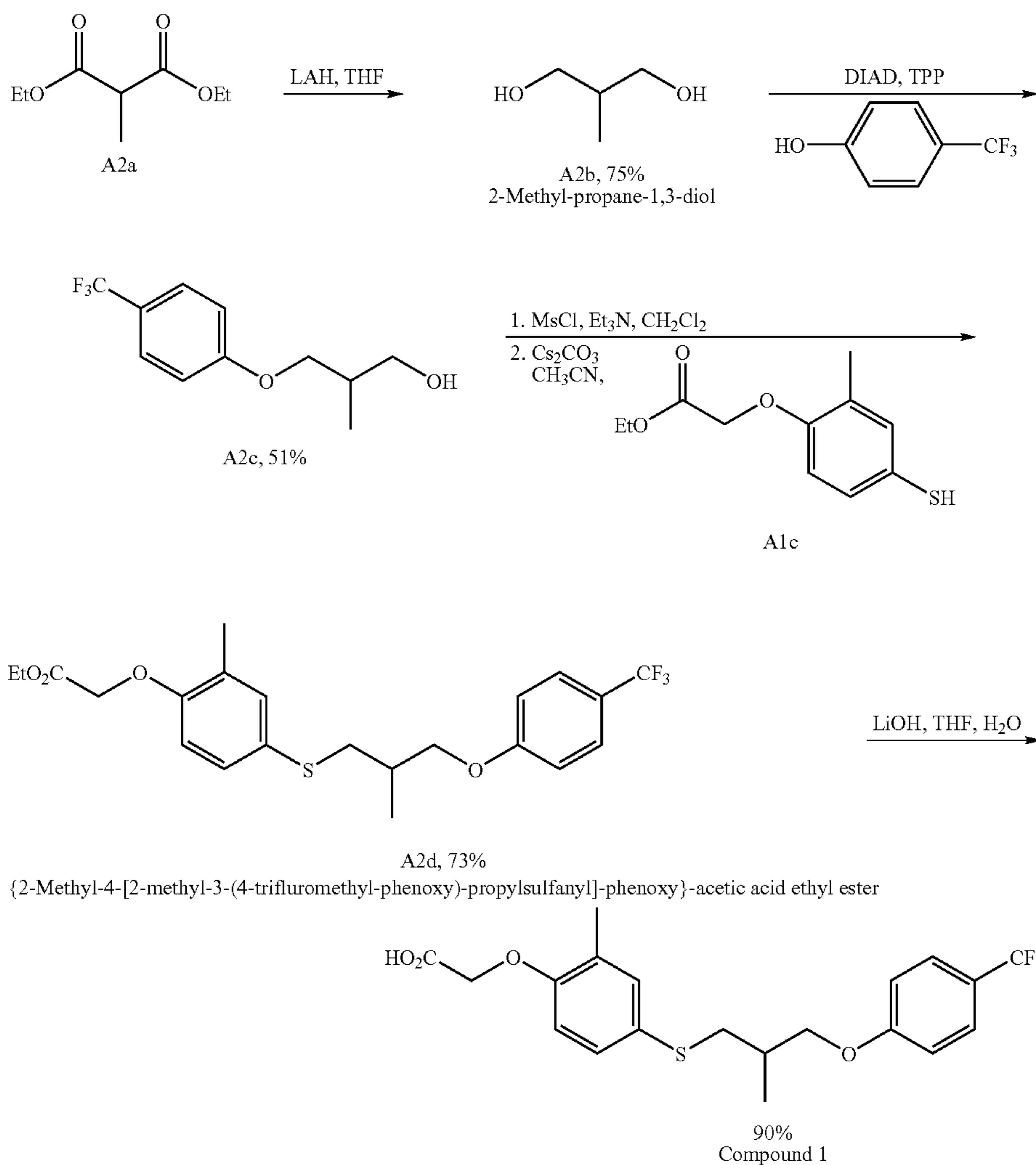
Scheme A2
