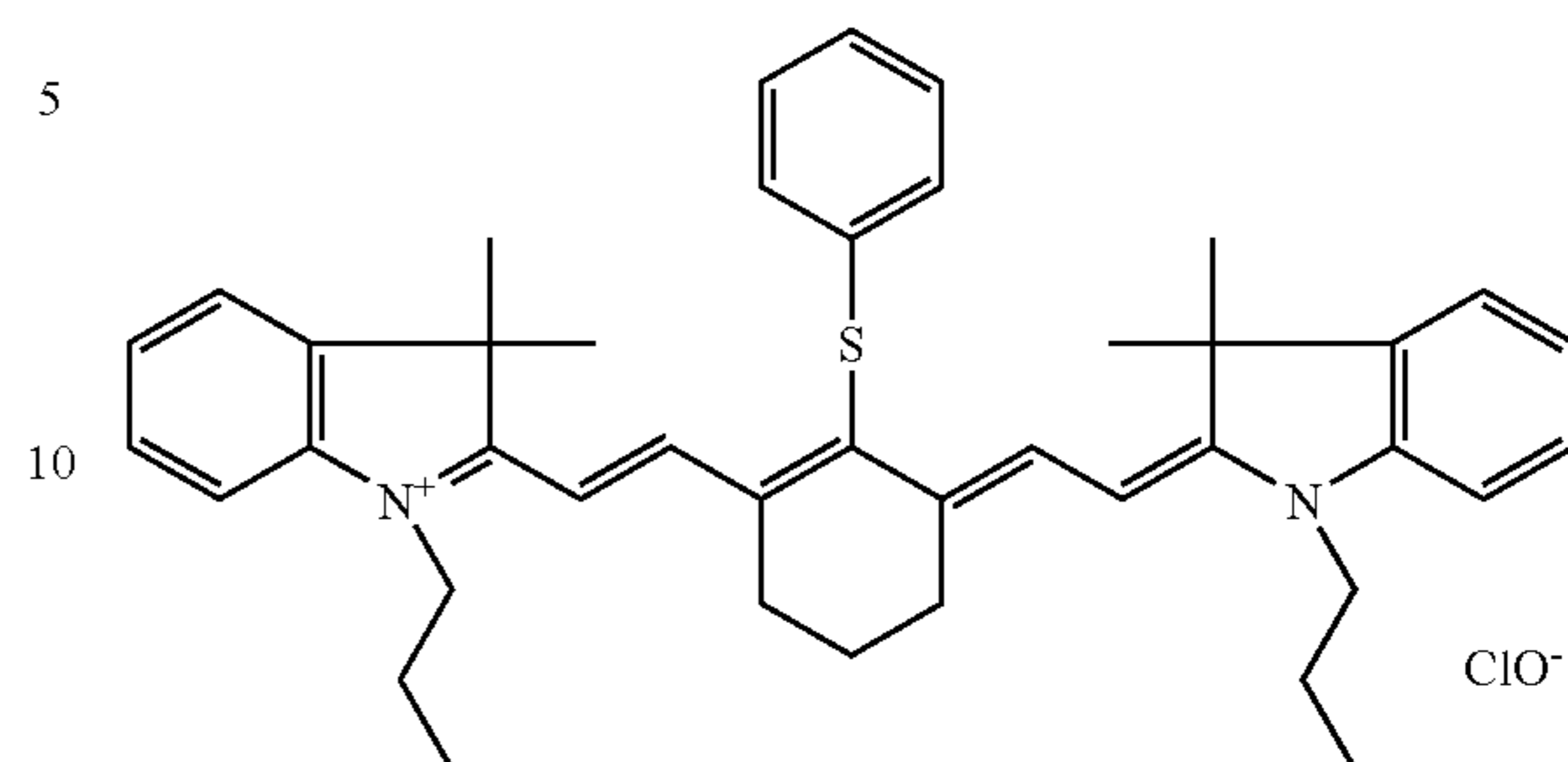
IR 792 Perchlorate.
