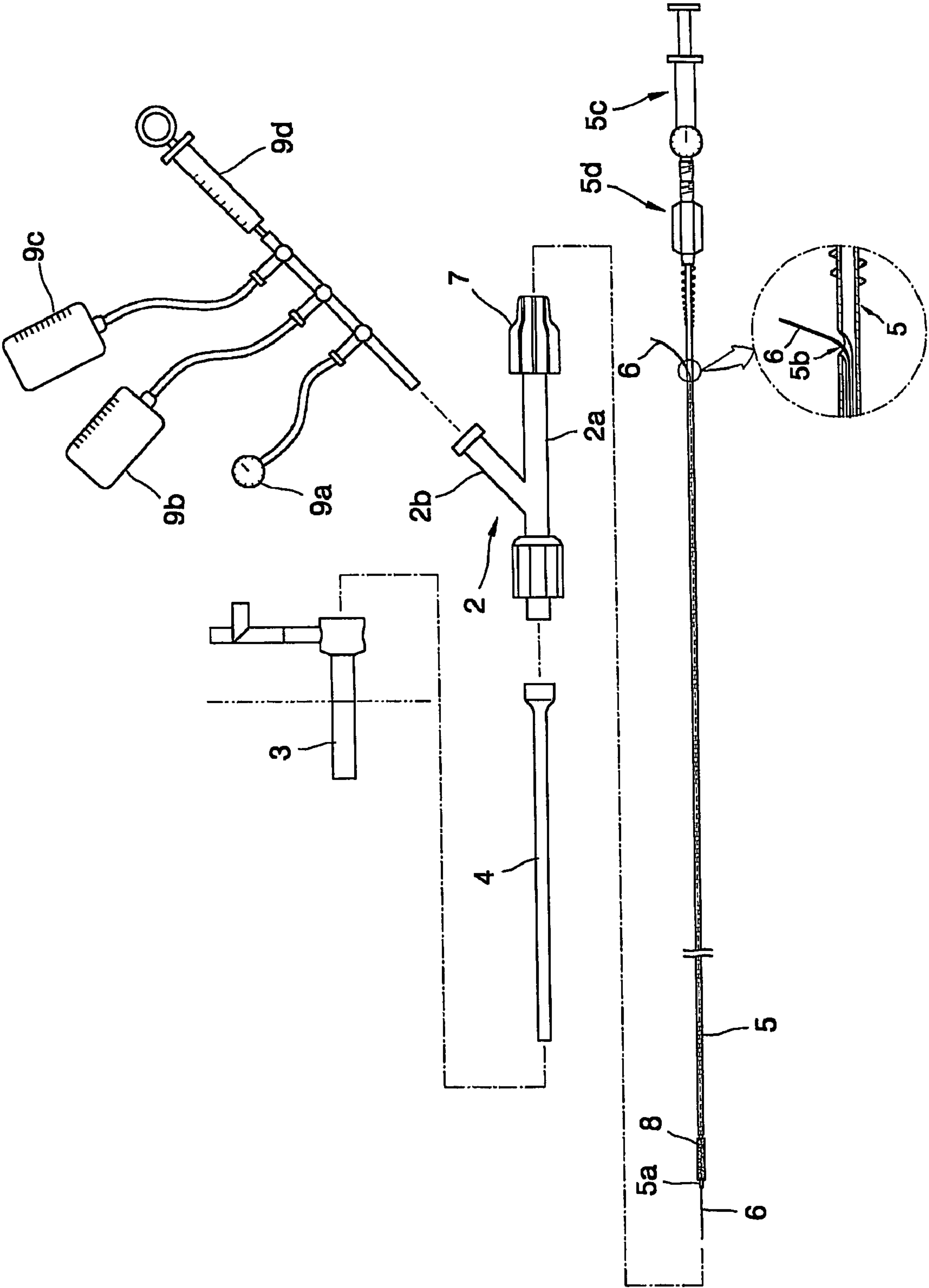
FIG. 1C
