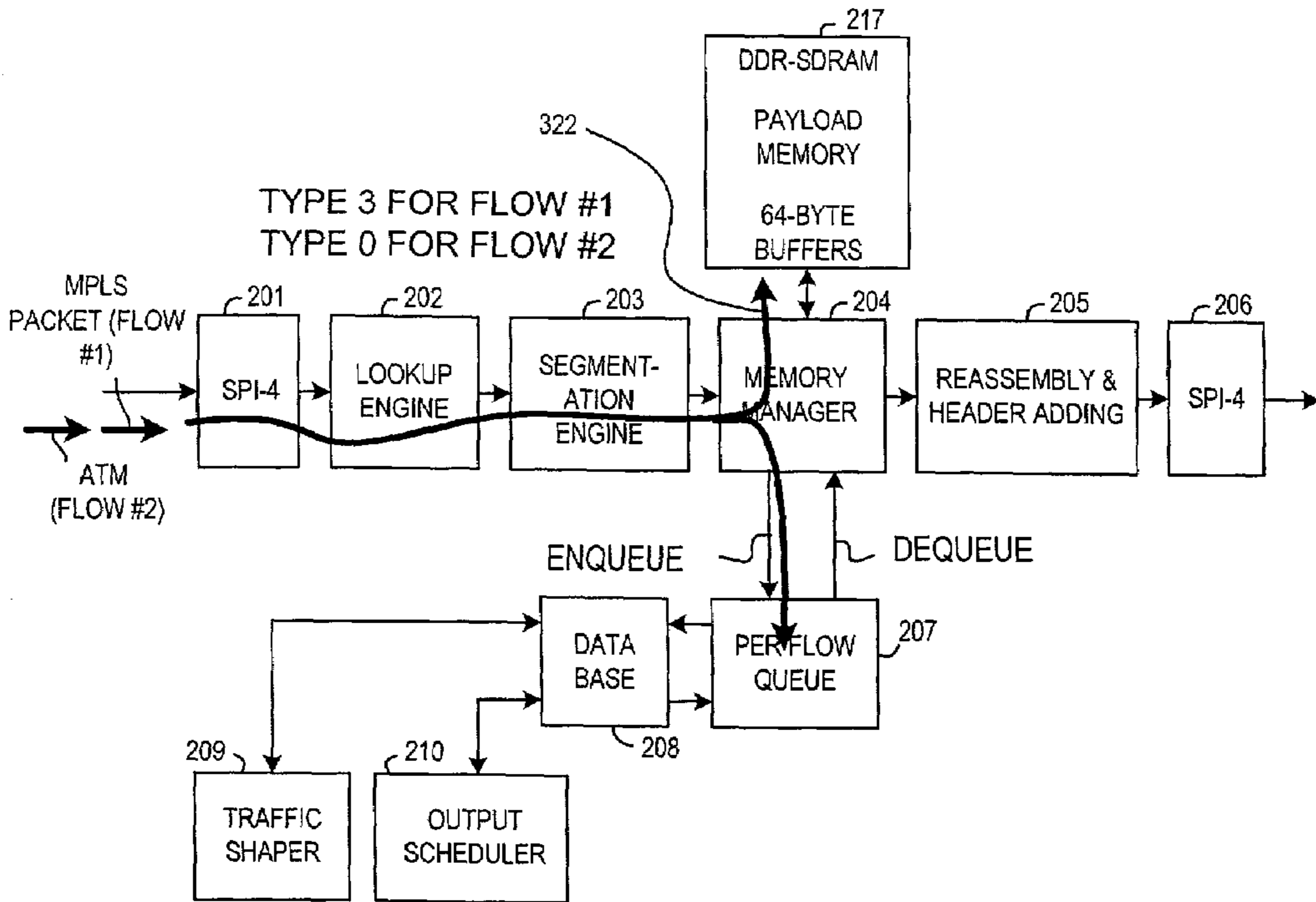
INGRESS MODE FIG. 13
