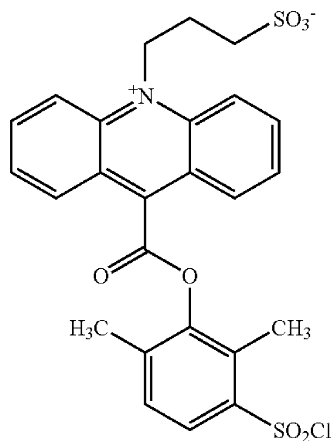
SPAE
