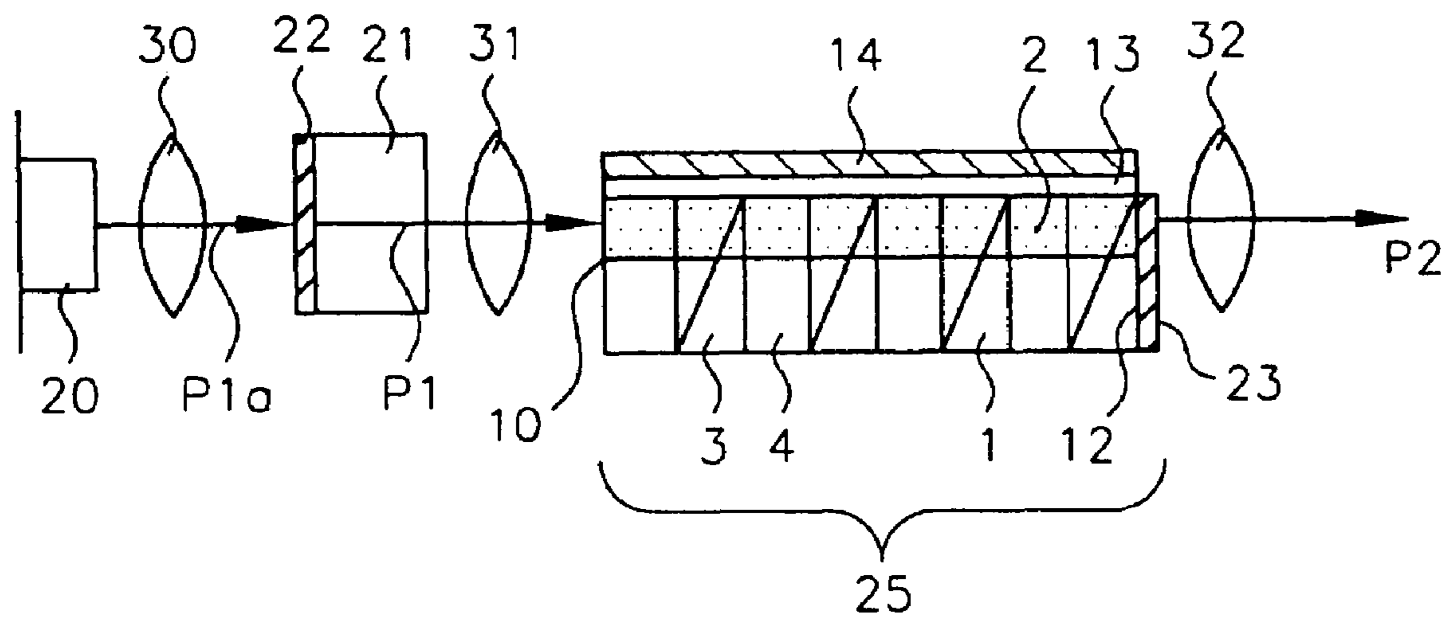
FIG. 17
