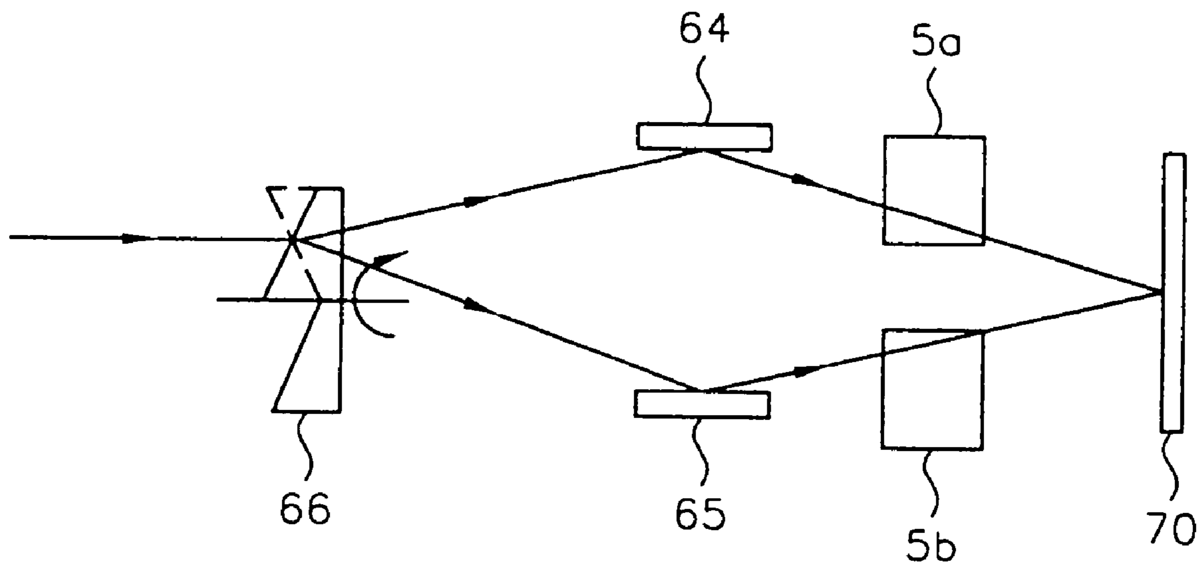
FIG. 30
