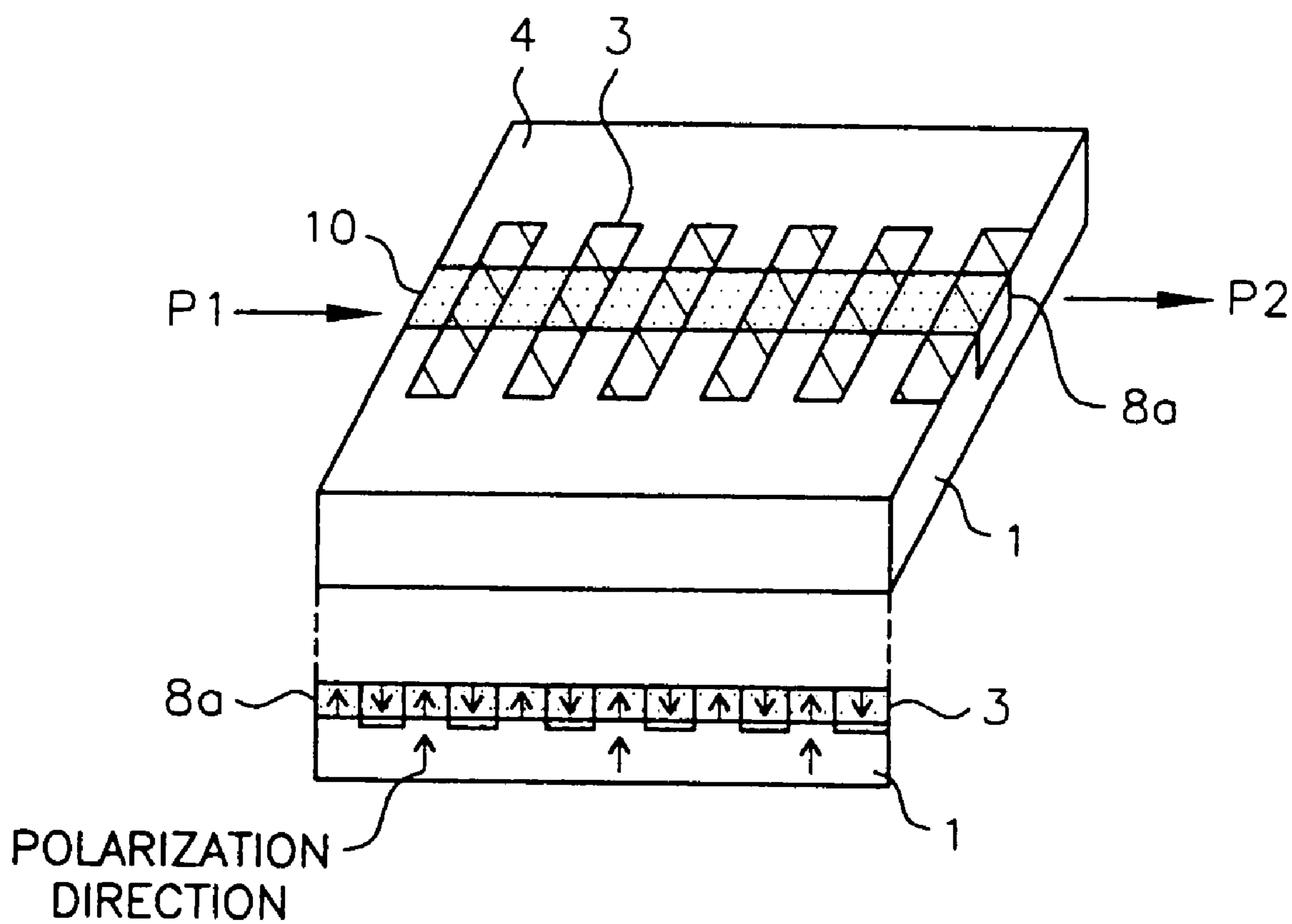
FIG. 7
