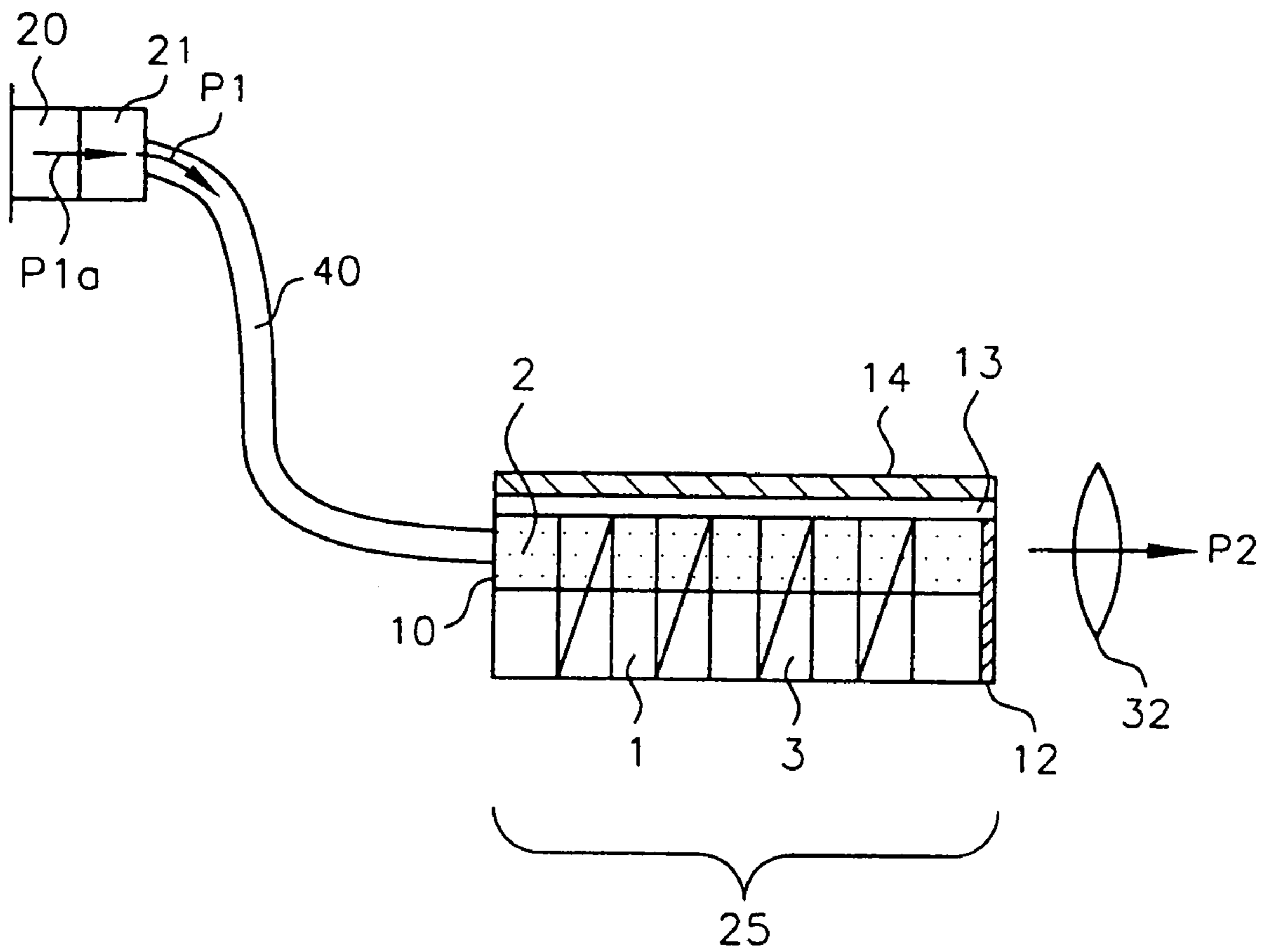
FIG. 26
