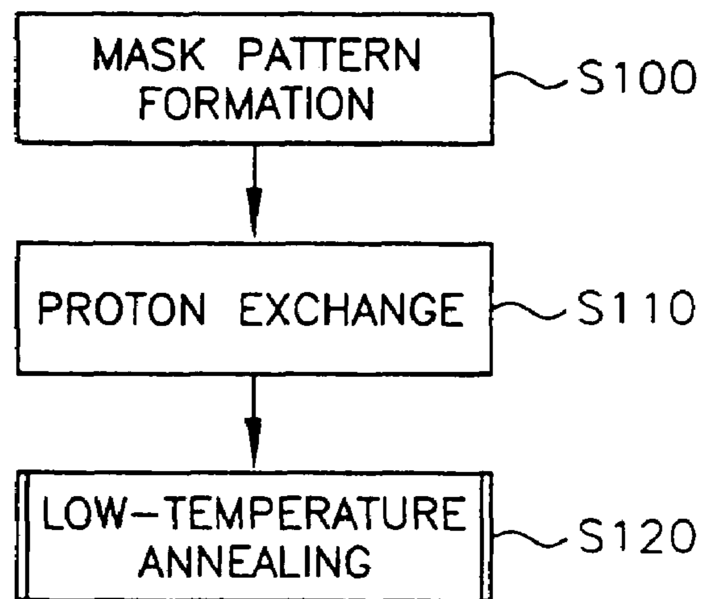
FIG. 14
