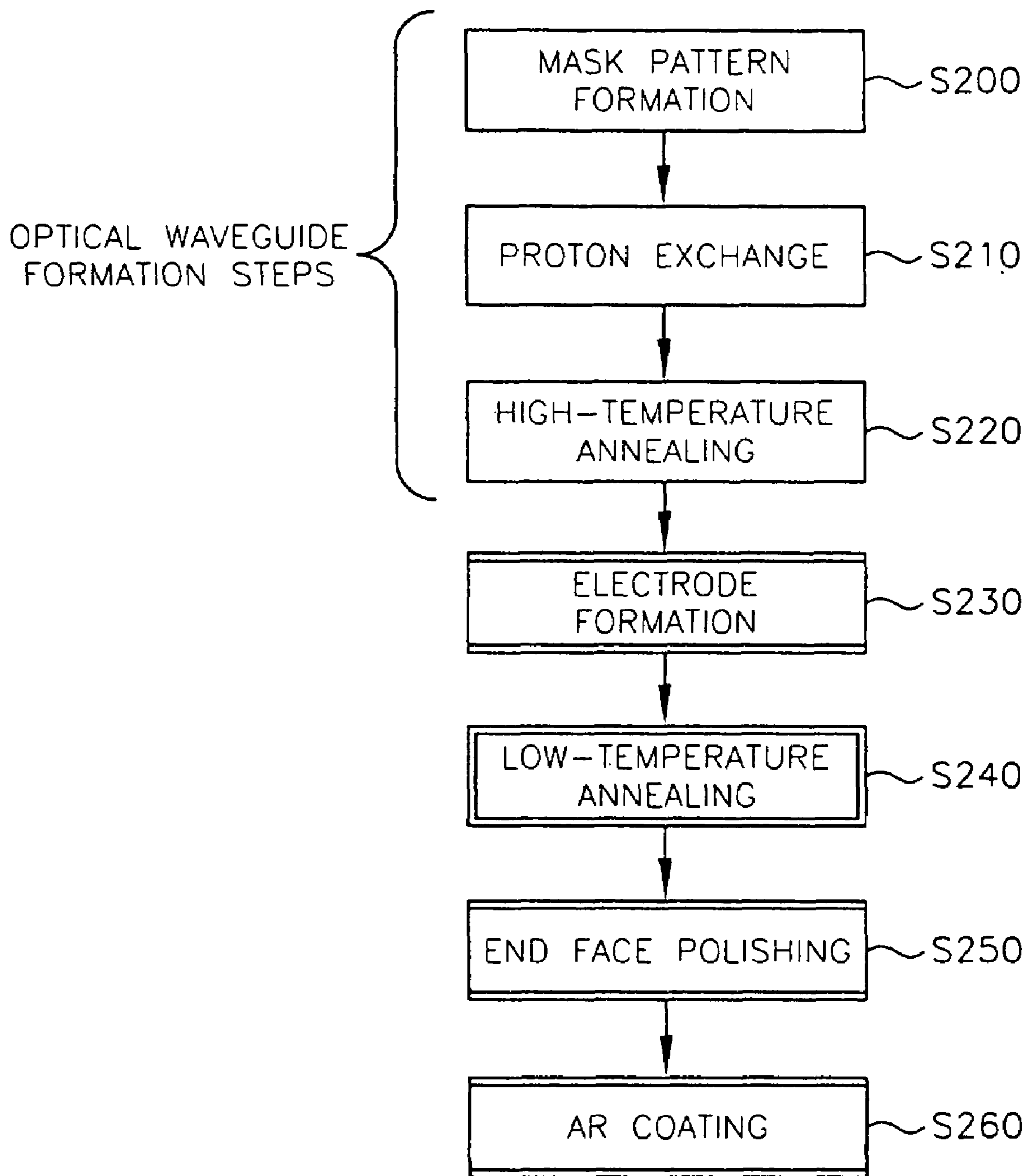
FIG. 16
