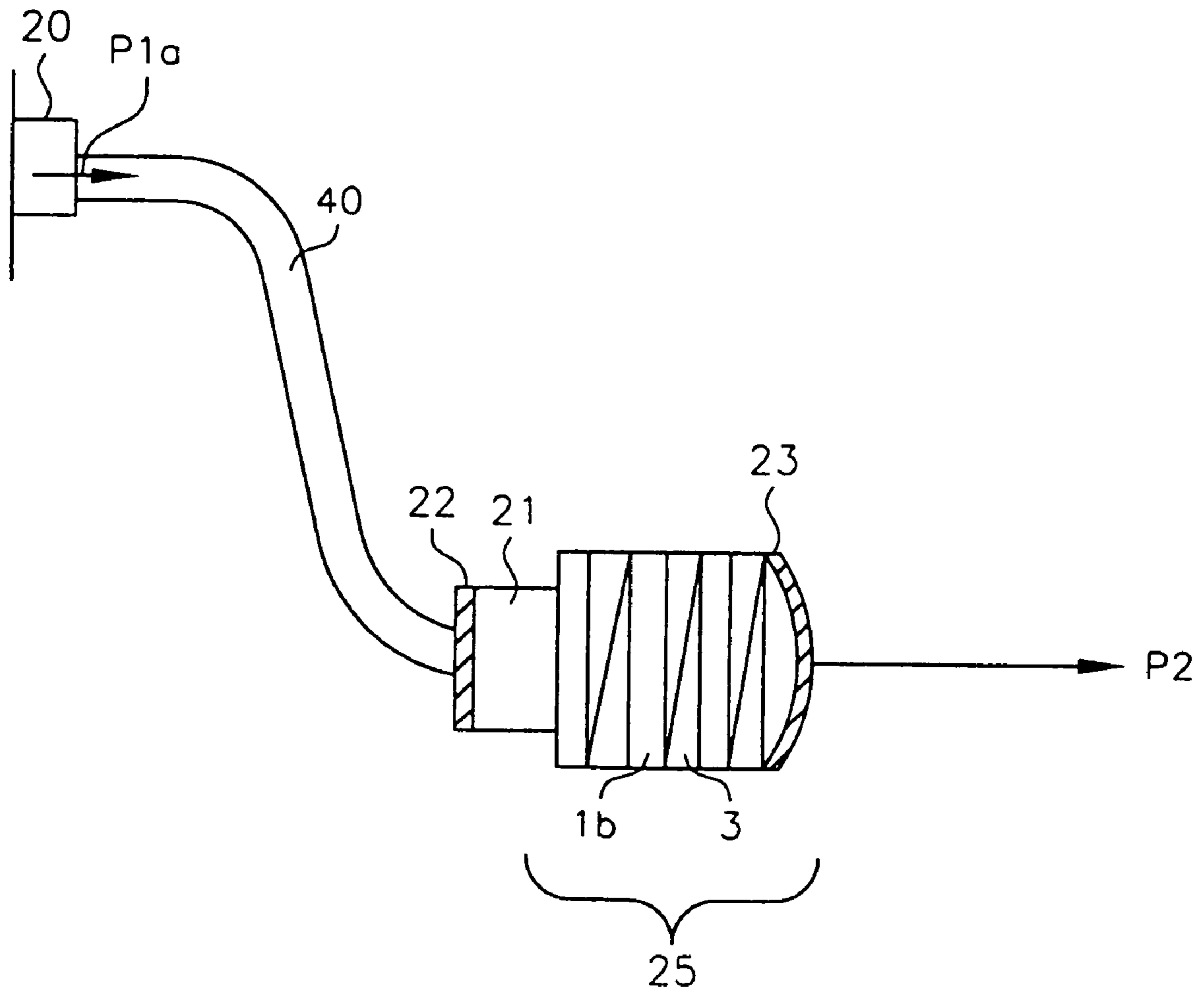
FIG. 25
