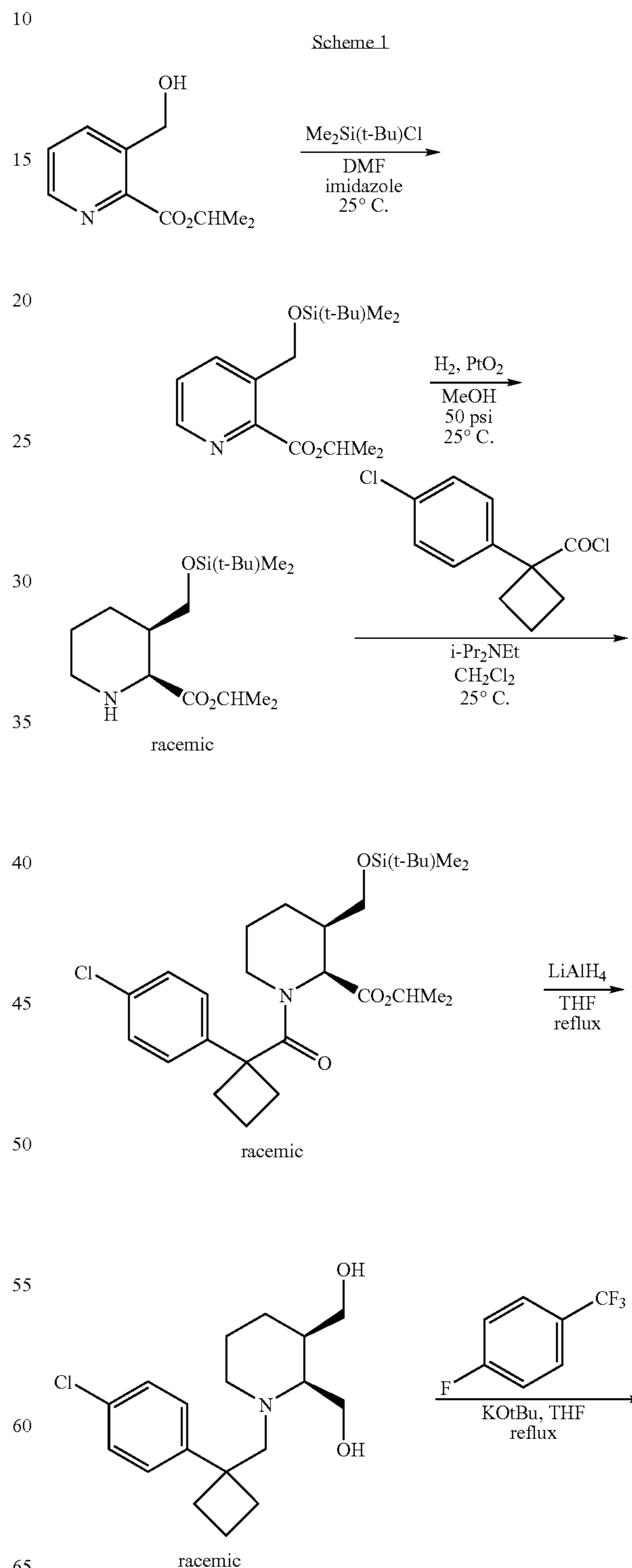
R-1-[1-(4-Chloro-phenyl)-cyclobutylmethyl]-3-(4-trifluoromethyl-benzyloxymethyl)-piperidine
