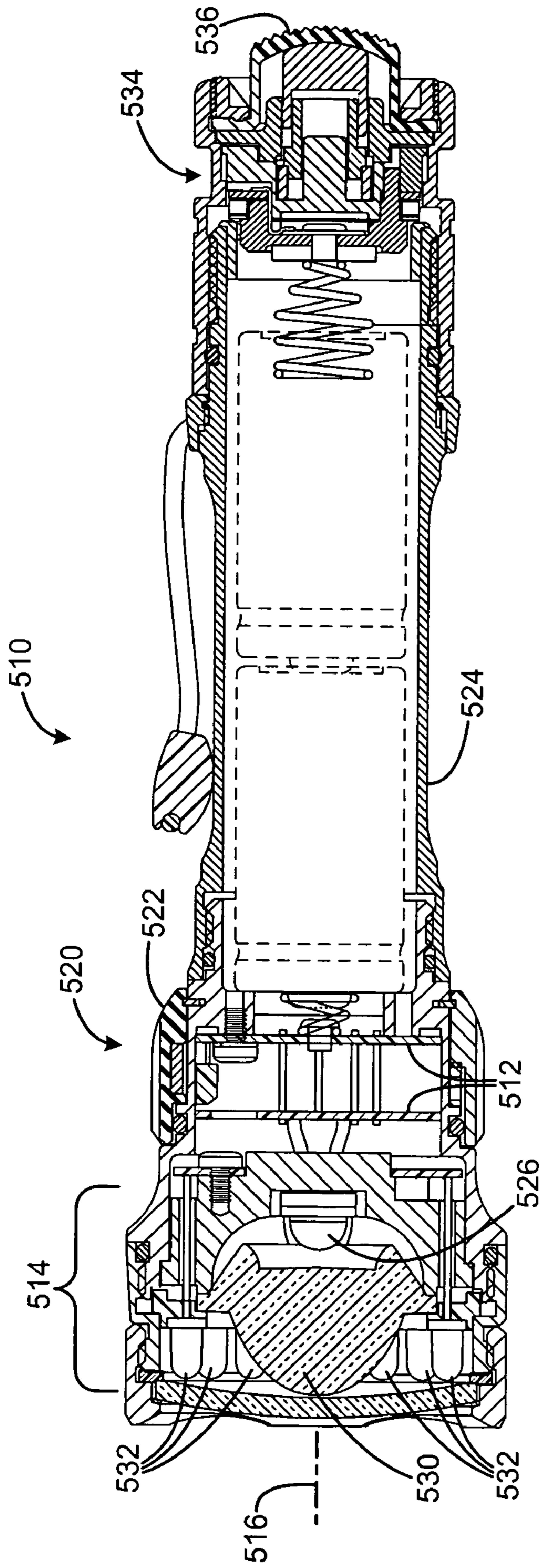
FIG. 14
