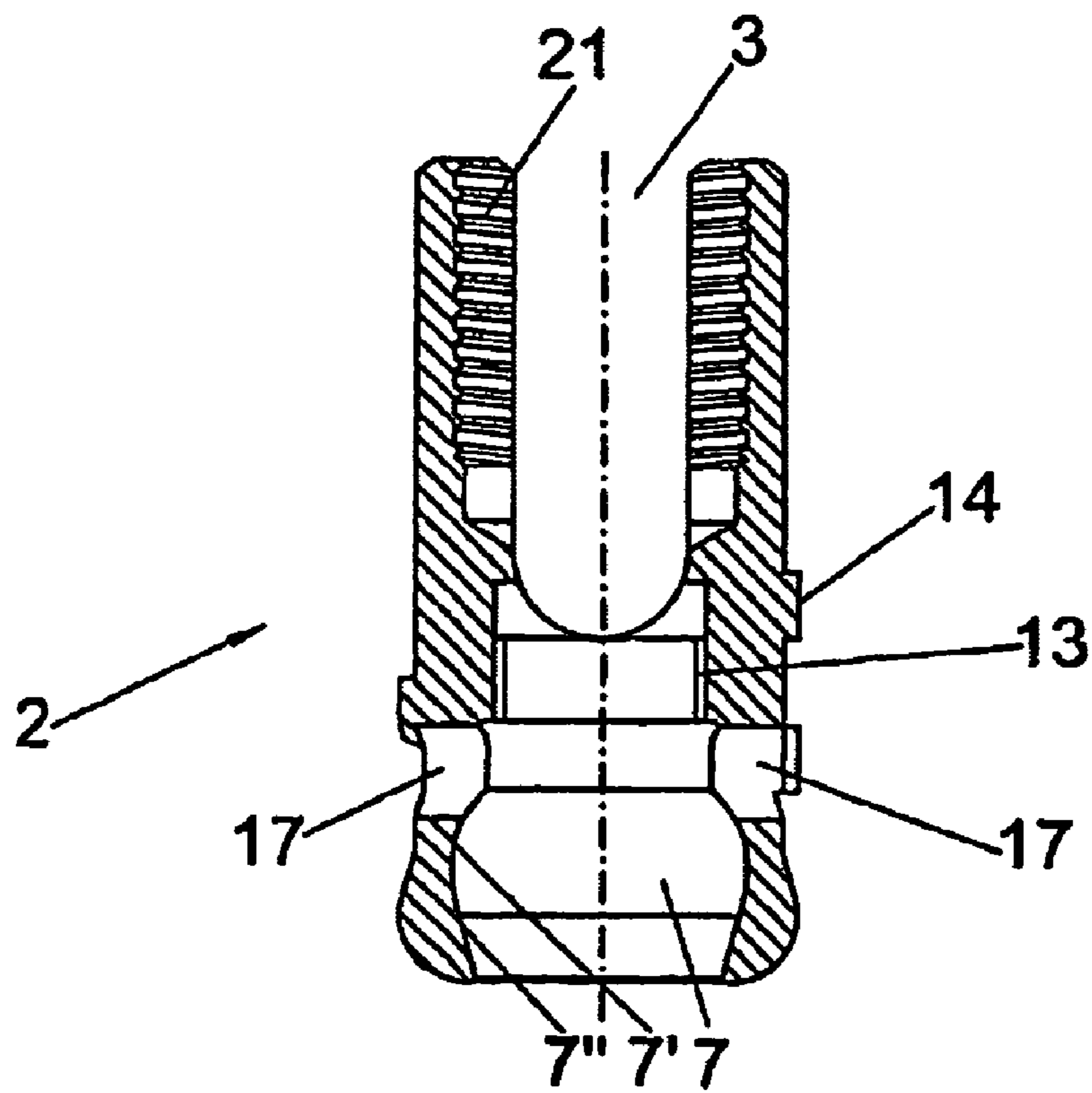
A-A FIG. 5
