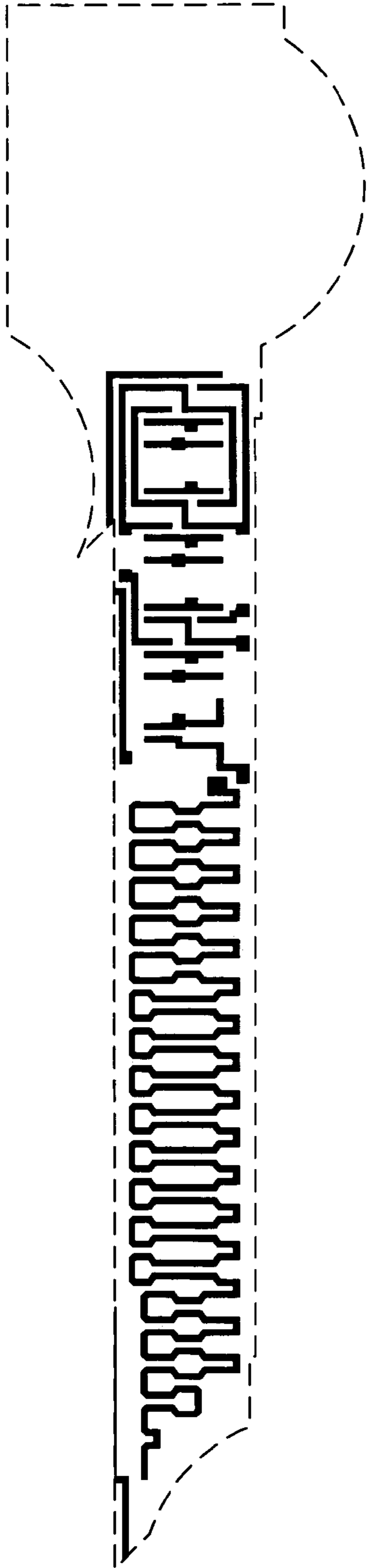
Poly mask
