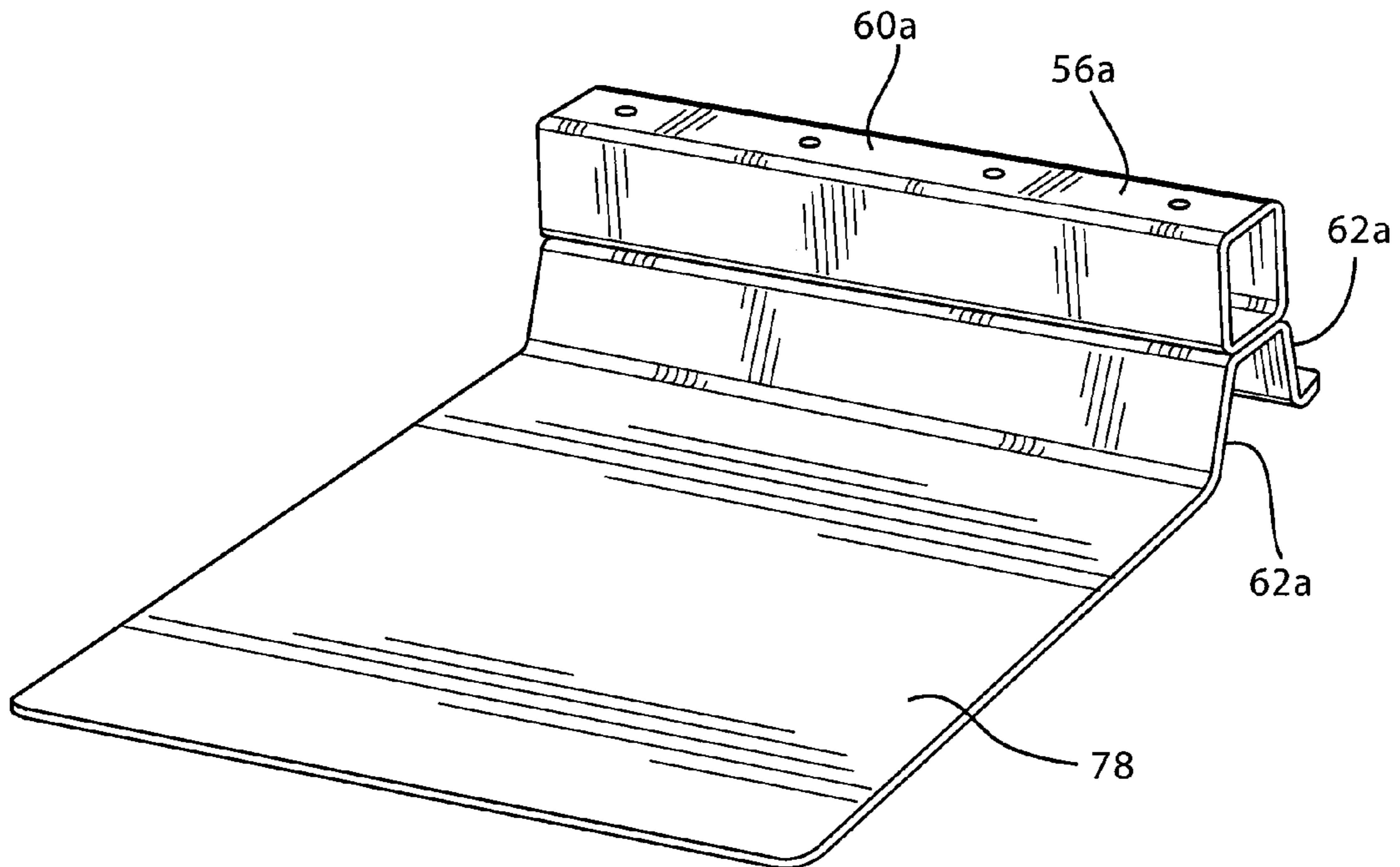
FIG. 9B
