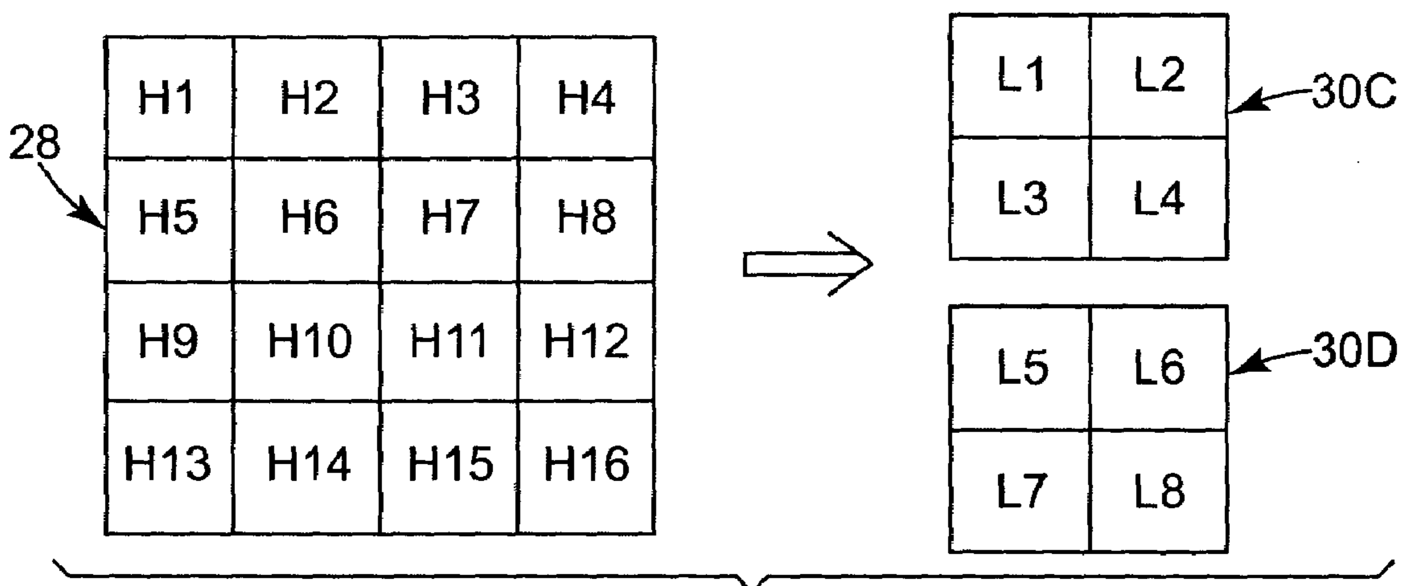
Fig. 6 (BILINEAR)
