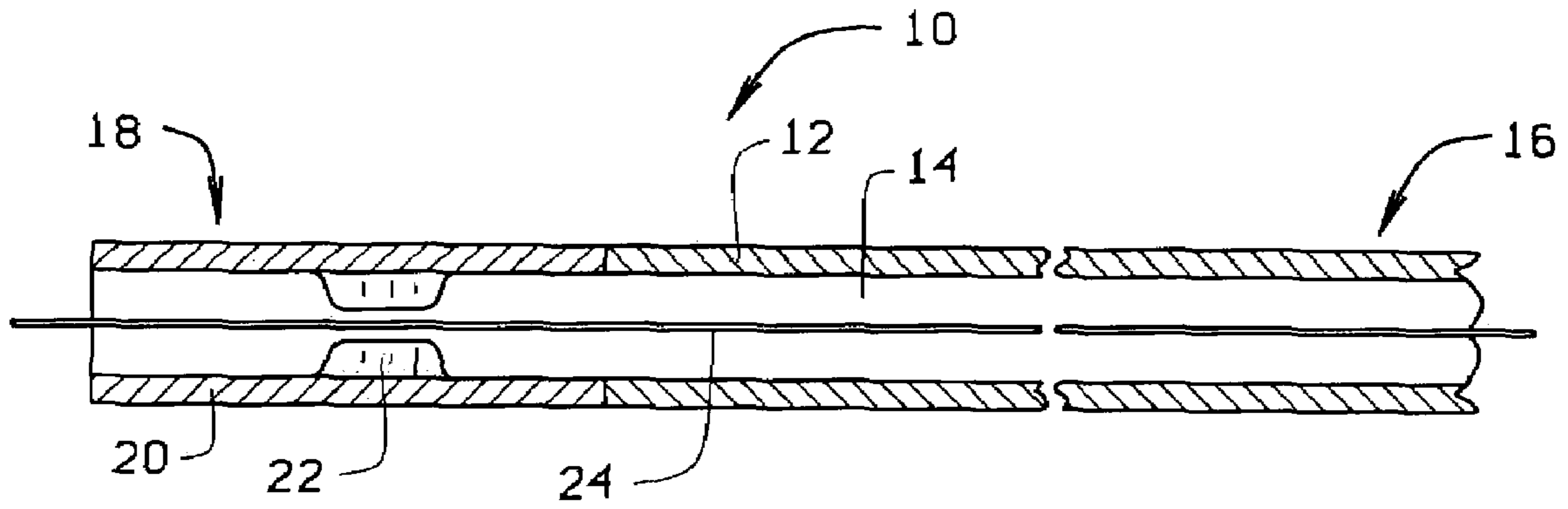
FIG. 1
