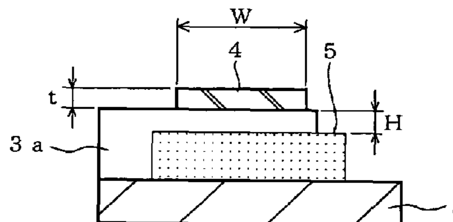
(y - y cross section)
