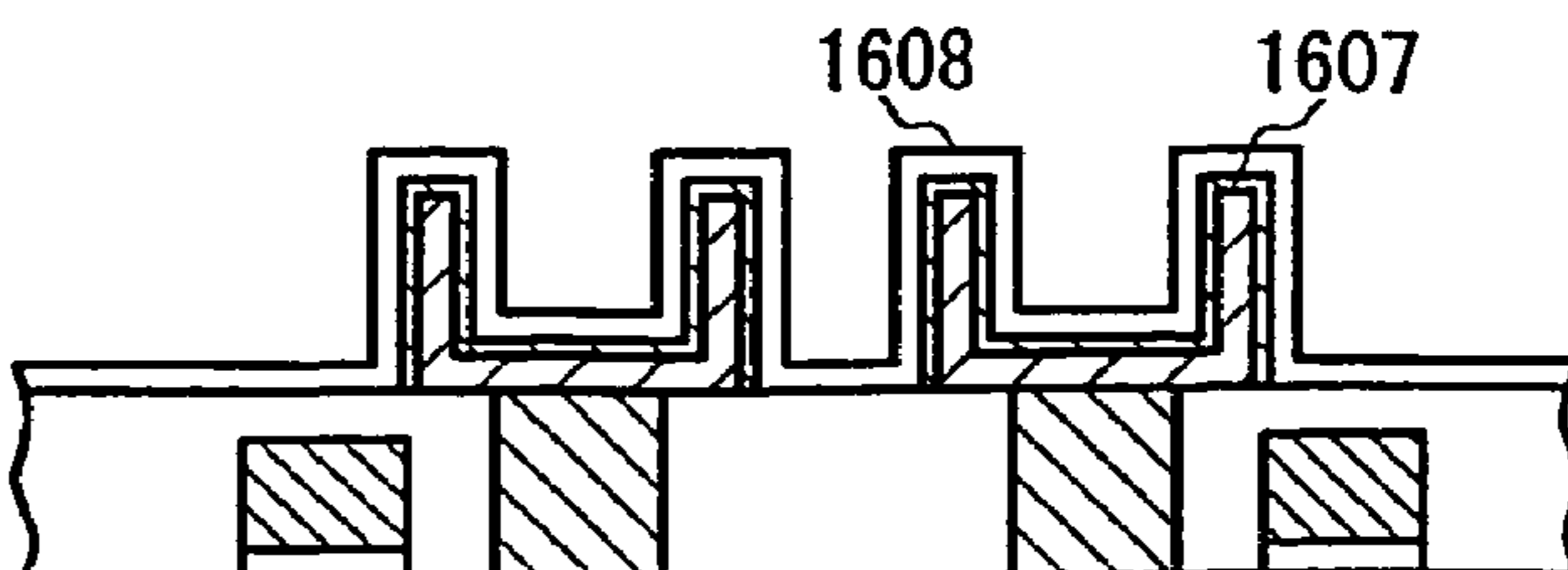
FIG. 16E PRIOR ART
