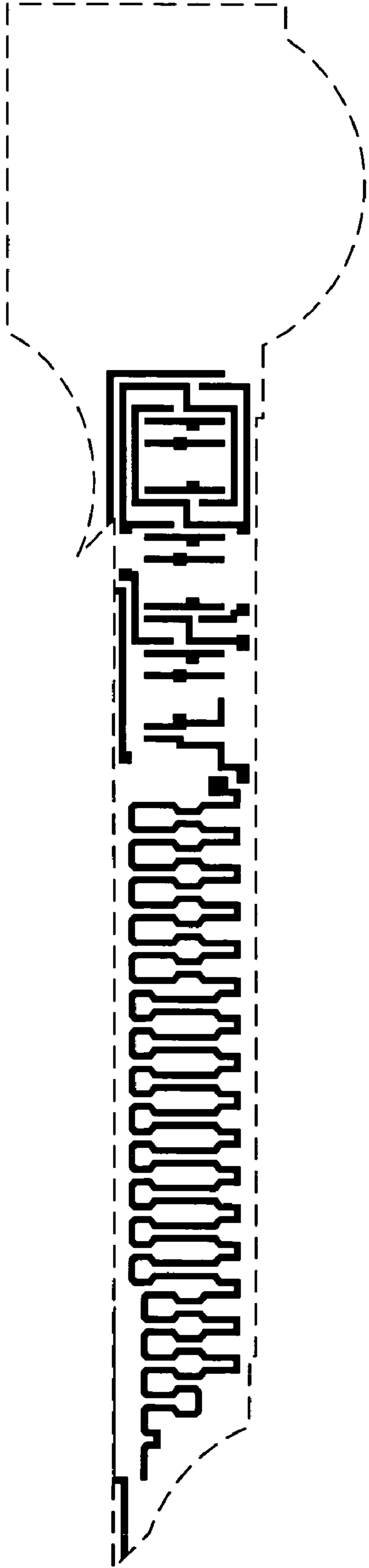
Poly mask
