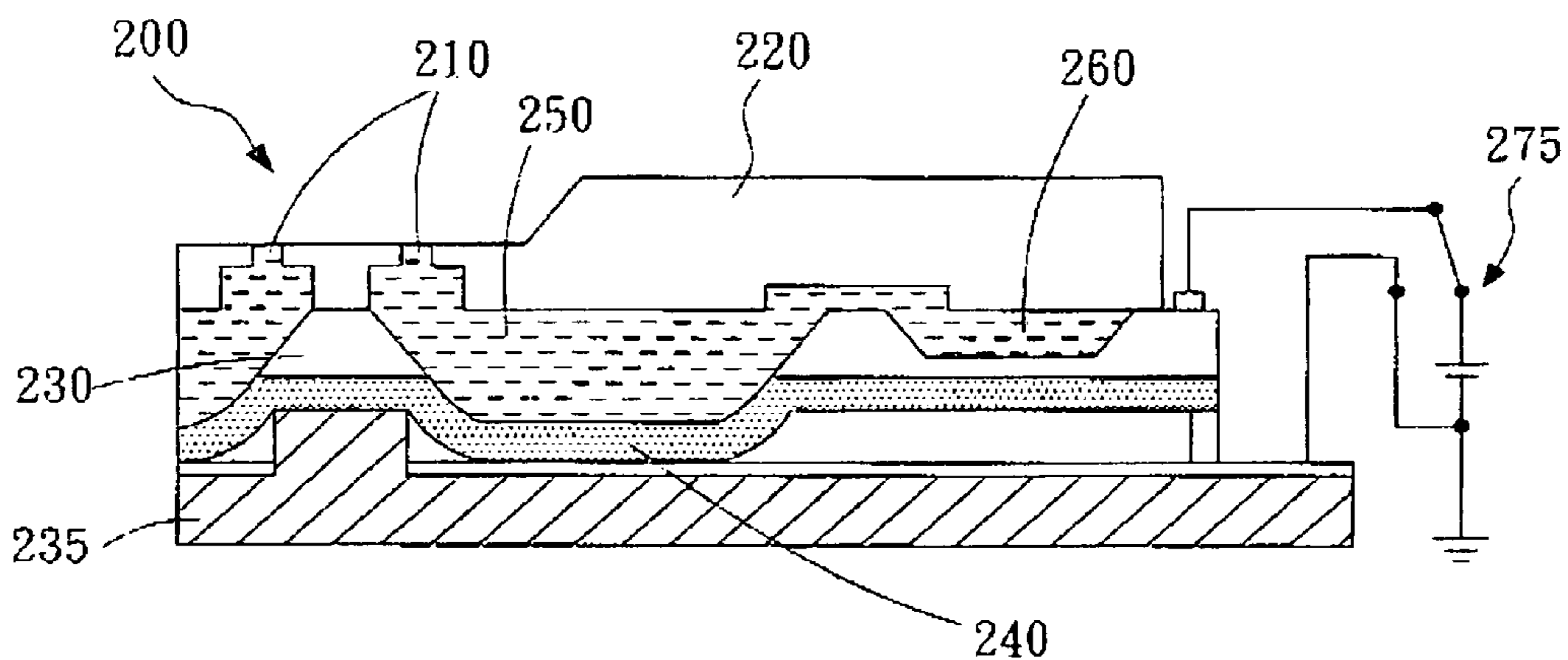
FIG. 2B(PRIOR ART)
