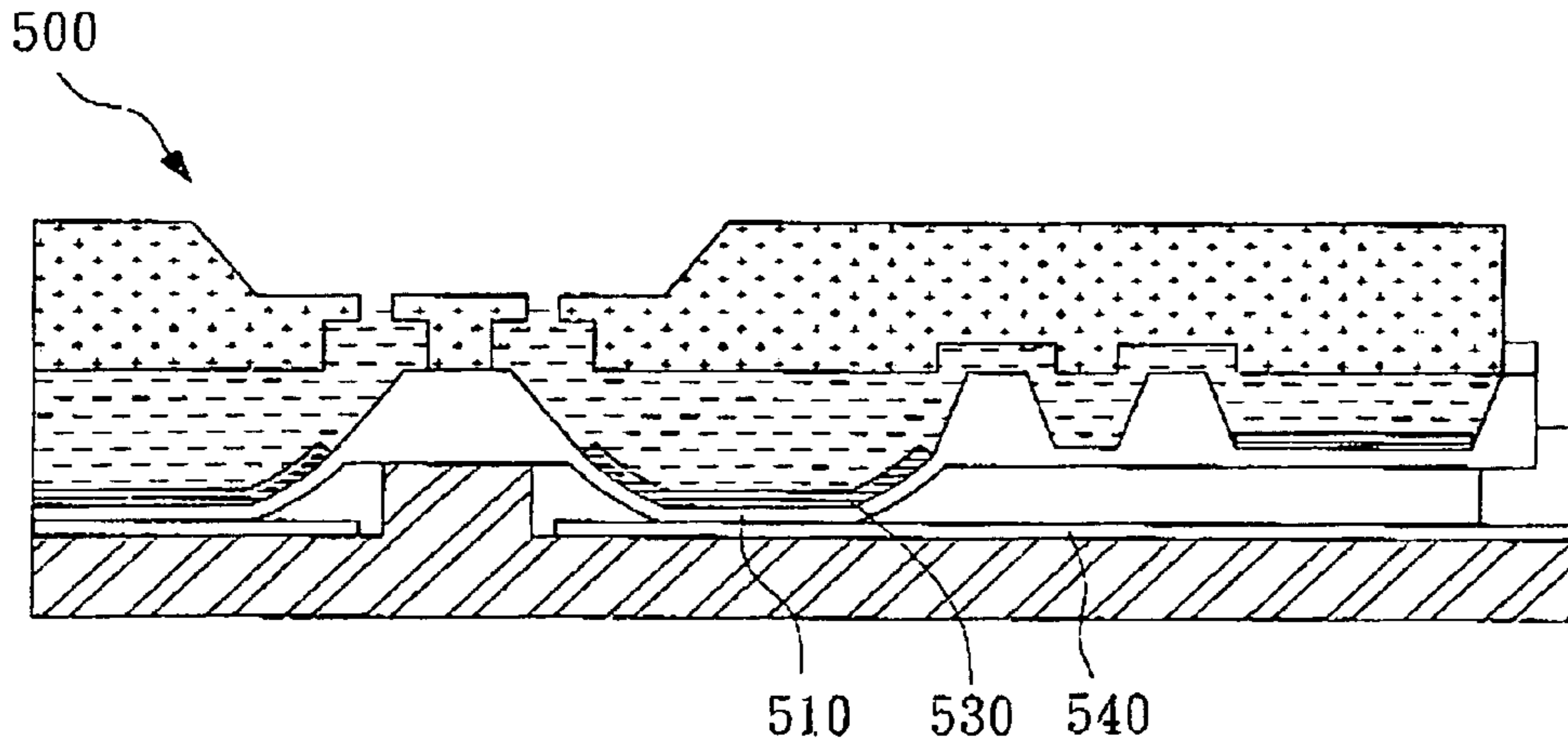
FIG. 5A
