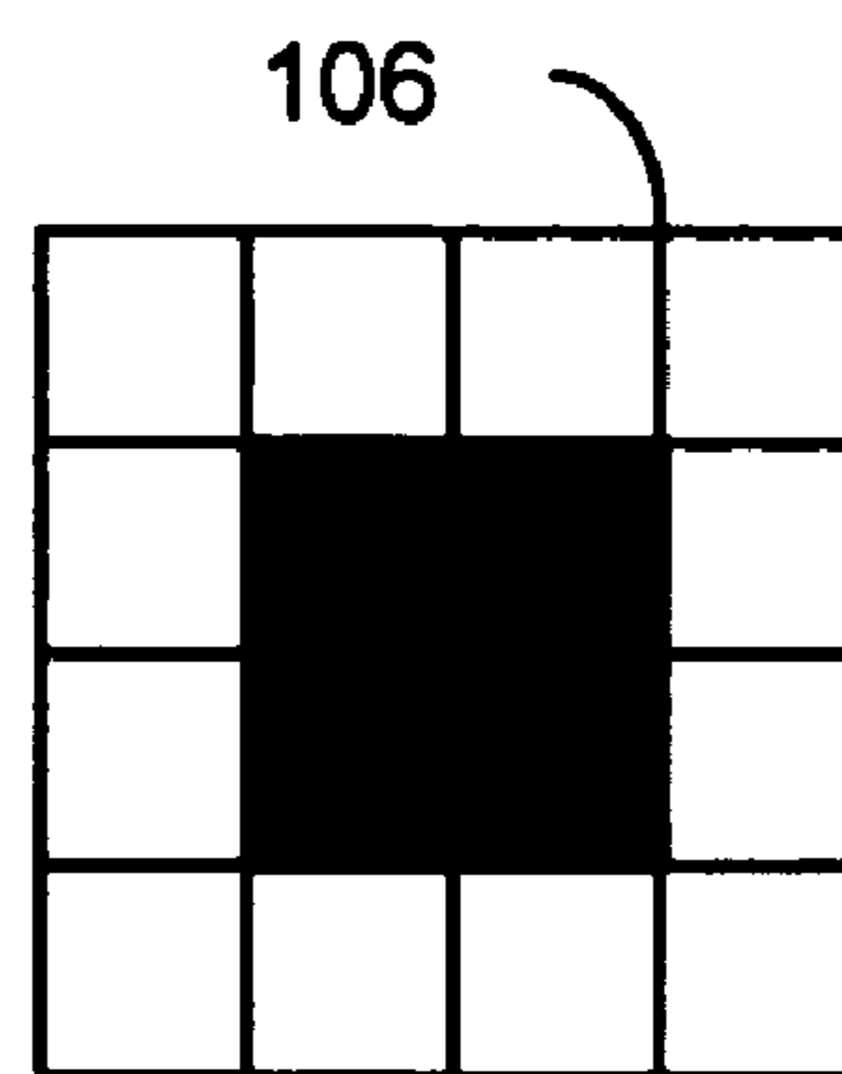
A-buffer
