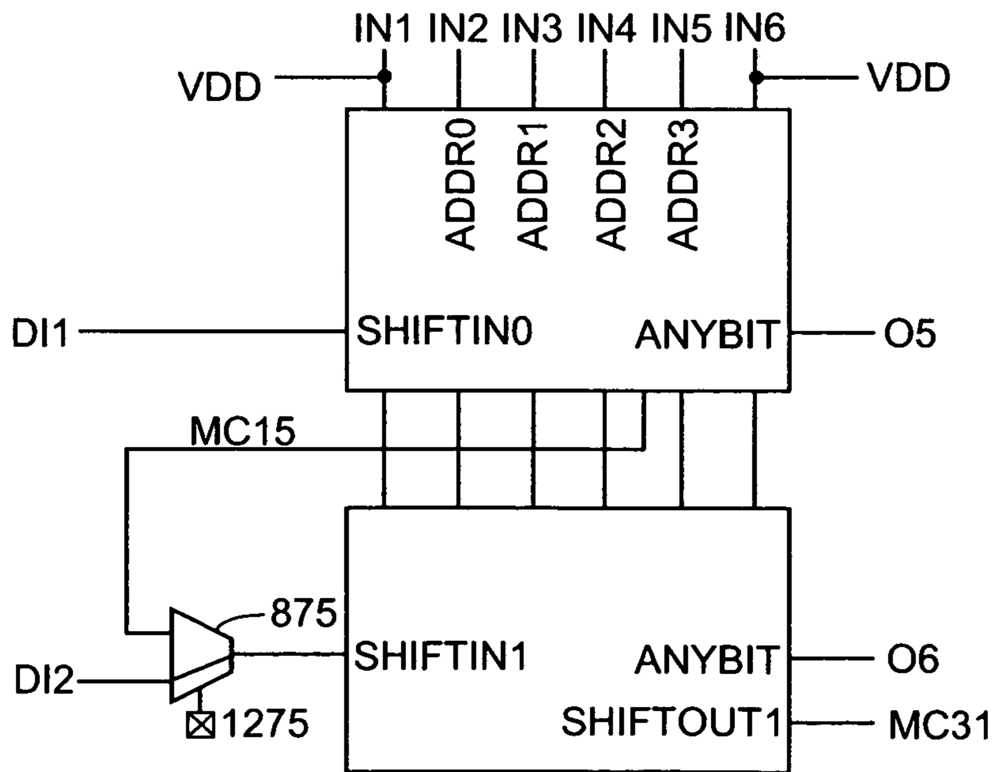
FIG. 13 (16x2 SRL)
