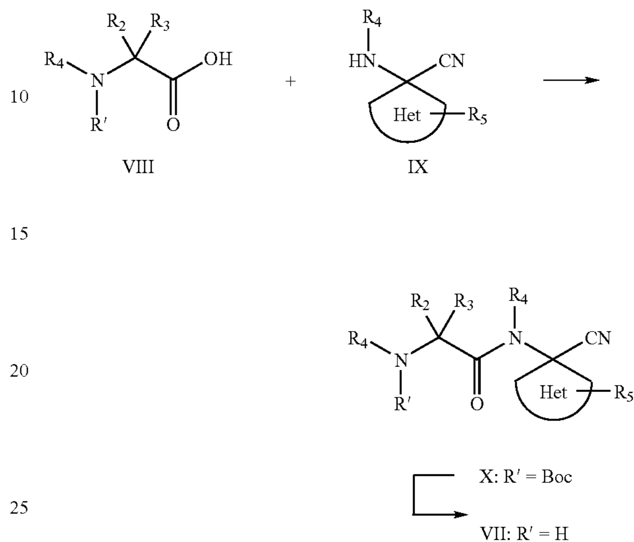
Scheme VI
