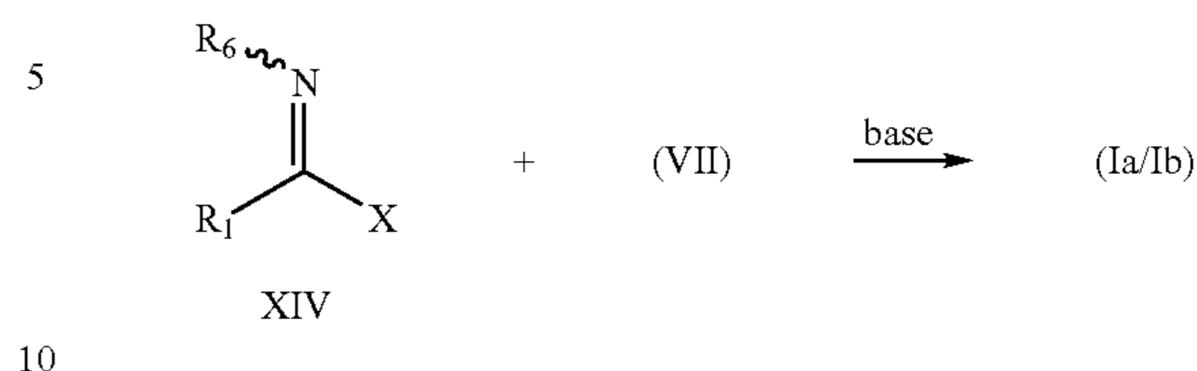
Scheme IX (Method G)
