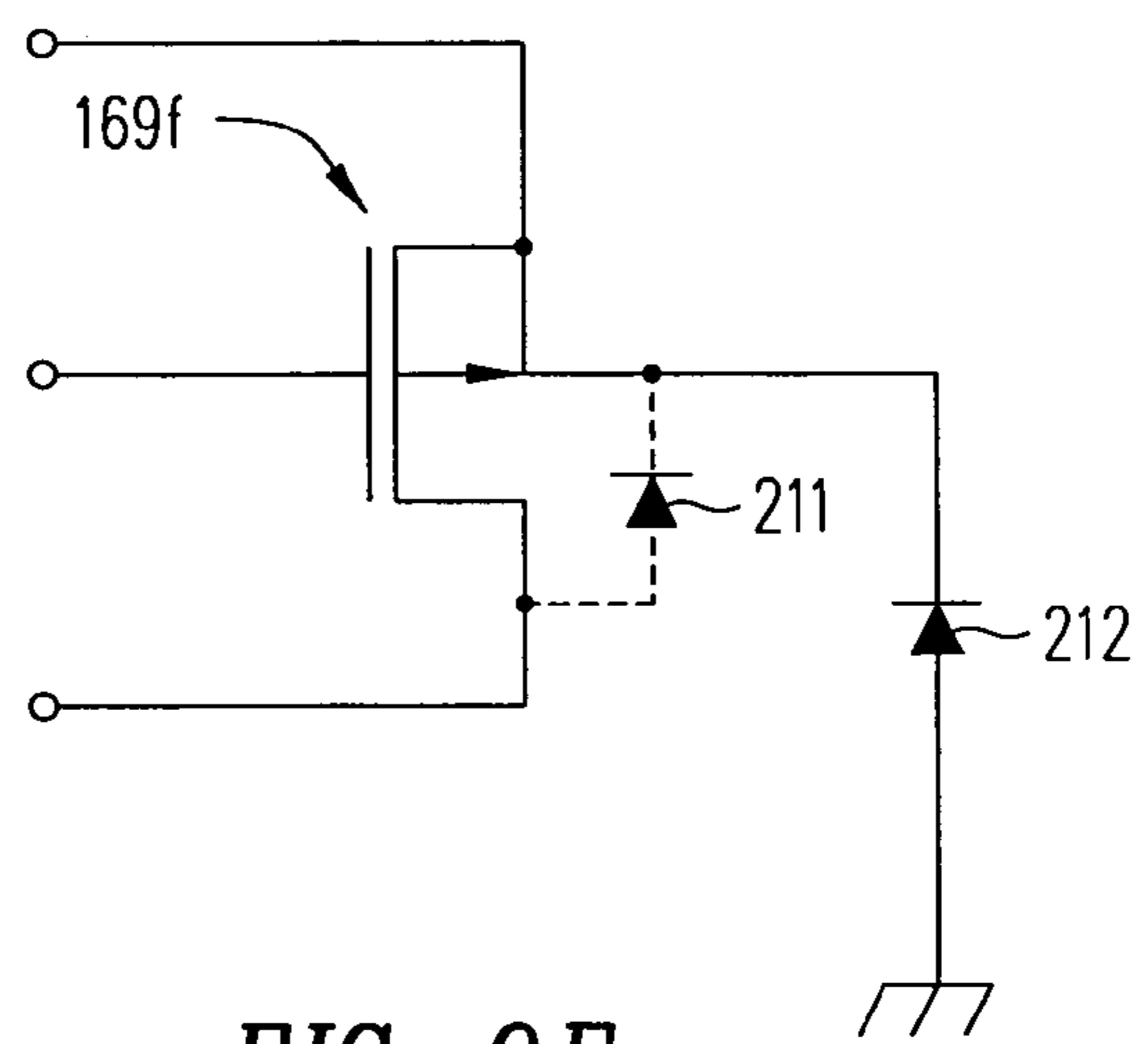
FIG. 9F
