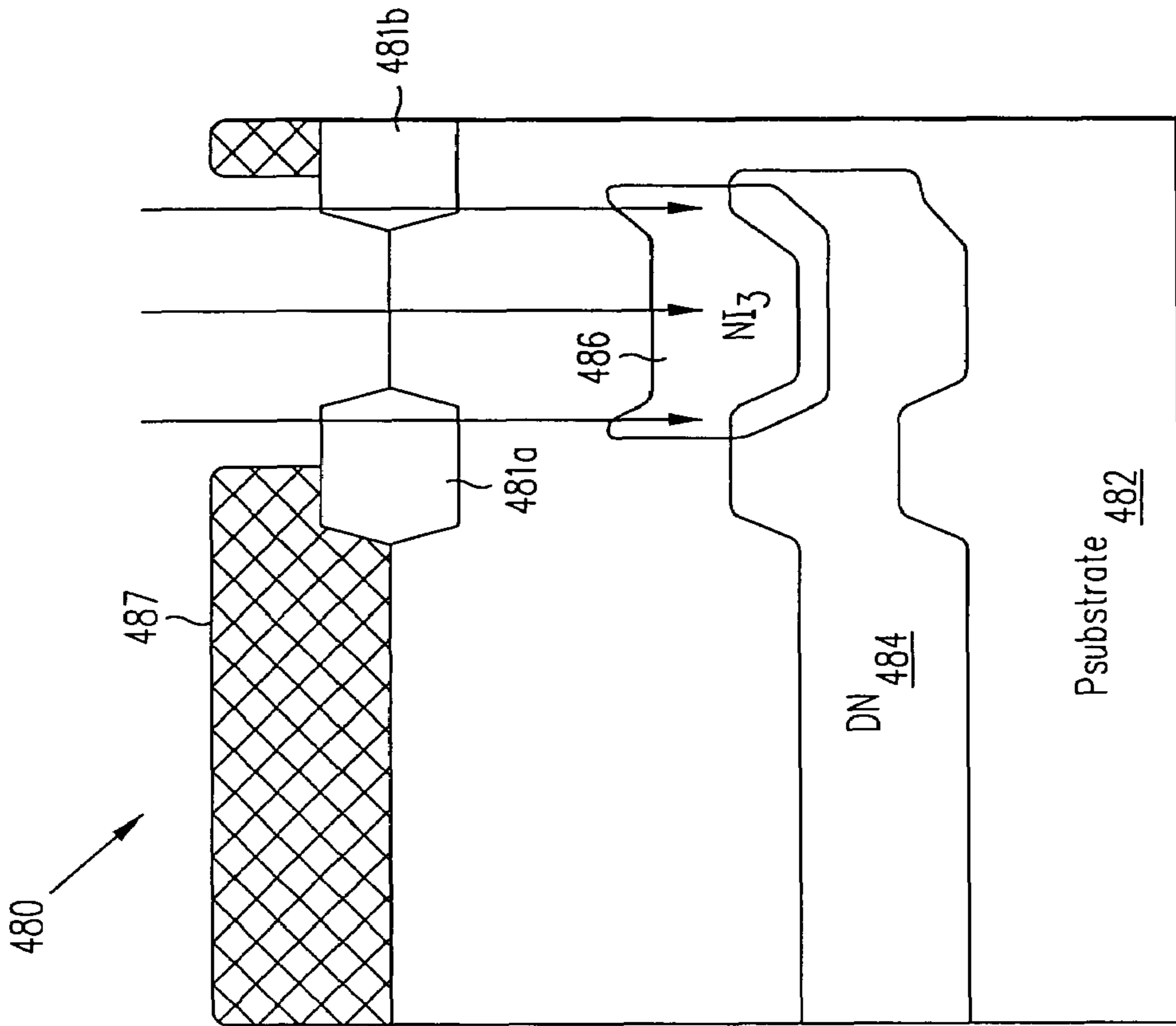
FIG. 20B
