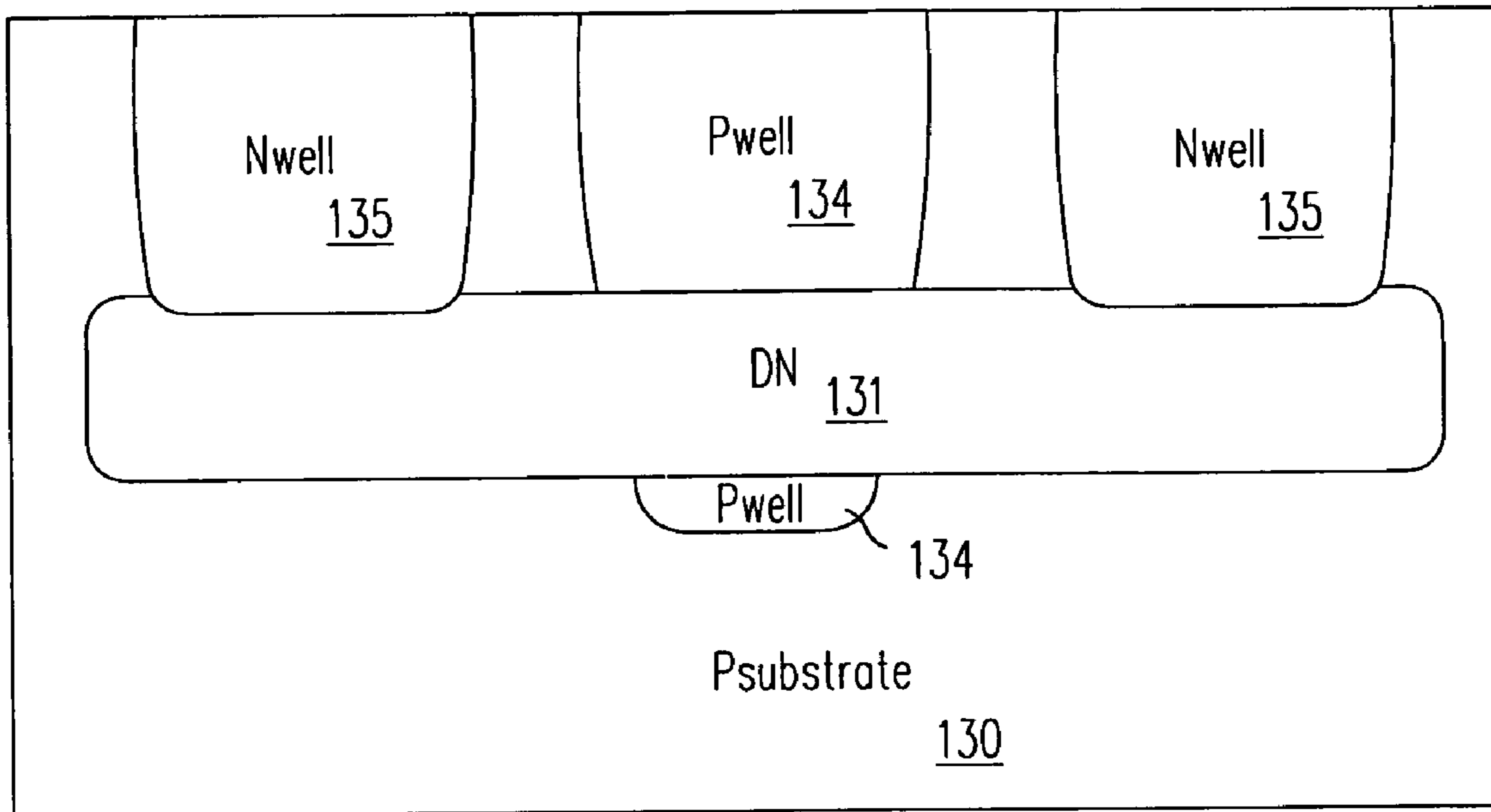
FIG. 6M
