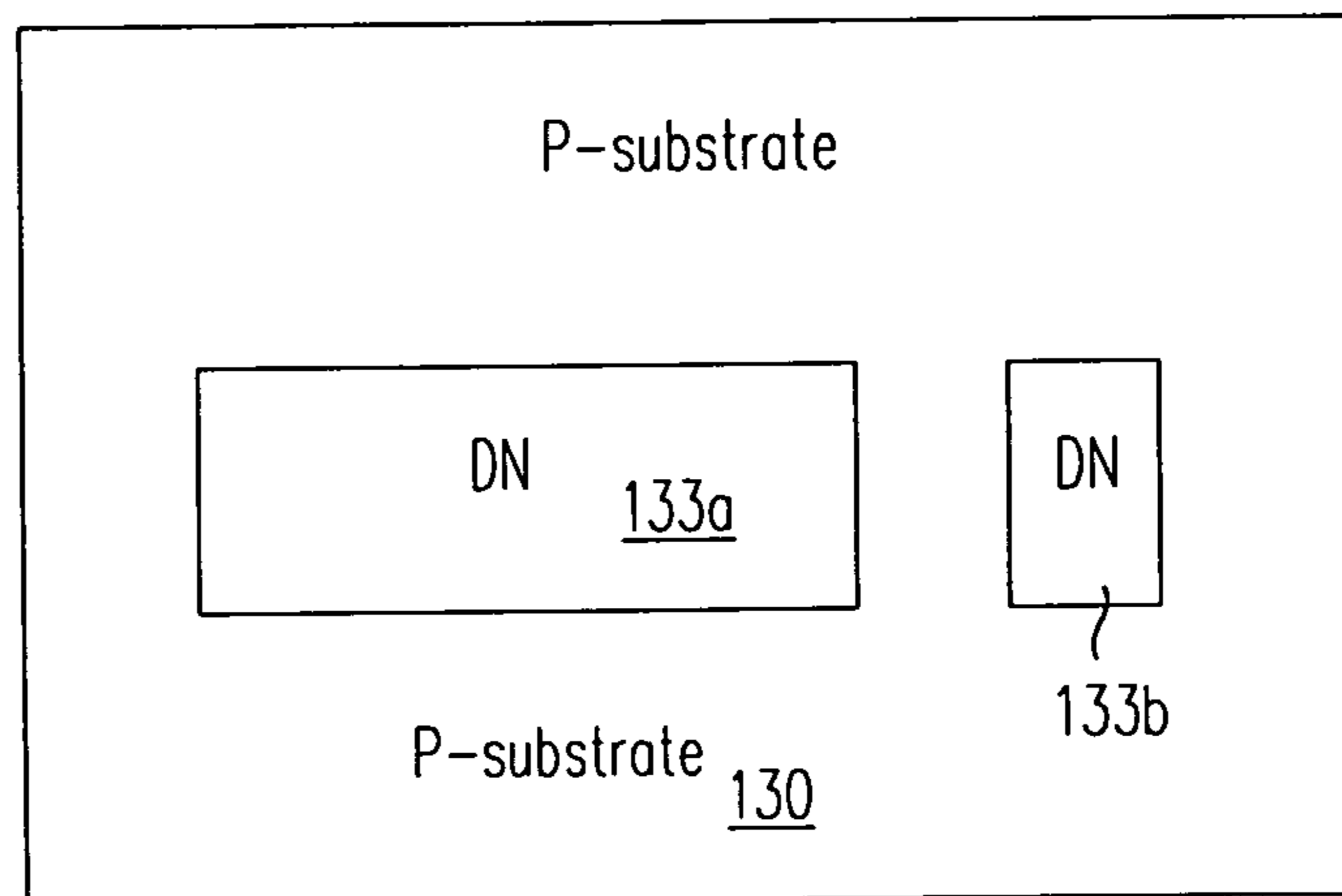
FIG. 6B
