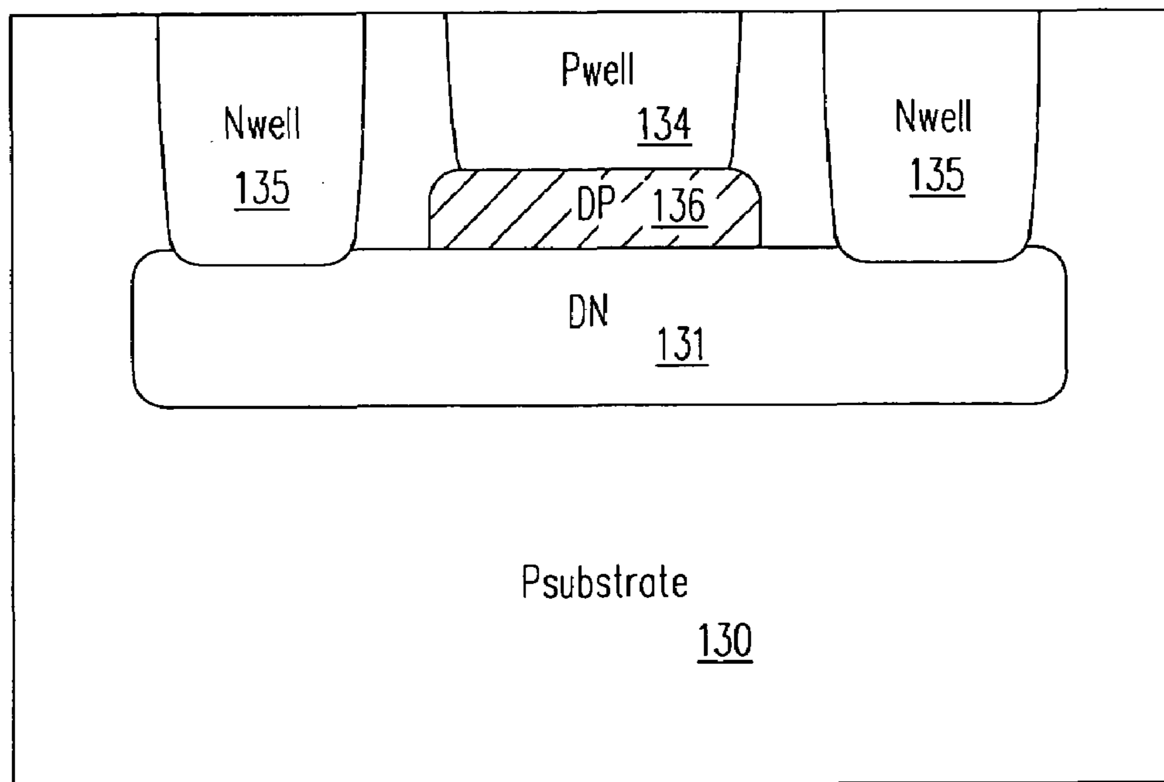
FIG. 6V
