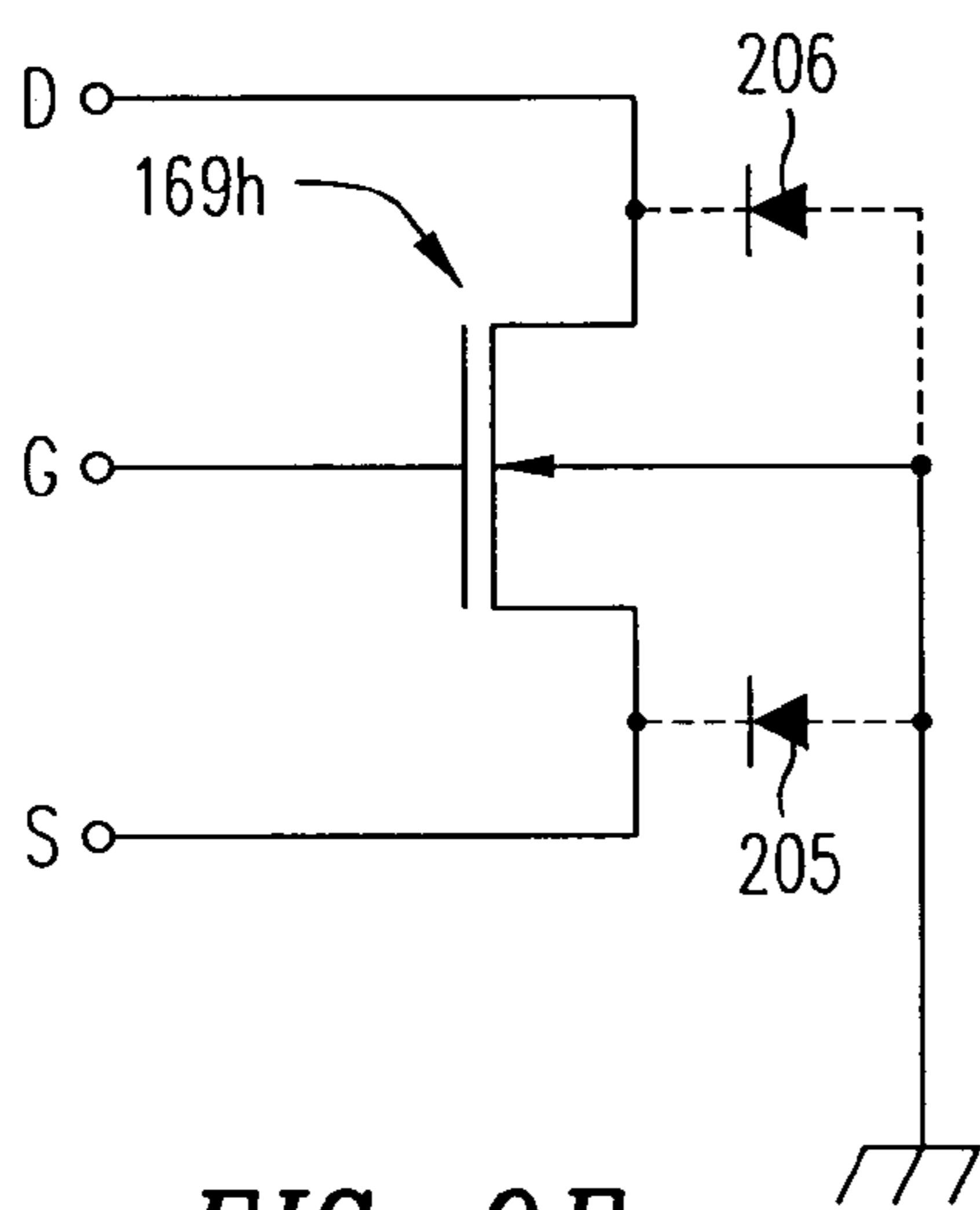
FIG. 9E
