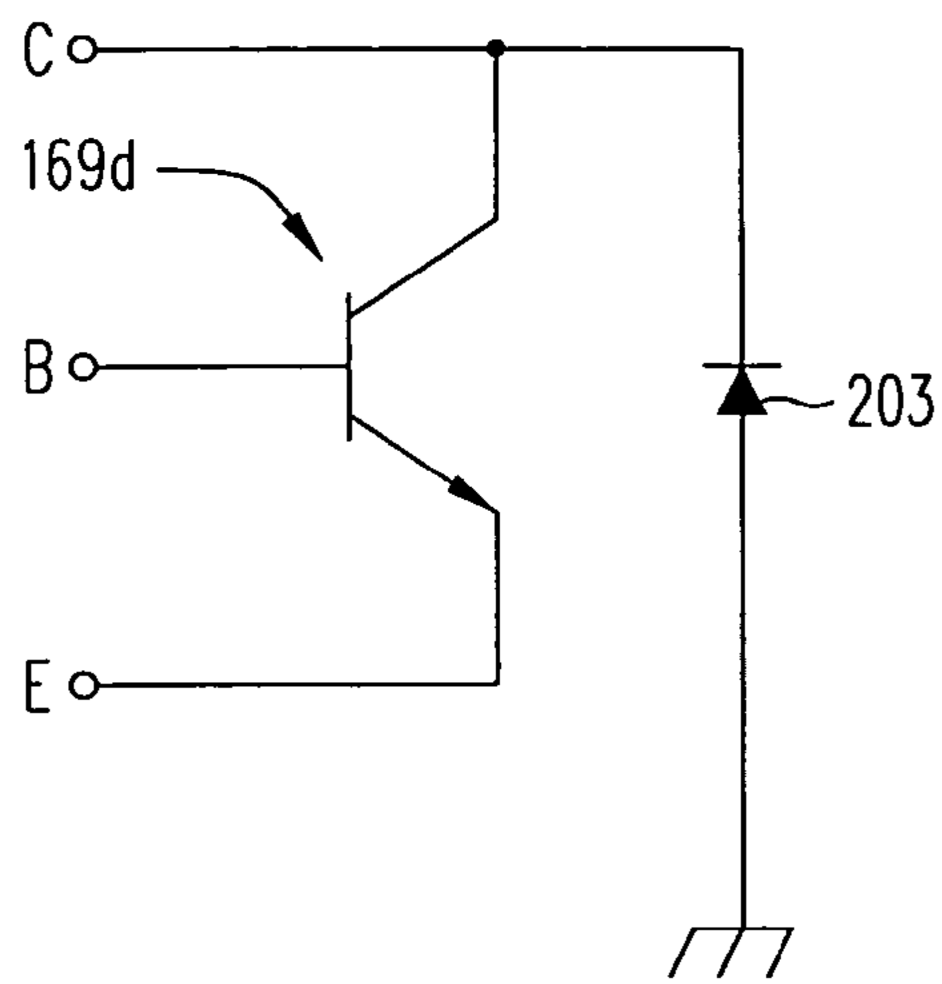
FIG. 9C
