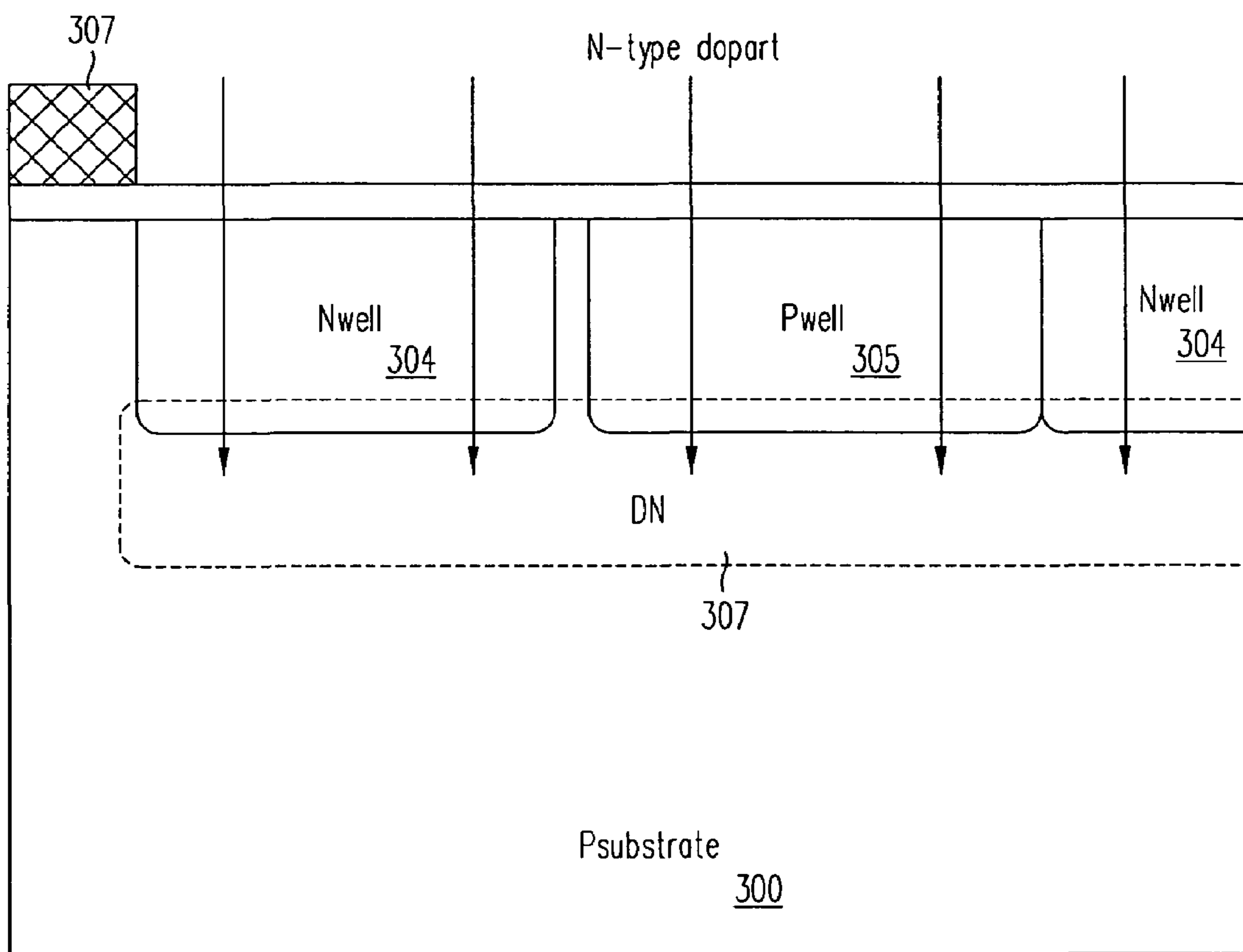
FIG. 14G
