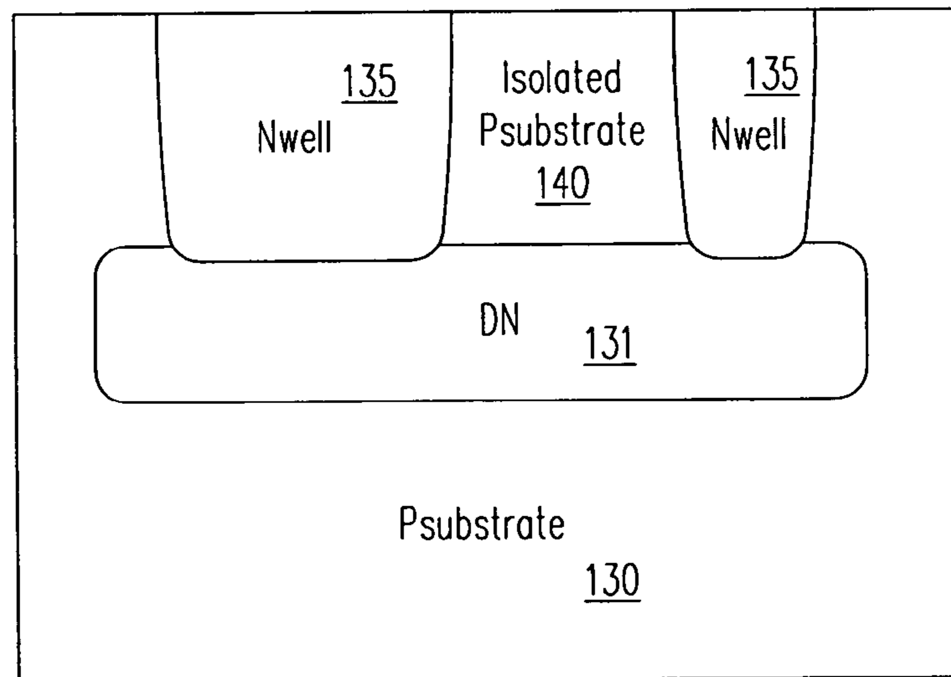
FIG. 6H
