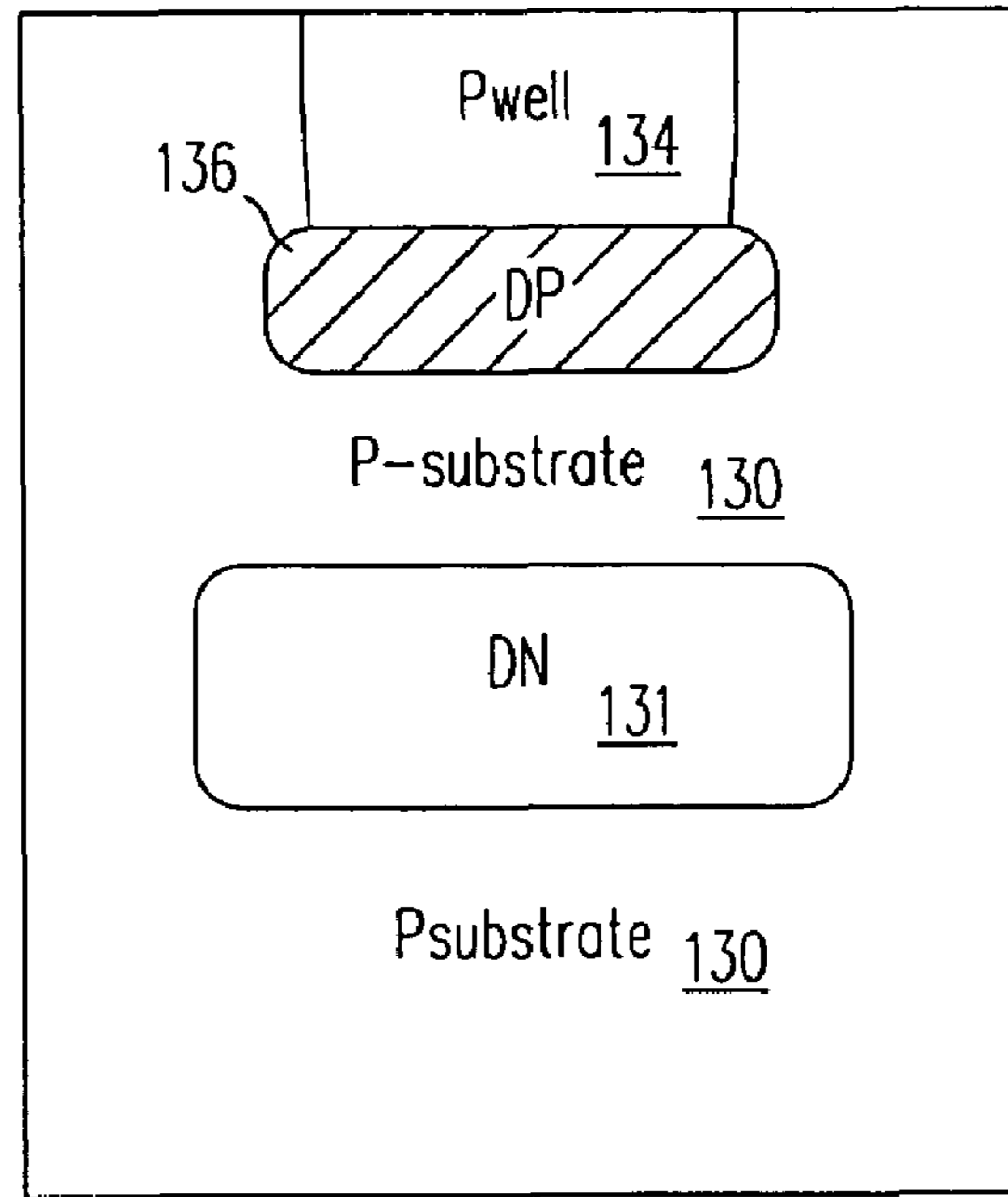
FIG. 6U
