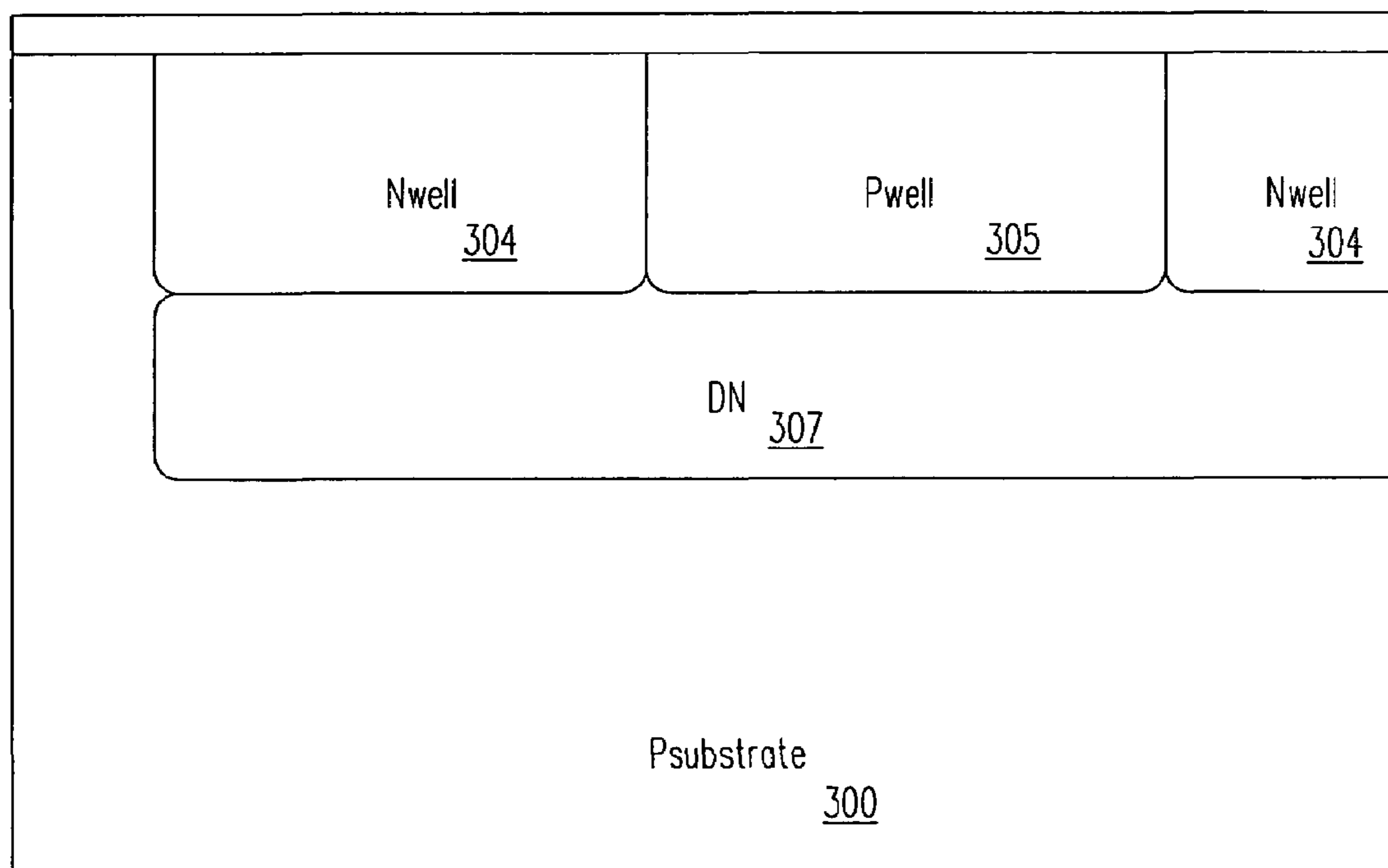
FIG. 14H
