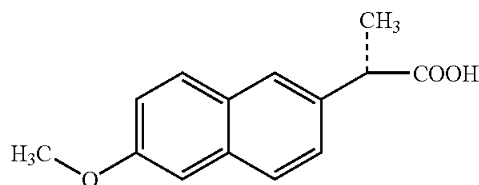
Naproxen
