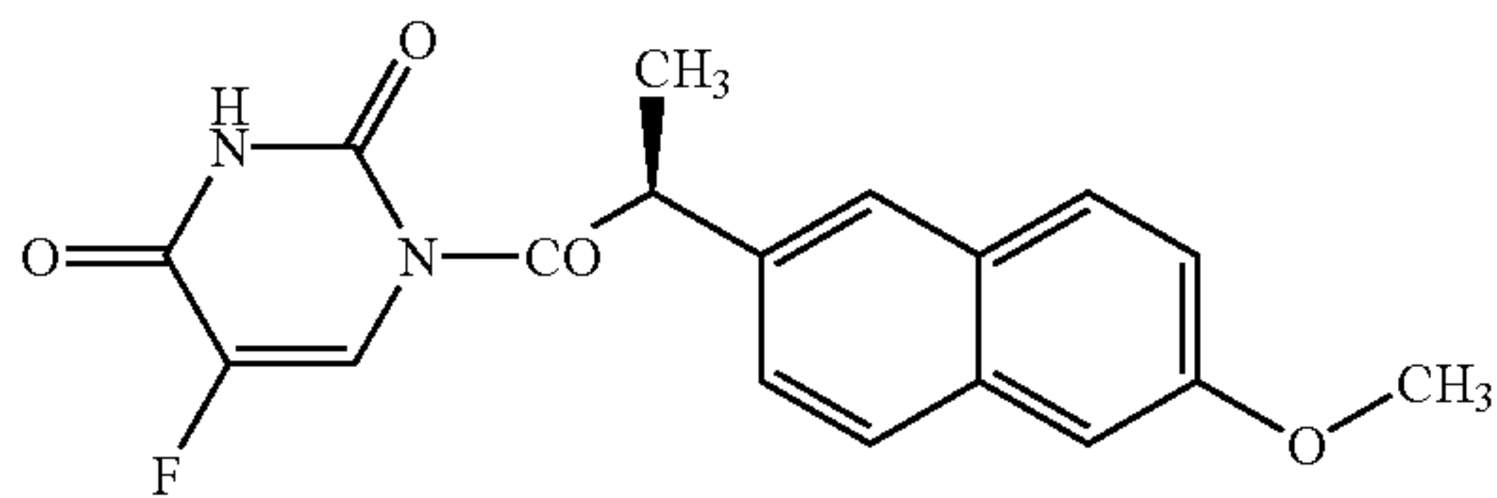
5FU-Naproxen
