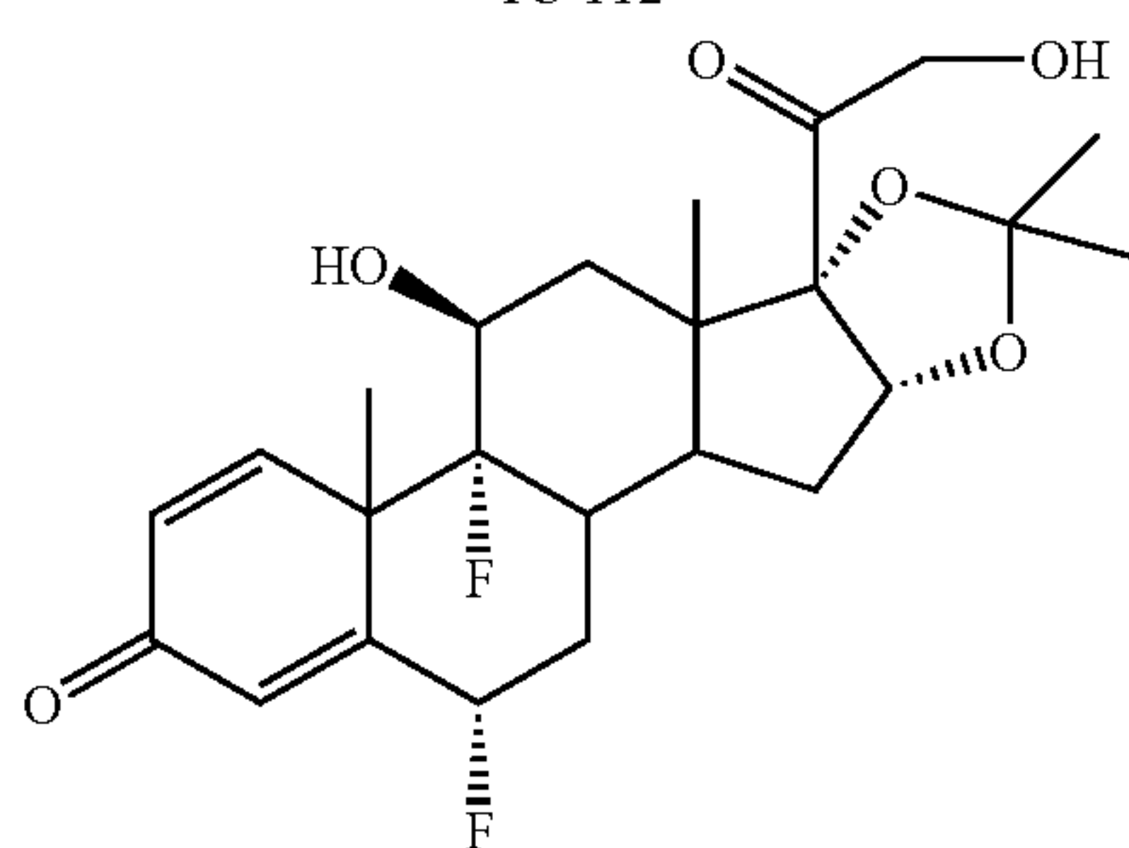
Flucinolone acetonide
