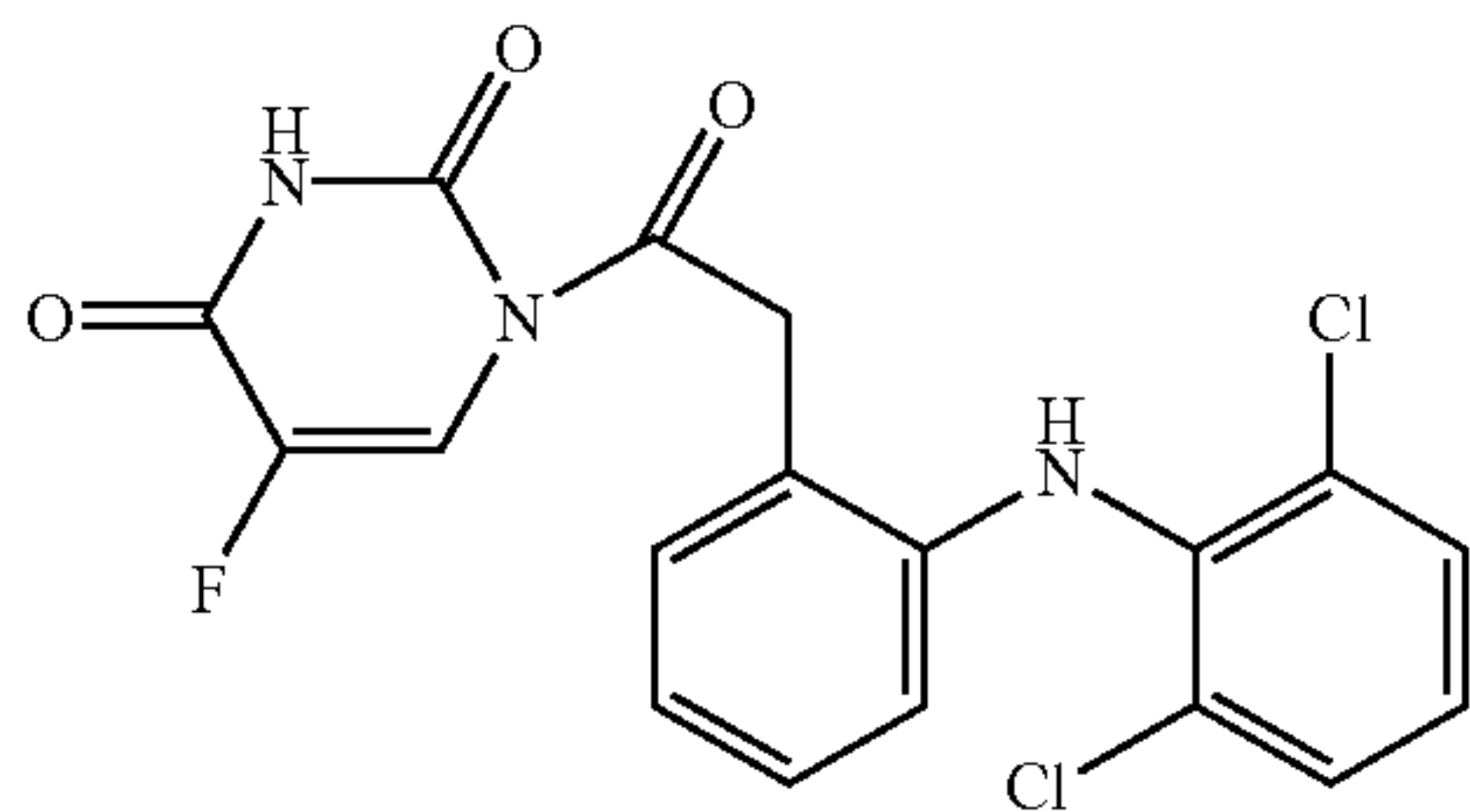
5FU-Diclofenac
