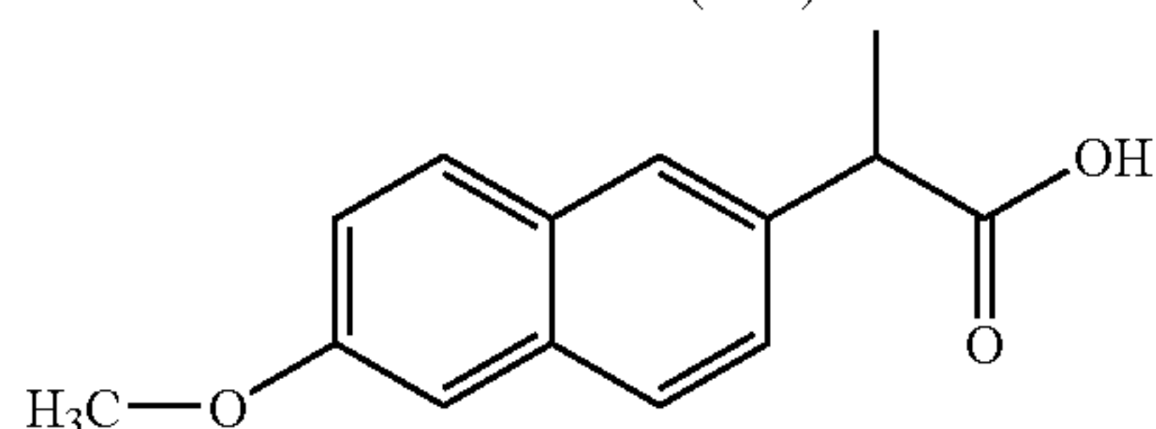
Naproxen
