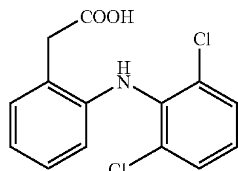
Diclofenac
