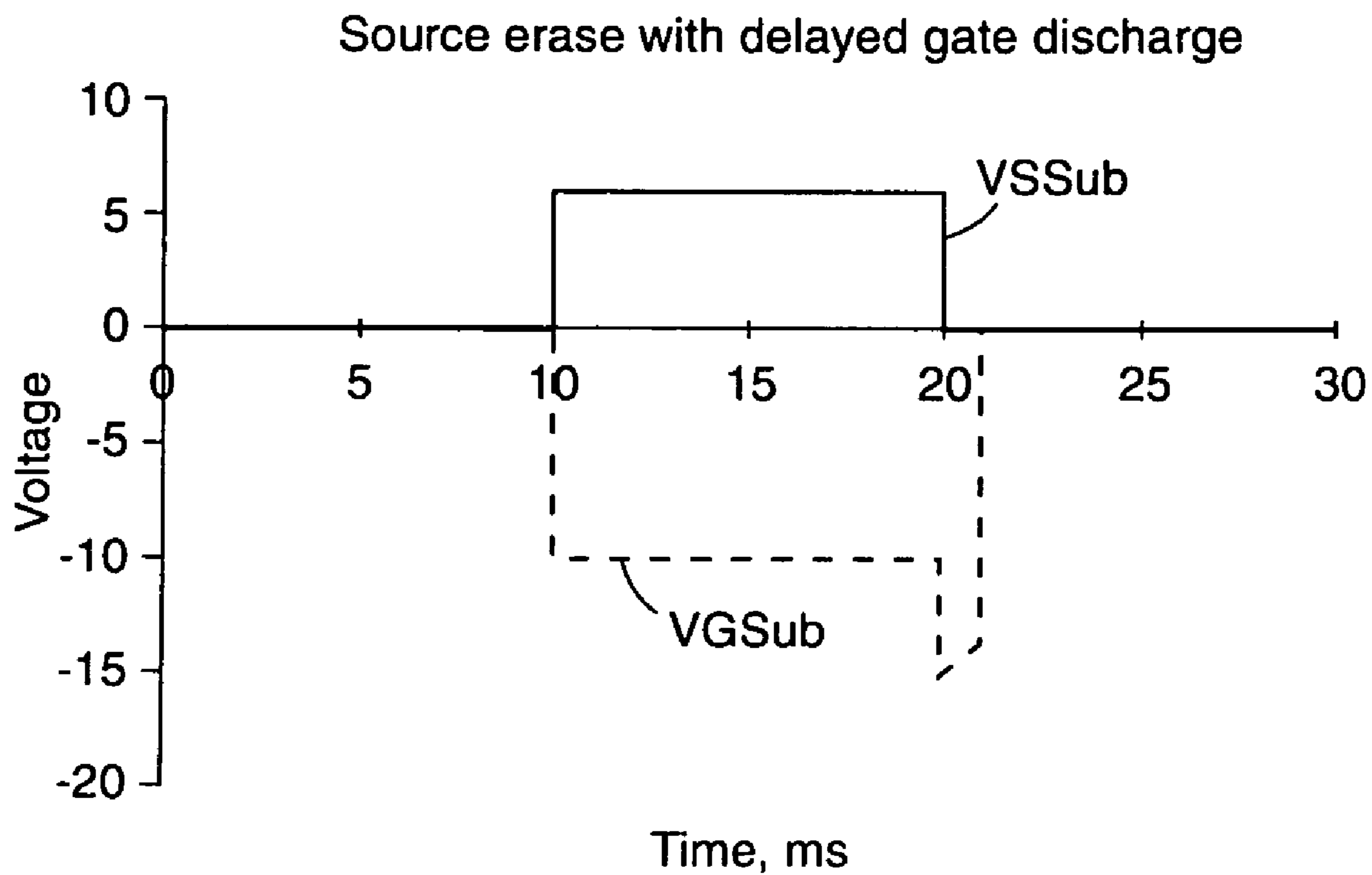
Fig. 7A
