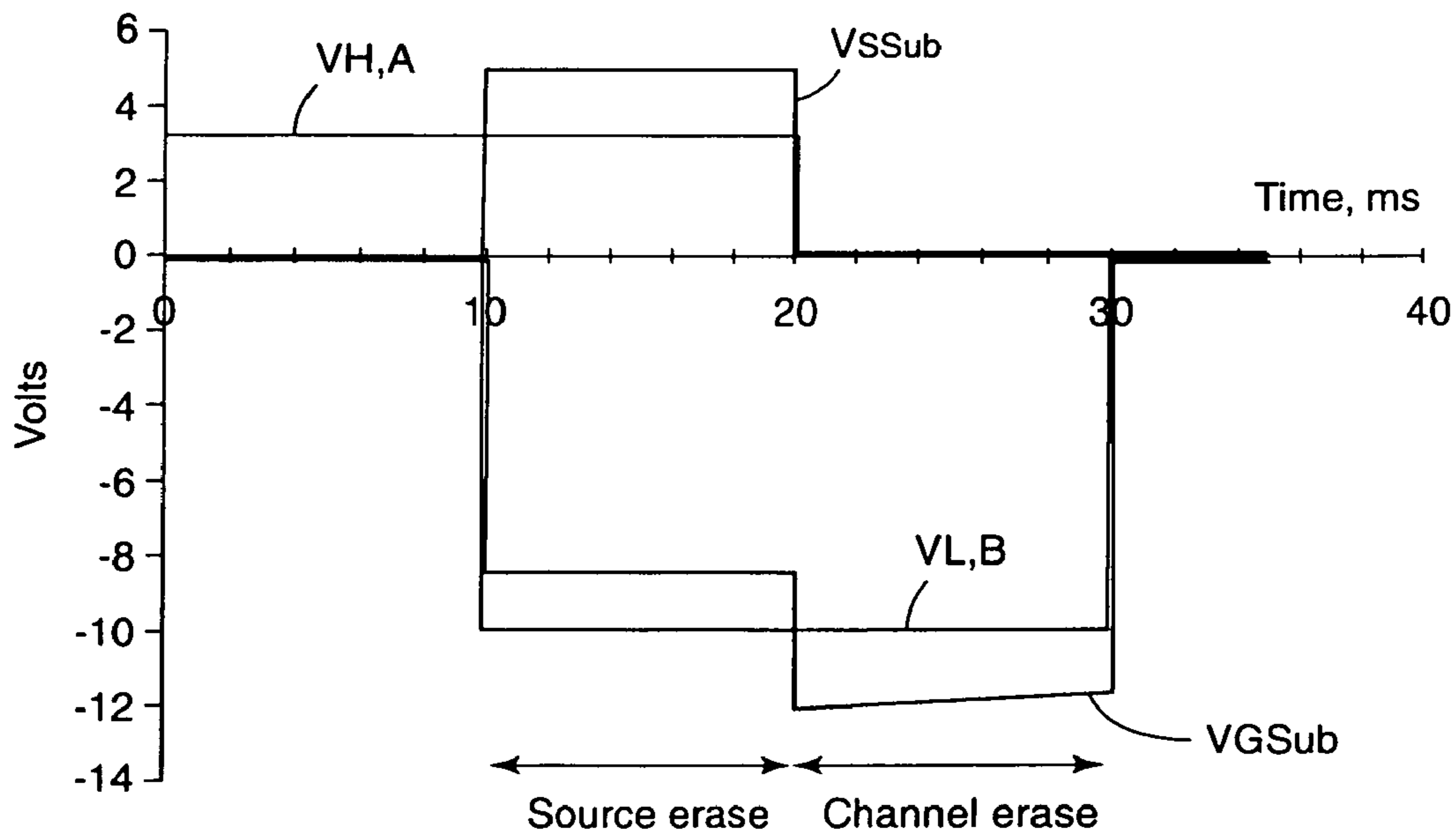
Fig. 7C
