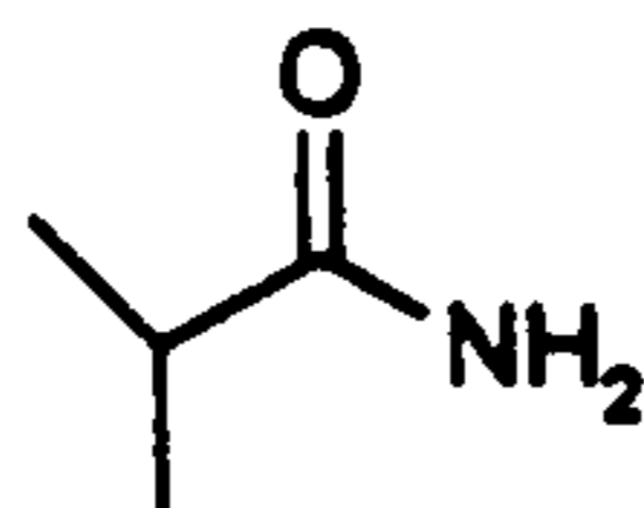
isobutyramide
