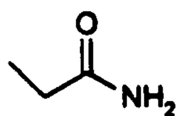
propionamide
