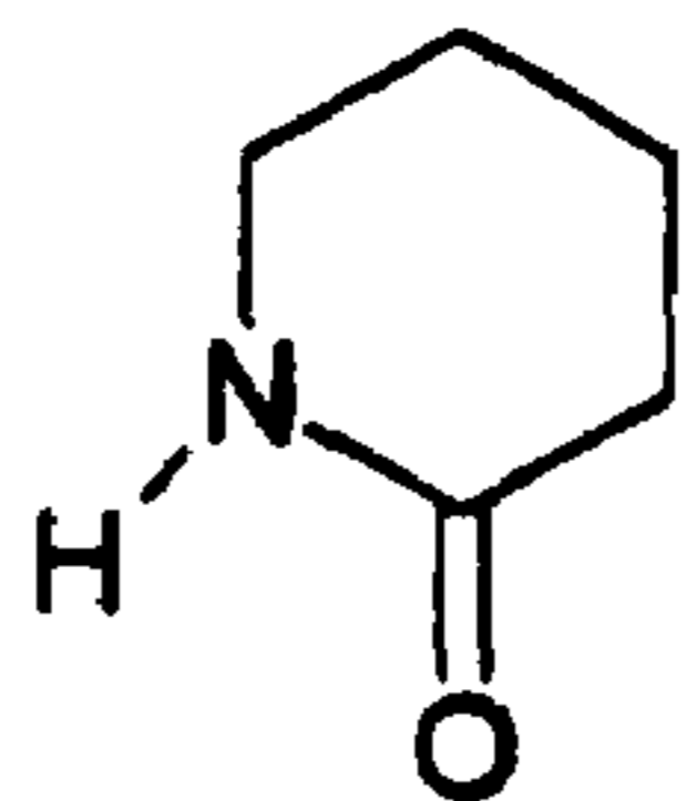
\delta -Valerolactam
