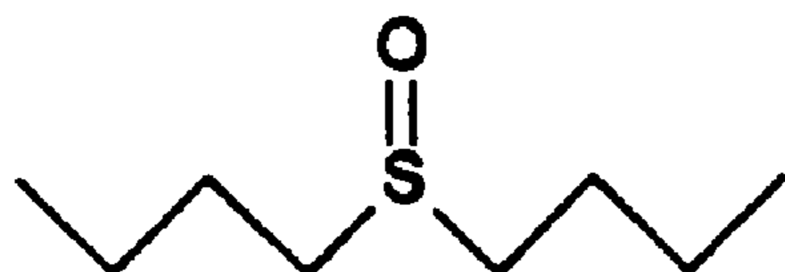
n-Butyl sulfoxide
