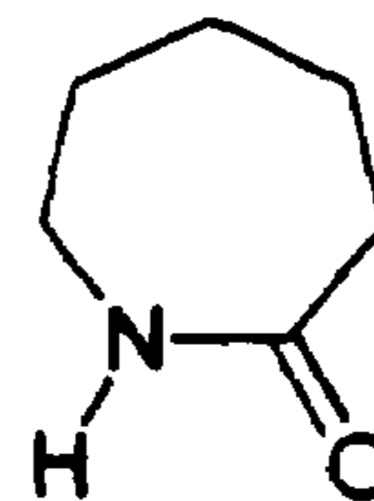
\epsilon -Caprolactam
