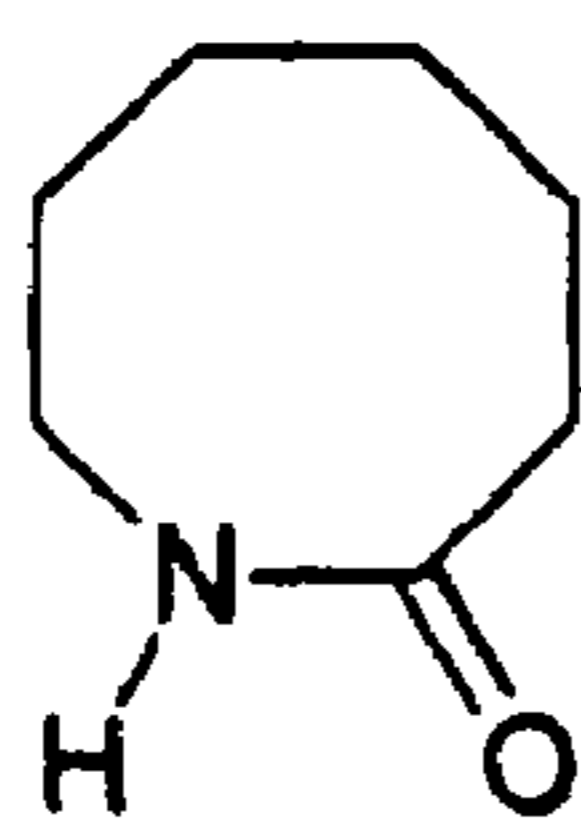
2-Azacyclooctanone
