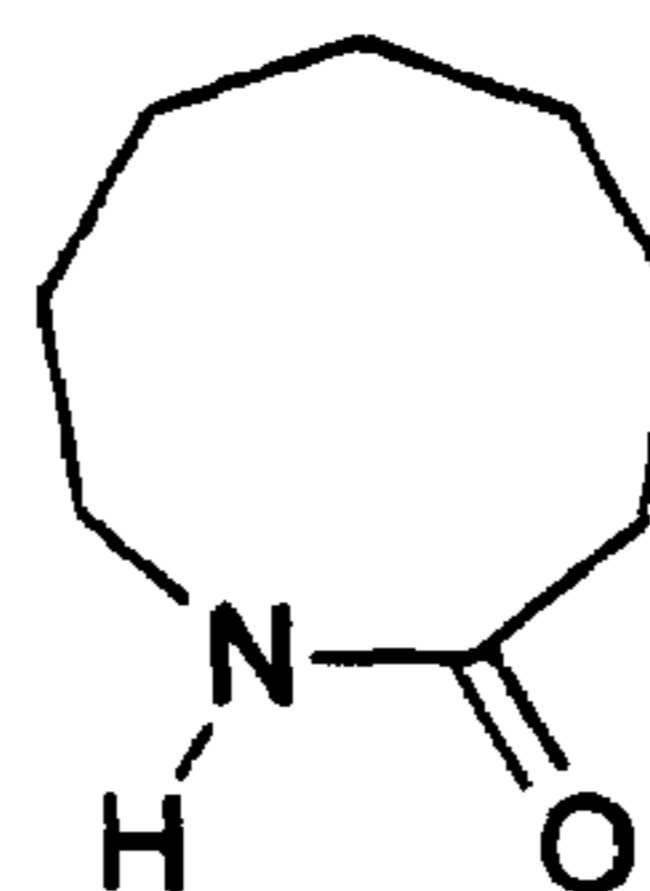
2-Azacyclononanone
